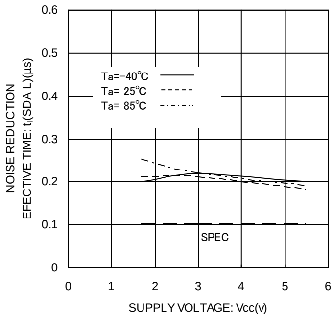
Figure 30. ノイズ除去有効時間 t_i(\text{SDA L})
