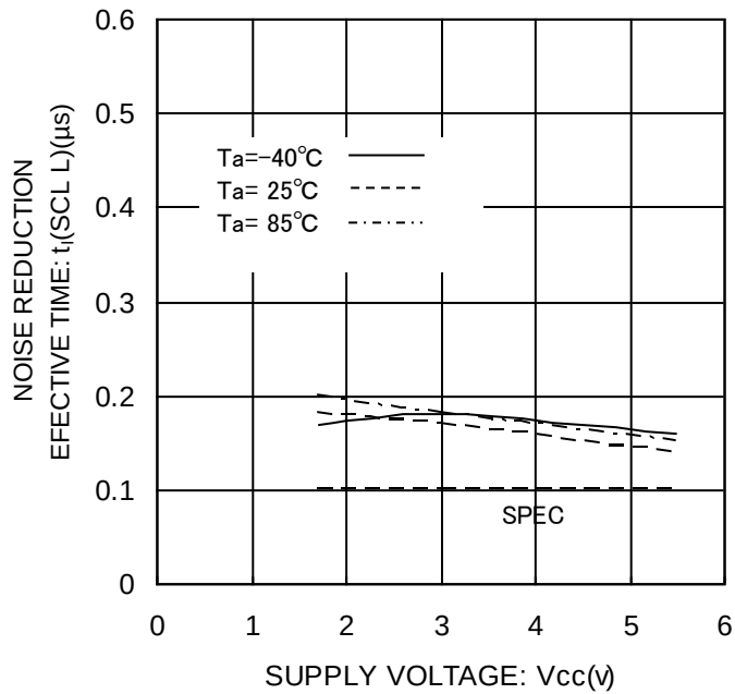
Figure 28. ノイズ除去有効時間 t_i(\text{SCL L})
