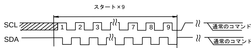
Figure 40.- (c) \text{START} \times 9 + \text{コマンド入力の場合}
