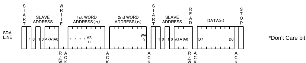
Figure 37. ランダムリードサイクル
