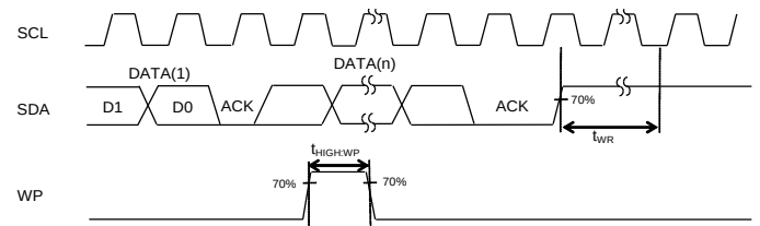
Figure 2-(e) ライトキャンセル時 WP タイミング
