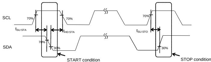
Figure 2-(b) スタート・ストップタイミング
