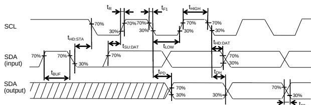
Figure 2-(a) 同期データ入出力タイミング
