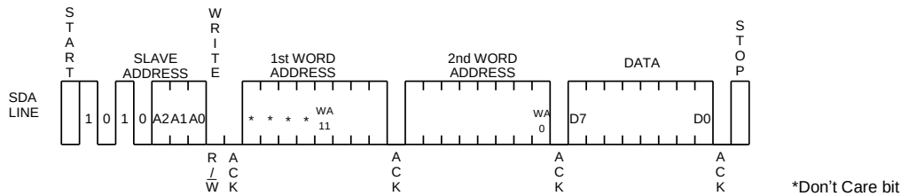
Figure 35. バイトライトサイクル
