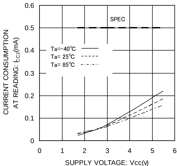
Figure 11. 動作時消費電流(リード) I_{cc2} ( f_{SCL}=400kHz )
