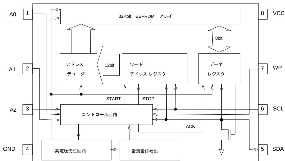
Figure 3. ブロック図
