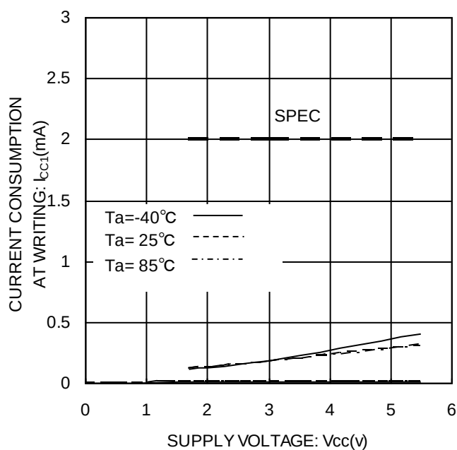
Figure 10. 動作時消費電流(ライト) I_{cc1} ( f_{SCL}=400kHz )
