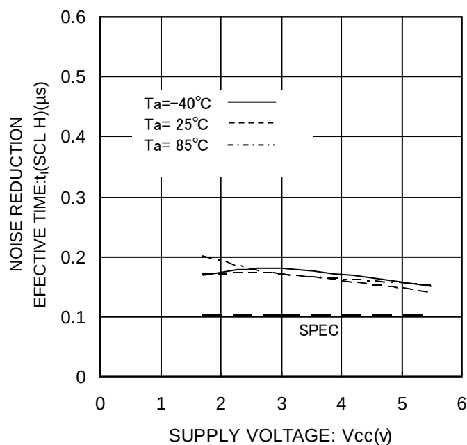
Figure 27. ノイズ除去有効時間 t_i (SCL H)
