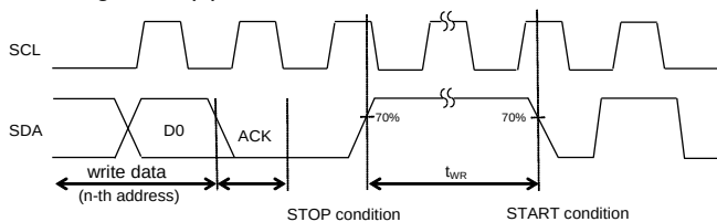
Fig.2-(c) 書き込みサイクルタイミング
