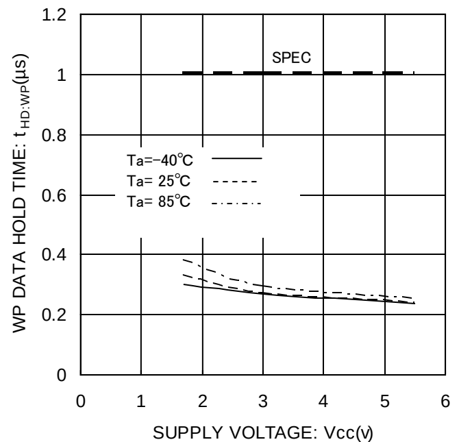
Figure 31. WP ホールド時間 t_{\text{DH:WP}}
