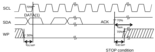
Figure 2-(d) ライト実行時 WP タイミング
