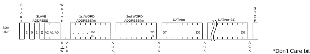
Figure 36. ページライトサイクル
