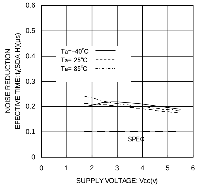
Figure 29. ノイズ除去有効時間 t_i(\text{SDA H})
