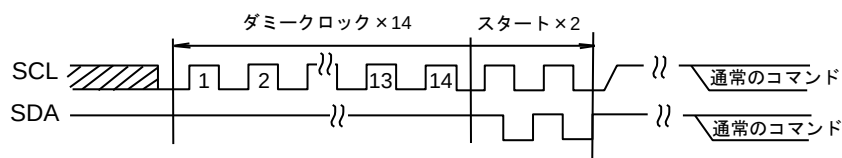
Figure 40.-(a) ダミークロック×14 + START + START + コマンド入力の場合
