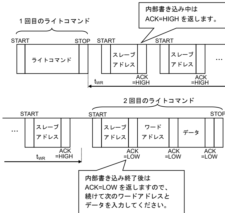
Figure 48. アクリッジポーリングで連続して書き込みを行う場合
