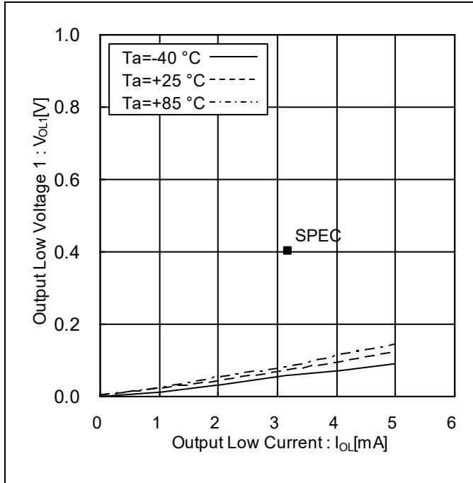
Figure 8. 'LOW'出力電圧 1 vs 'LOW'出力電流 (V CC =2.5 V)
