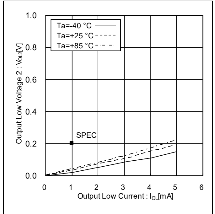
Figure 9. 'LOW'出力電圧 2 vs 'LOW'出力電流 (V CC =1.6 V)
