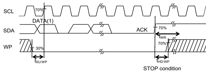
Figure 5-(d). ライト実行時 WP タイミング
