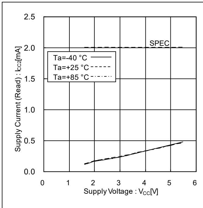
Figure 14. 消費電流(リード) vs 電源電圧 ( f_{SCL}=1 MHz)
