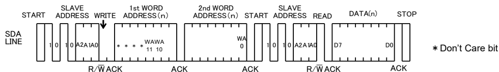
Figure 44. ランダムリード
