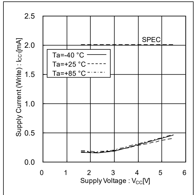
Figure 13. 消費電流(ライト) vs 電源電圧
