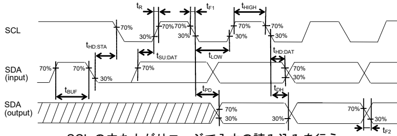
・SCL の立ち上がりエッジで入力の読み込みを行う。 ・SCL の立ち下がりエッジに同期してデータ出力を行う。 Figure 5-(a). 入出力タイミング
