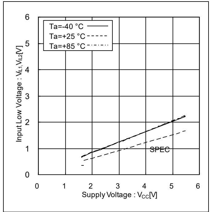
Figure 7. 'LOW'入力電圧 vs 電源電圧
