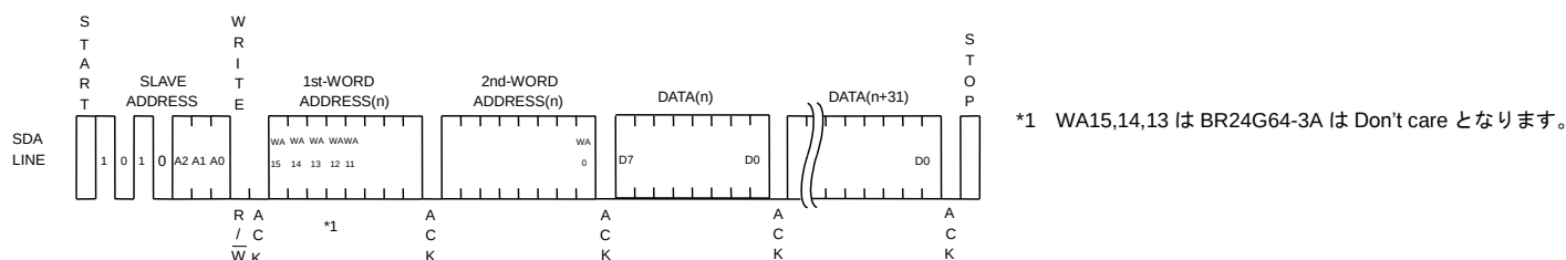
Figure 37. ページライトサイクル
