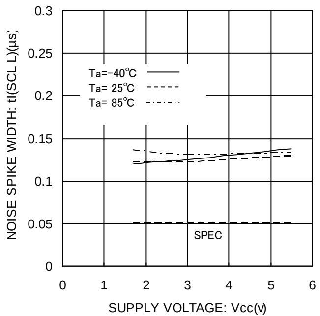
Figure 29. ノイズ除去有効時間 t_I(\text{SCL L})
