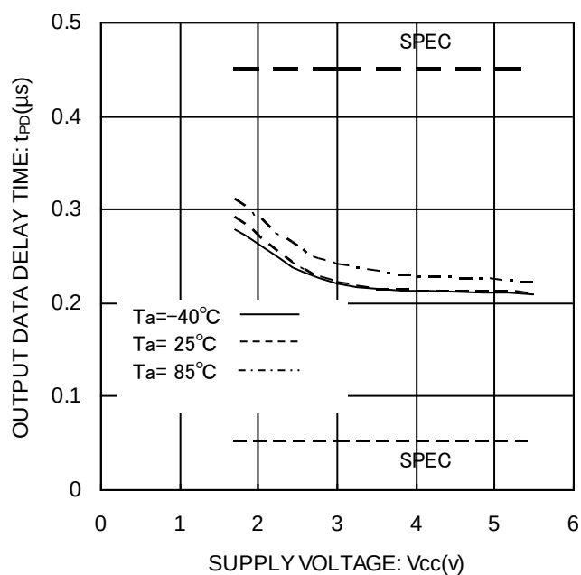
Figure 24. 出力データ遅延時間 t_{PD(HIGH)}
