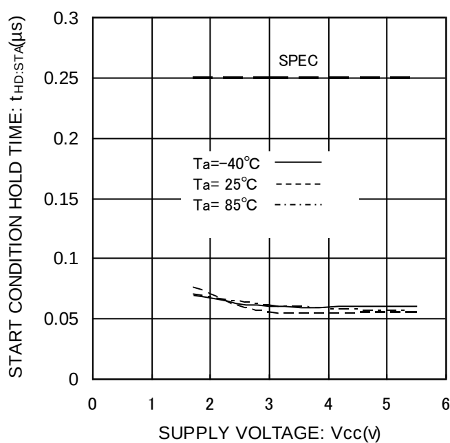
Figure 17. スタートコンディションホールド時間 t_{HD:STA}
