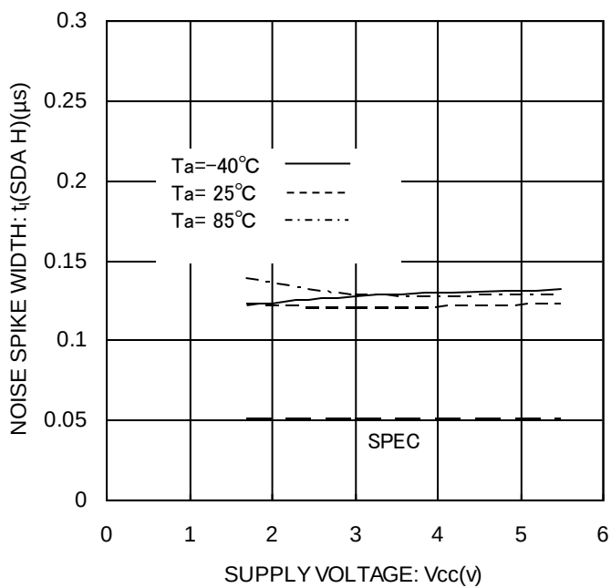
Figure 30. ノイズ除去有効時間 t_I(\text{SDA H})
