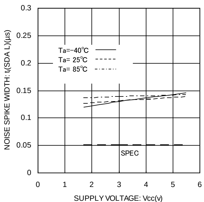
Figure 31. ノイズ除去有効時間 t_I(\text{SDA L})
