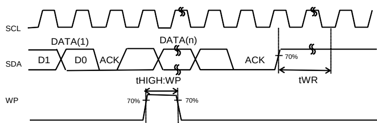
Figure 2-(e). ライトキャンセル時 WP タイミング
