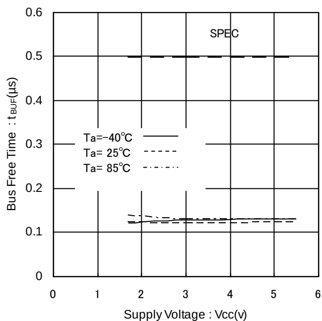
Figure 26. 転送開始前バス開放時間 t_{BUF}
