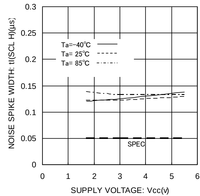
Figure 28. ノイズ除去有効時間 t_I(\text{SCL H})
