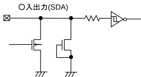
Figure 51. 入出力 pin 回路図
