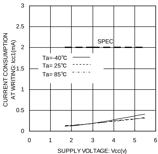
Figure 10. ライト動作時消費電流 I_{cc1} ( f_{SCL} = 1\text{MHz} )
