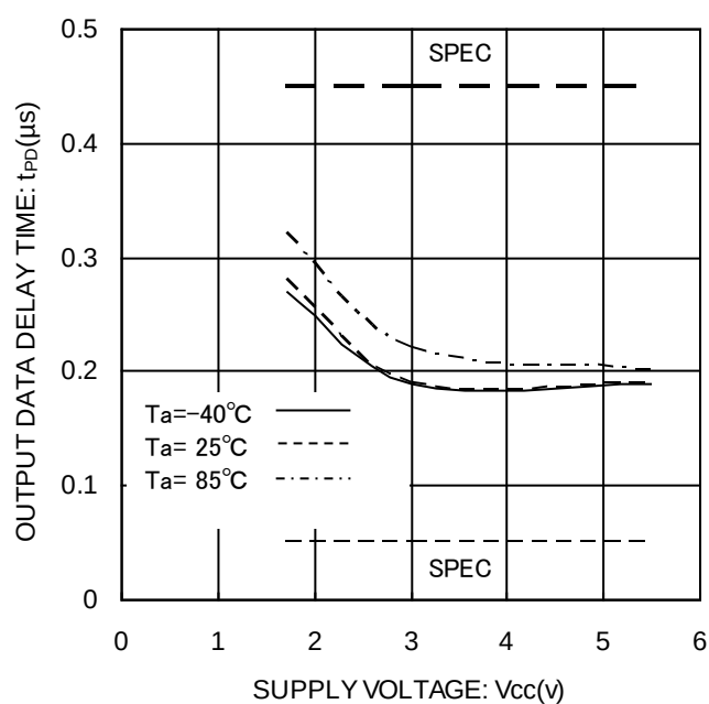
Figure 23. 出力データ遅延時間 t_{PD} (LOW)
