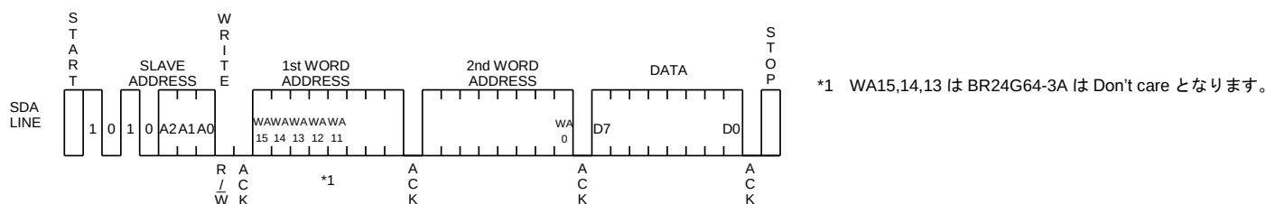
Figure 36. バイトライトサイクル
