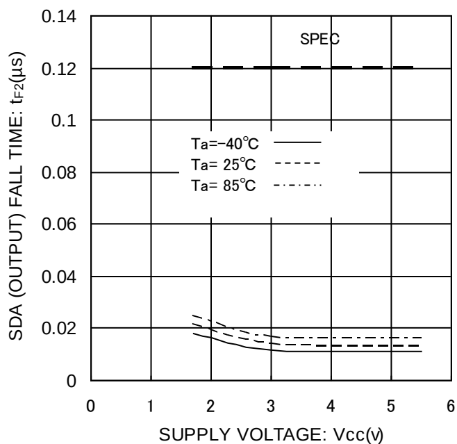
Figure 16. SDA の出力立ち下がり時間 t_{F2}
