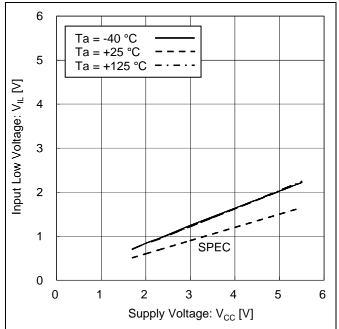
Figure 7. 'LOW'入力電圧 vs 電源電圧
