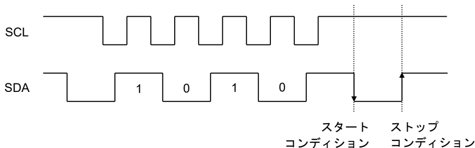
Figure 50. スレープアドレス入力中にスタート・ストップコンディションでキャンセルした場合
