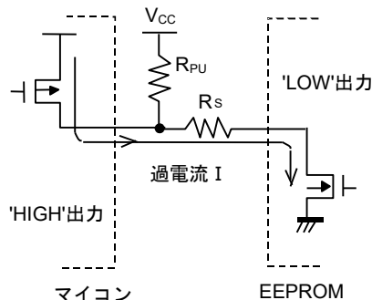
Figure 55. I/O 回路図
