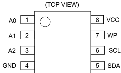
Figure 3. 端子配置図 (SOP8、SOP-J8、TSSOP-B8、MSOP8)
