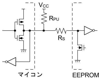
Figure 52. I/O 回路図
