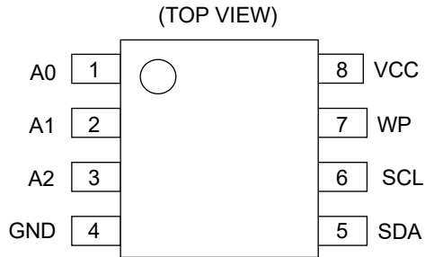
Figure 3. 端子配置図 (SOP8*1、SOP-J8、TSSOP-B8、MSOP8)
