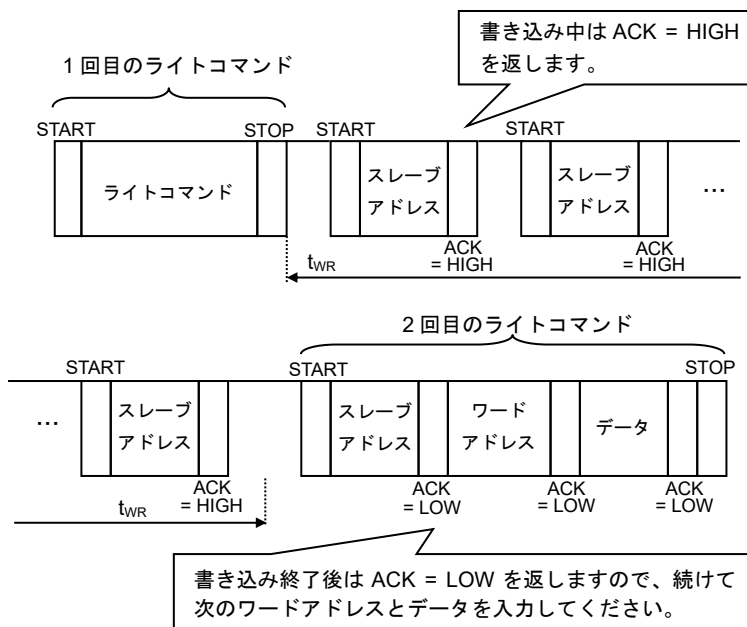
Figure 48. アクリッジポーリングで連続して書き込みを行う場合
