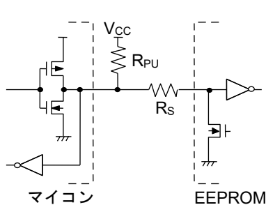
Figure 52. I/O 回路図
