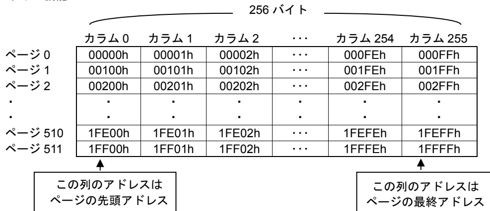
Figure 44. ページライト機能における 256 バイトのページとメモリアレイのアドレスの関係
