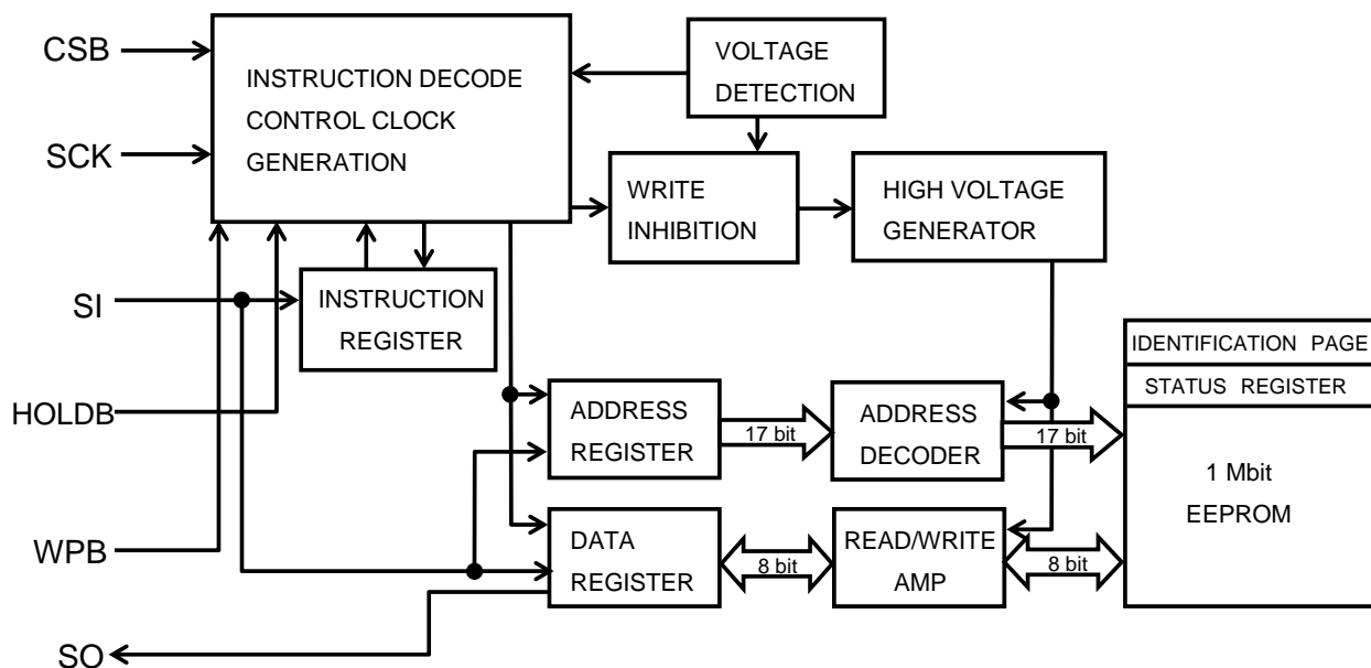
Figure 4. ブロック図
