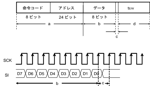
Figure 54. WRITE, WRID, LID キャンセル有効タイミング
