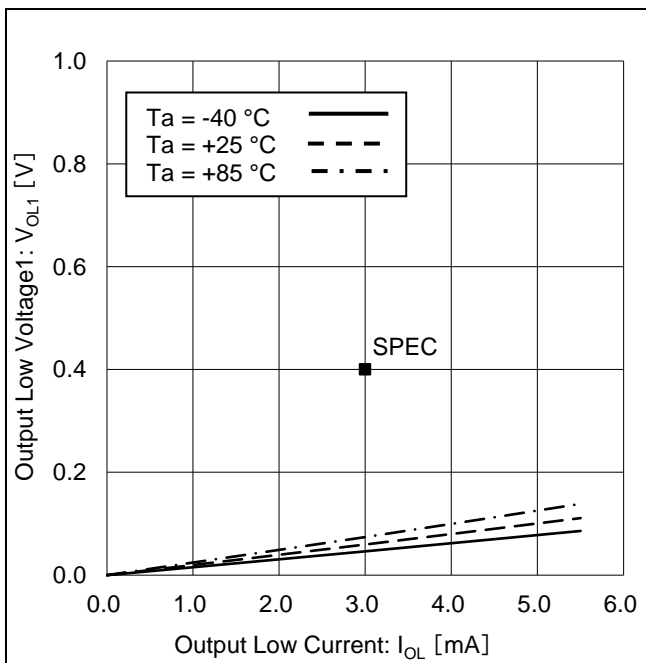
Figure 9. 'LOW'出力電圧1 vs 'LOW'出力電流 ( V_{CC} = 2.5\text{ V} )
