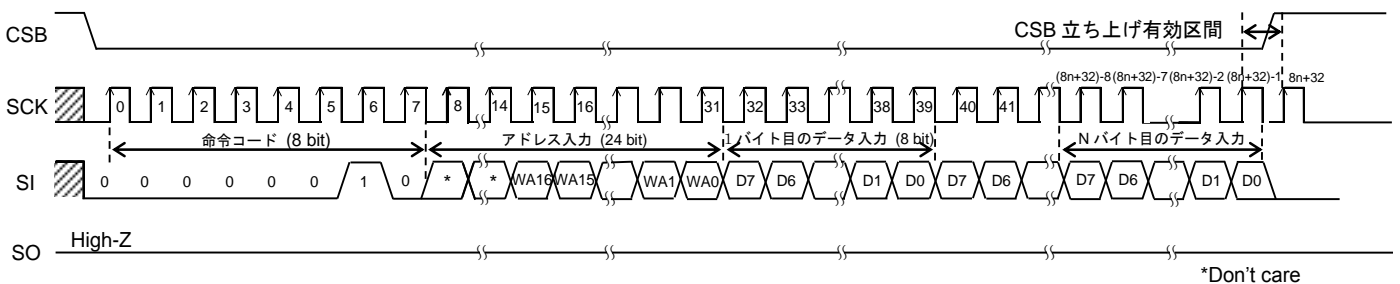
Figure 43. 書き込み命令 (ページライト)
