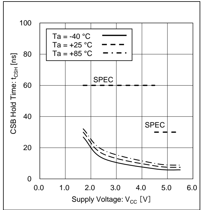
Figure 24. CSB ホールド時間 vs 電源電圧
