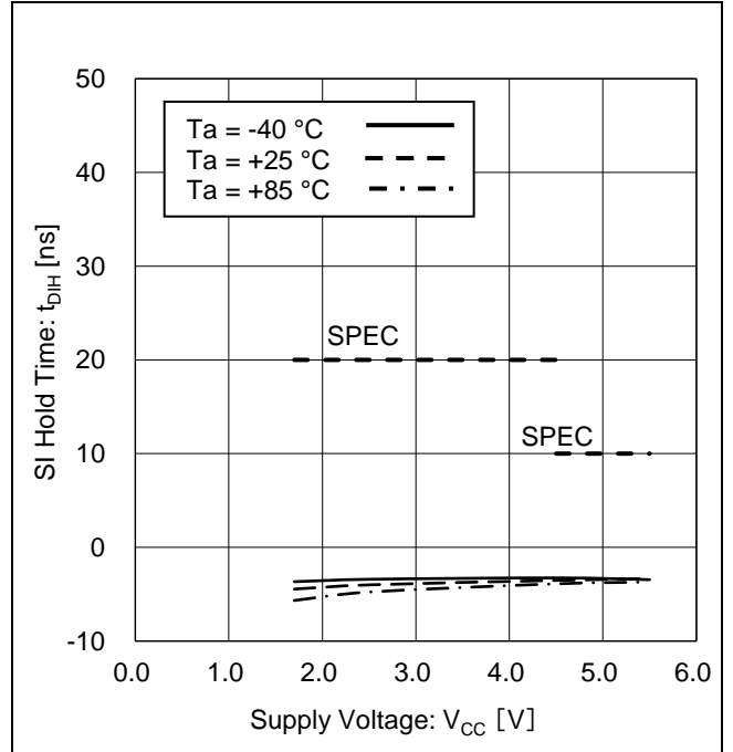
Figure 26. SI ホールド時間 vs 電源電圧
