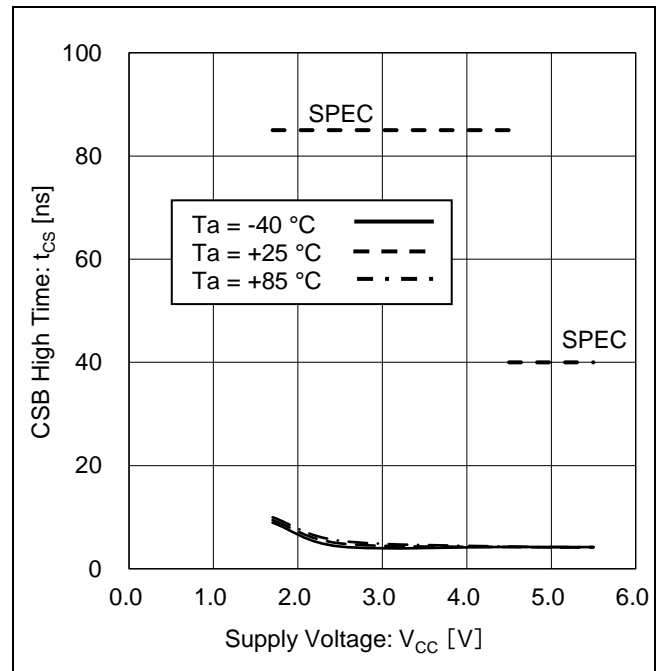
Figure 22. CSB ハイ時間 vs 電源電圧
