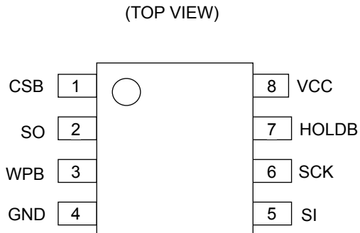
Figure 3. 端子配置図
