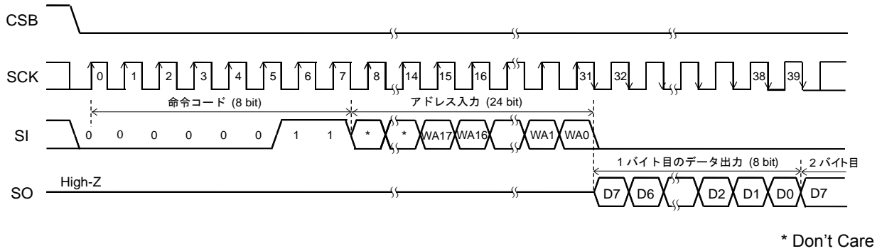
Figure 40. 読み出し命令
