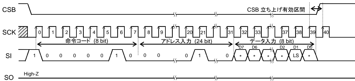
Figure 49. ID ページロック命令
