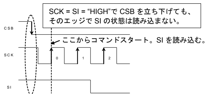
Figure 50. 動作タイミング
