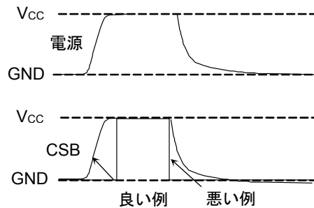
Figure 62. 電源 ON/OFF 時の CSB タイミング
