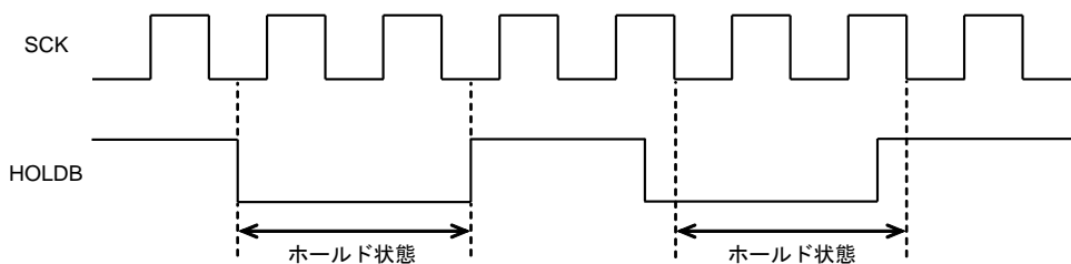
Figure 37. ホールド状態
