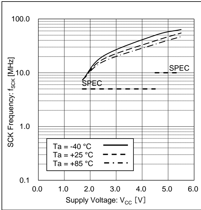
Figure 19. SCK 周波数 vs 電源電圧
