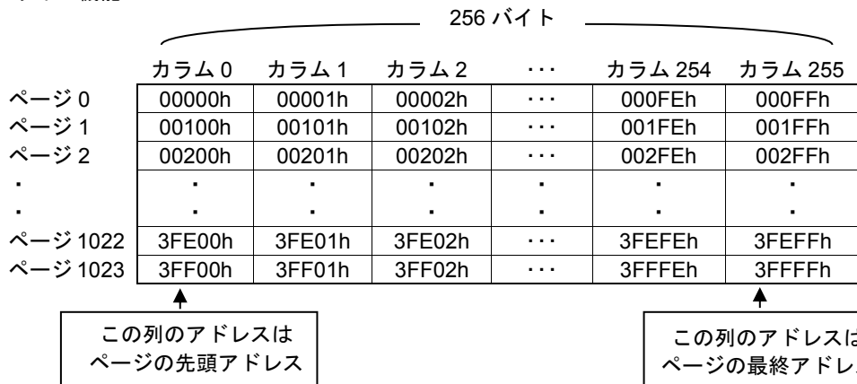
Figure 43. ページライト機能における 256 バイトのページとメモリアレイのアドレスの関係
