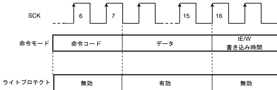
Figure 36. ライトプロテクト有効タイミング (WRSR)
