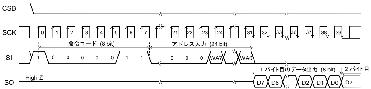
Figure 46. ID ページ読み出し命令
