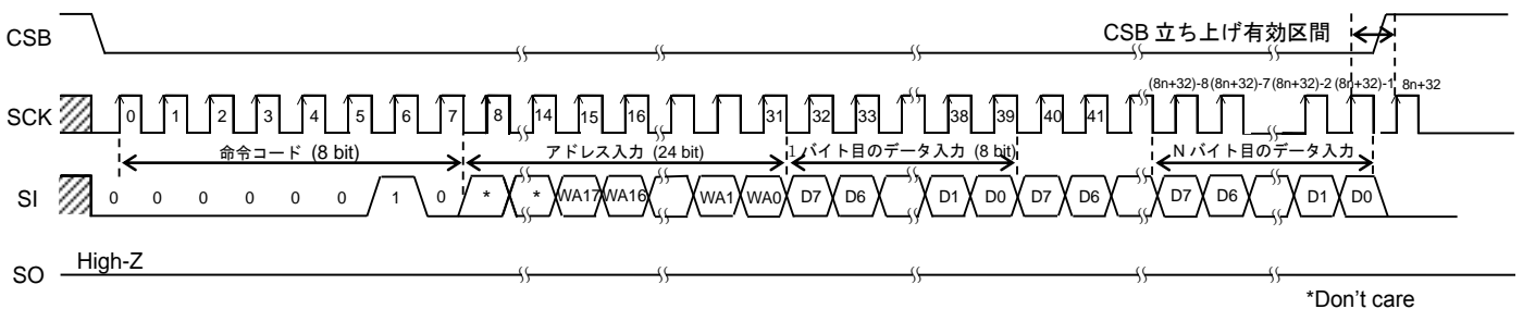
Figure 42. 書き込み命令 (ページライト)
