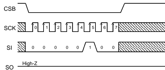
Figure 39. 書き込み禁止命令
