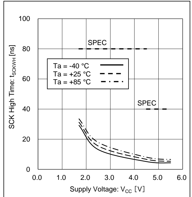
Figure 20. SCK ハイ時間 vs 電源電圧
