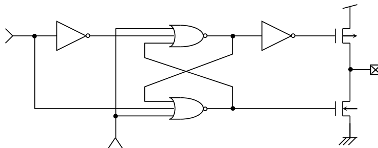
Figure 60. 出力端子回路図 (SO)
