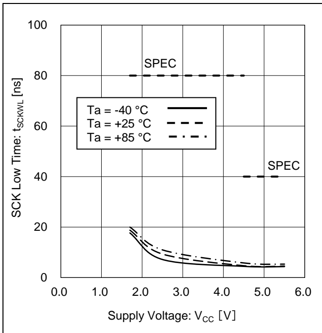
Figure 21. SCK ロウ時間 vs 電源電圧
