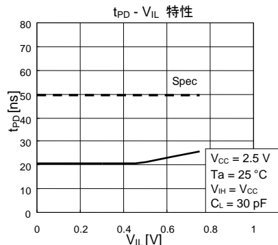
Figure 58. データ出力遅延時間 t_{PD} の V_{IL} 依存性
