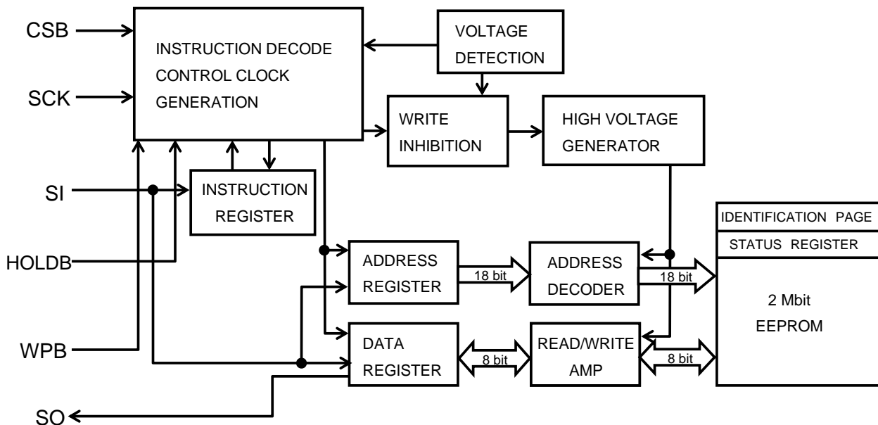
Figure 4. ブロック図
