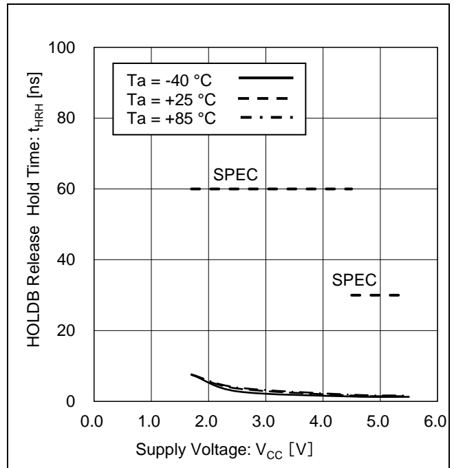
Figure 30. HOLDB 解除ホールド時間 vs 電源電圧
