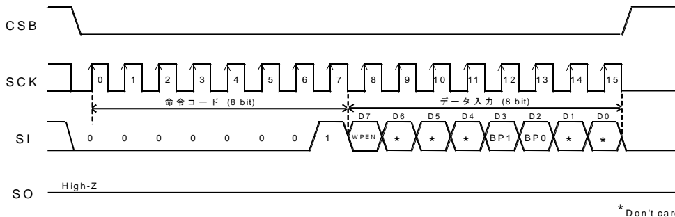
Figure 45. ステータスレジスタ書き込み命令
