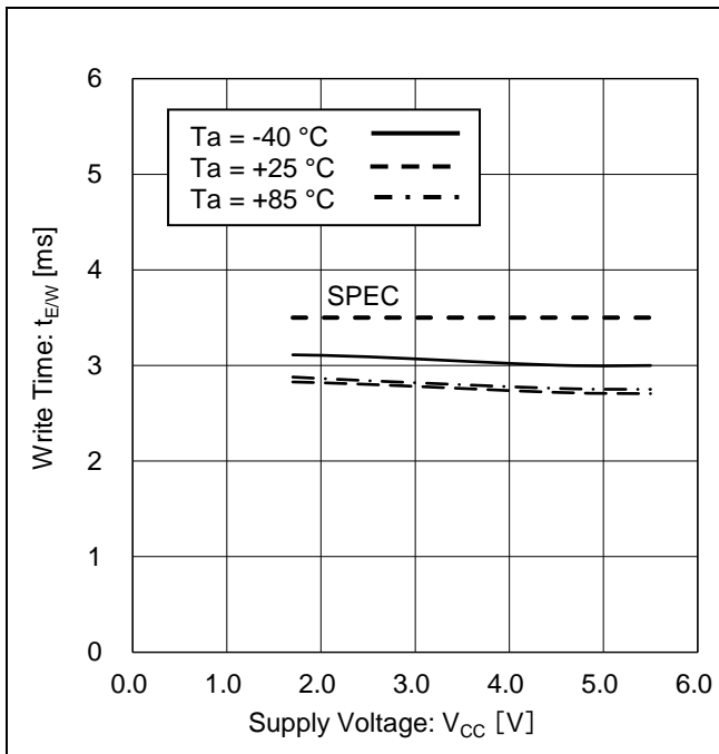
Figure 35. 書き込み時間 vs 電源電圧
