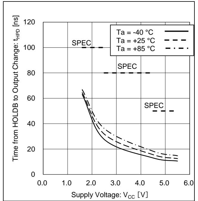
Figure 32. HOLDB より出力変化までの時間 vs 電源電圧
