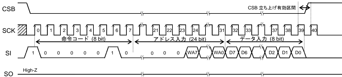
Figure 47. ID ページ書き込み命令
