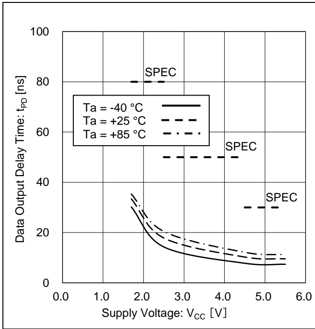
Figure 27. データ出力遅延時間 vs 電源電圧
