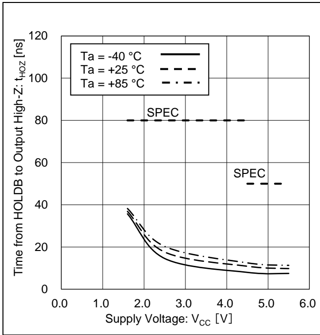
Figure 31. HOLDB より出力 High-Z までの時間 vs 電源電圧
