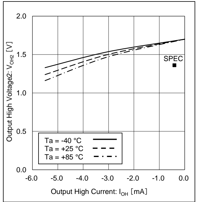
Figure 12. 'HIGH'出力電圧 2 vs 'HIGH'出力電流 ( V_{CC} = 1.7\text{ V} )
