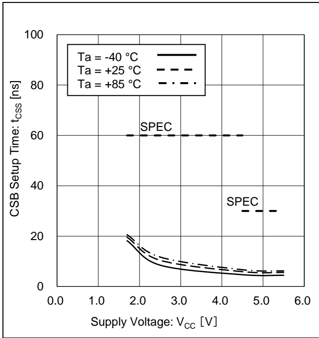
Figure 23. CSB セットアップ時間 vs 電源電圧
