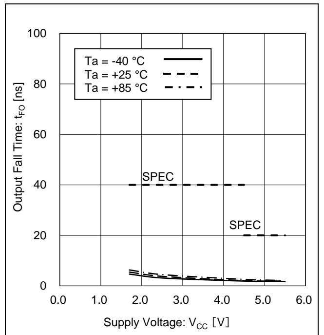
Figure 34. 出力立ち下がり時間 vs 電源電圧
