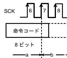
Figure 55. WREN/WRDI キャンセル有効タイミング
