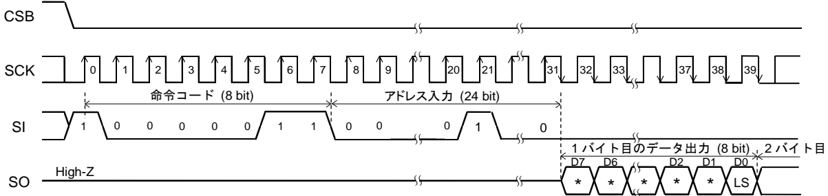
Figure 48. ロックステータス読み出し命令
