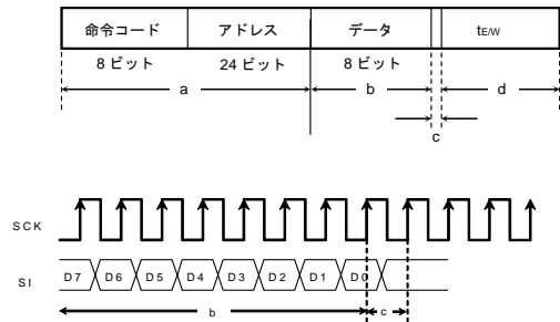
Figure 53. WRITE, WRID, LID キャンセル有効タイミング
