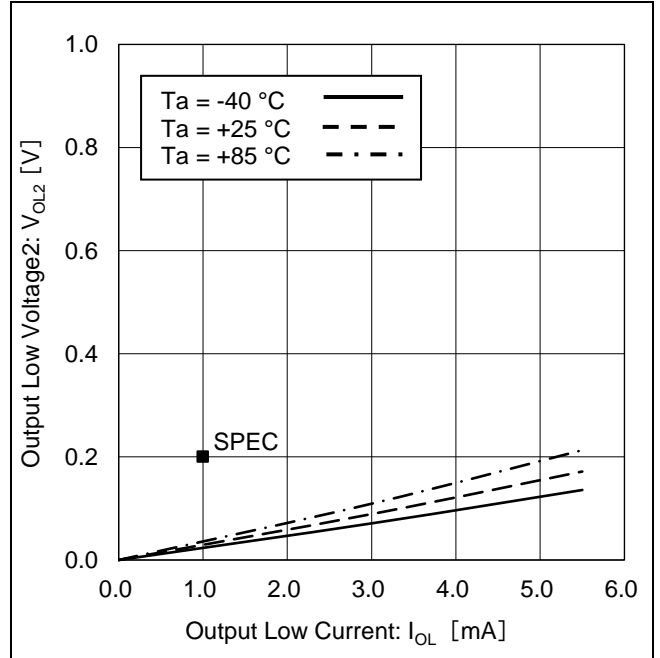
Figure 10. 'LOW'出力電圧 2 vs 'LOW'出力電流 ( V_{CC} = 1.7 \text{ V} )
