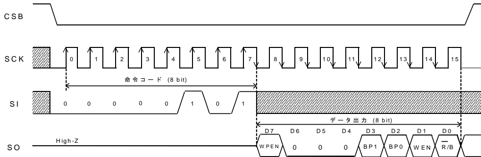
Figure 44. ステータスレジスタ読み出し命令
