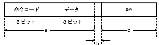
Figure 54. WRSR キャンセル有効タイミング
