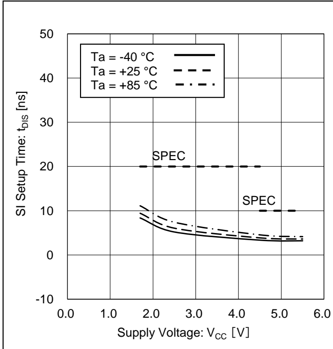
Figure 25. SI セットアップ時間 vs 電源電圧
