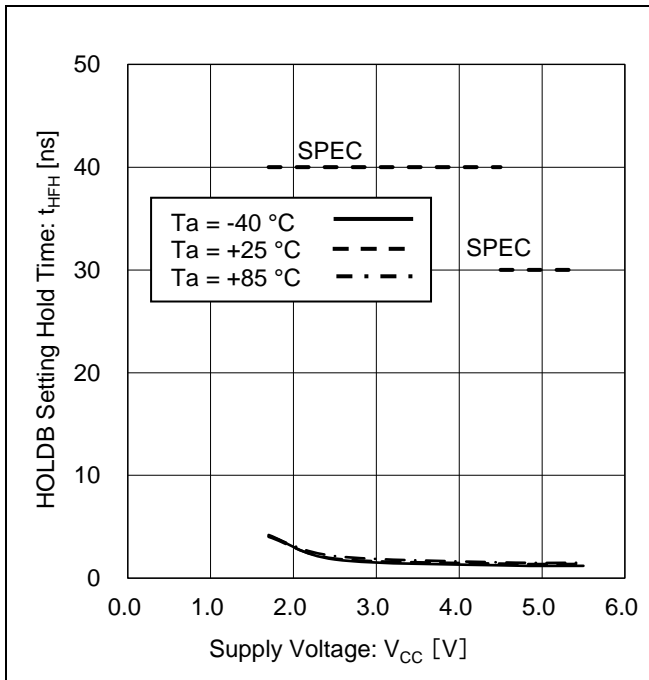
Figure 29. HOLDB 設定ホールド時間 vs 電源電圧
