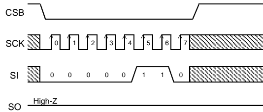
Figure 38. 書き込み許可命令
