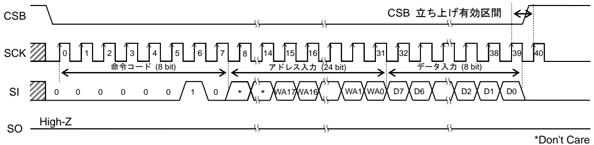
Figure 41. 書き込み命令 (バイトライト)
