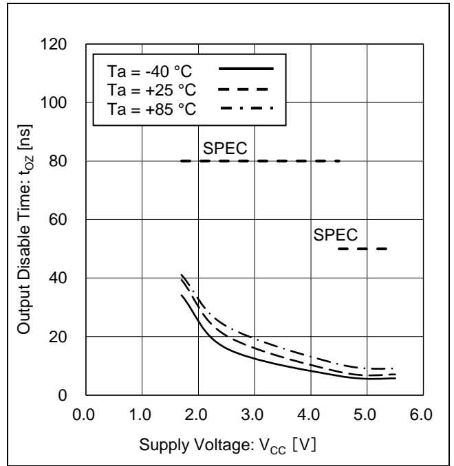
Figure 28. 出力ディセーブル時間 vs 電源電圧
