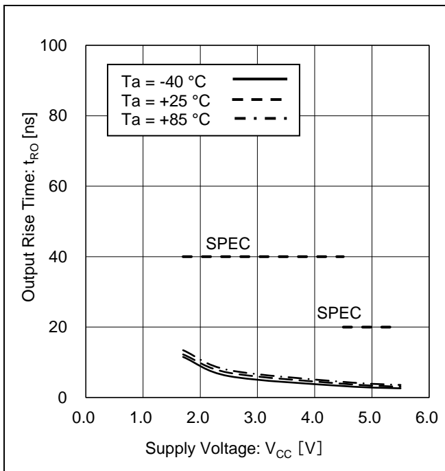
Figure 33. 出力立ち上がり時間 vs 電源電圧
