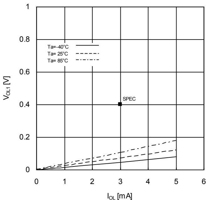
Figure 7. "L" 出力電圧 1 vs 出力電流 (V CC =2.5V)
