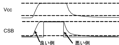
Figure 58. 電源 ON/OFF 時の CSB タイミング
