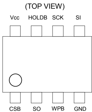
Figure 4. 端子配置図
