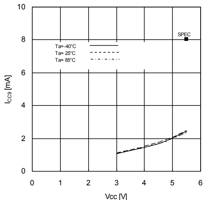
Figure 18. 動作時消費電流リード vs 電源電圧 ( f_{SCK} = 20\text{MHz} )
