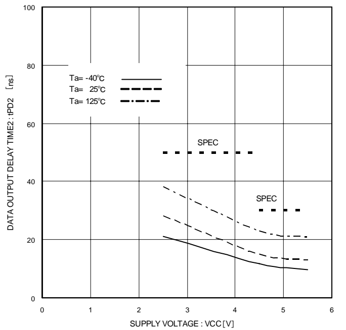
Figure 26. データ出力遅延時間 tPD2 (CL=30pF)
