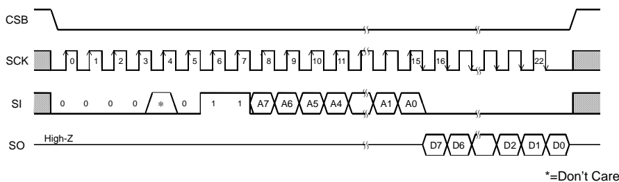
Figure 37. 読み出し命令
