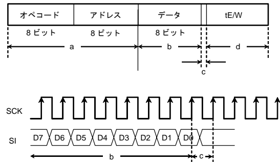
Figure 48. WRITE キャンセル有効タイミング
