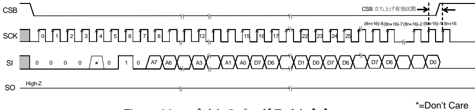
Figure 39. n バイトのページライト命令
