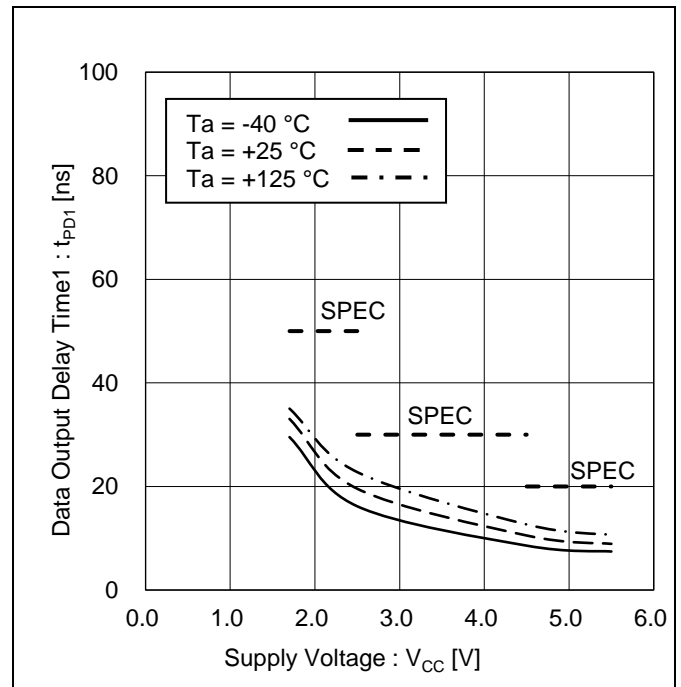
Figure 28. データ出力遅延時間 1 vs 電源電圧
