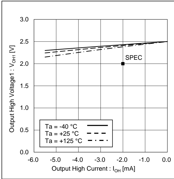
Figure 11. 'HIGH'出力電圧 1 vs 'HIGH'出力電流 (V CC = 2.5 V)
