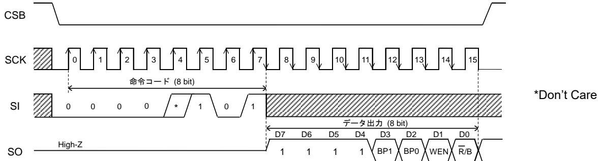
Figure 46. ステータスレジスタ読み出し命令
