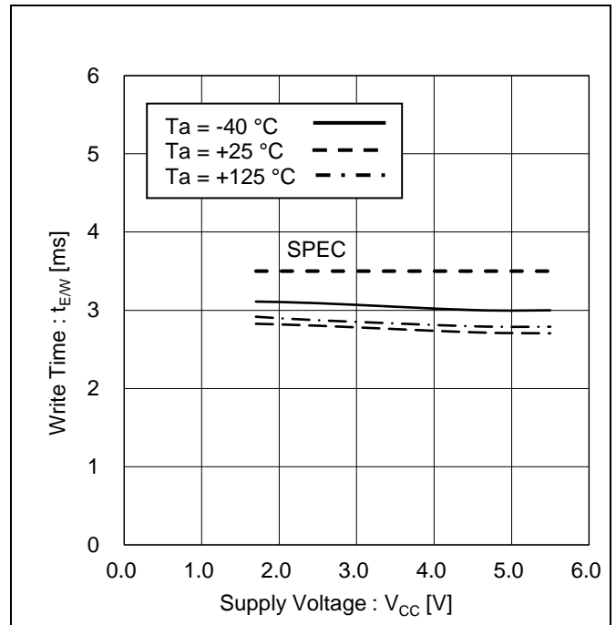
Figure 36. 書き込み時間 vs 電源電圧
