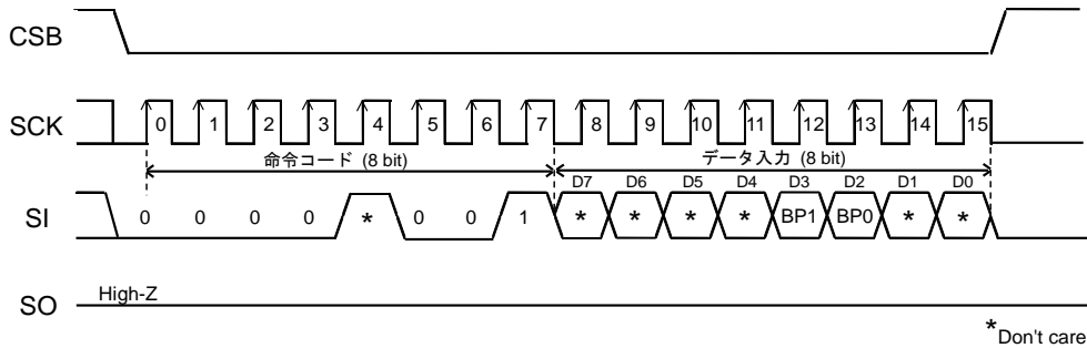
Figure 47. ステータスレジスタ書き込み命令
