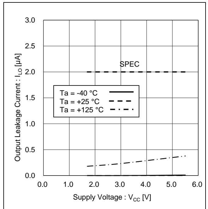
Figure 14. 出力リーク電流 vs 電源電圧 (SO)
