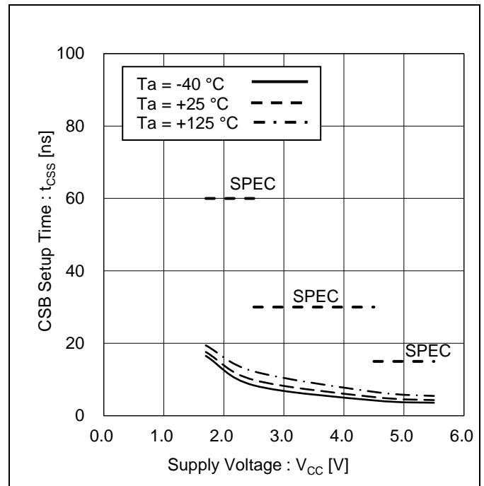
Figure 24. CSB セットアップ時間 vs 電源電圧
