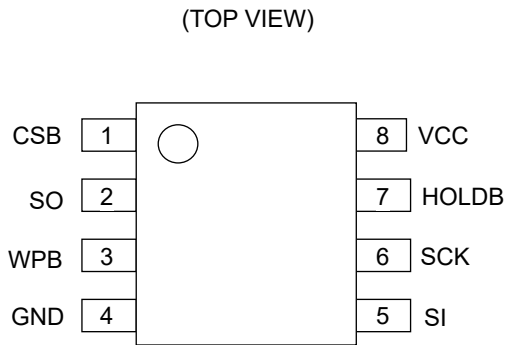
Figure 3-(a). 端子配置図 (SOP8、SOP-J8、TSSOP-B8、MSOP8)
