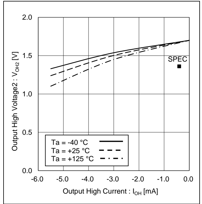
Figure 12. 'HIGH'出力電圧 2 vs 'HIGH'出力電流 (V CC = 1.7 V)
