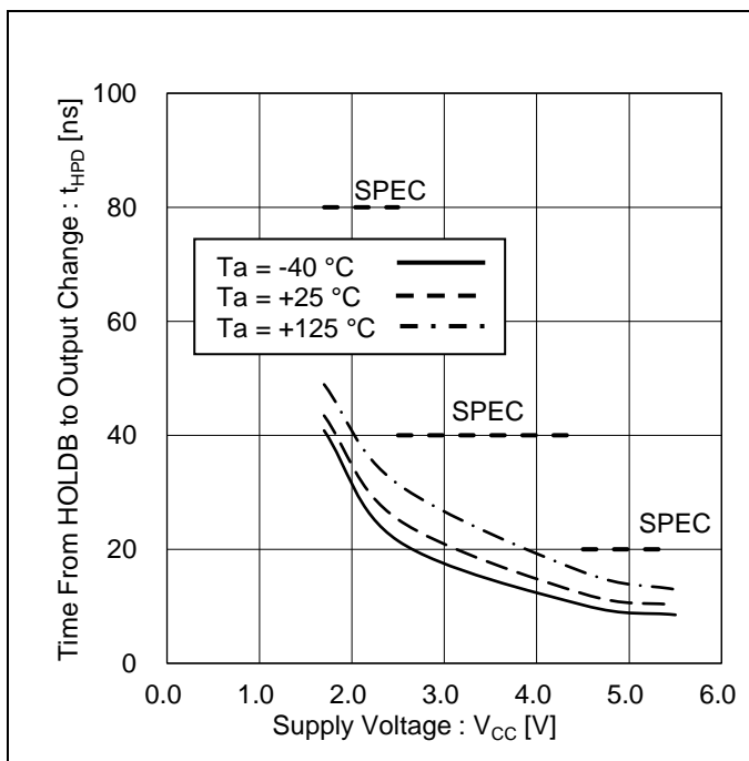
Figure 33. HOLDより出力変化までの時間 vs 電源電圧
