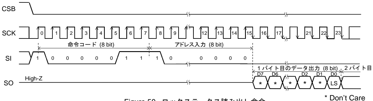
Figure 50. ロックステータス読み出し命令
