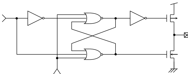
Figure 62. 出力端子回路図 (SO)
