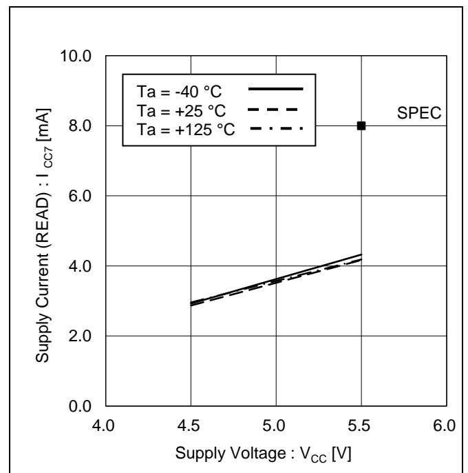
Figure 18. 消費電流 (リード) vs 電源電圧
