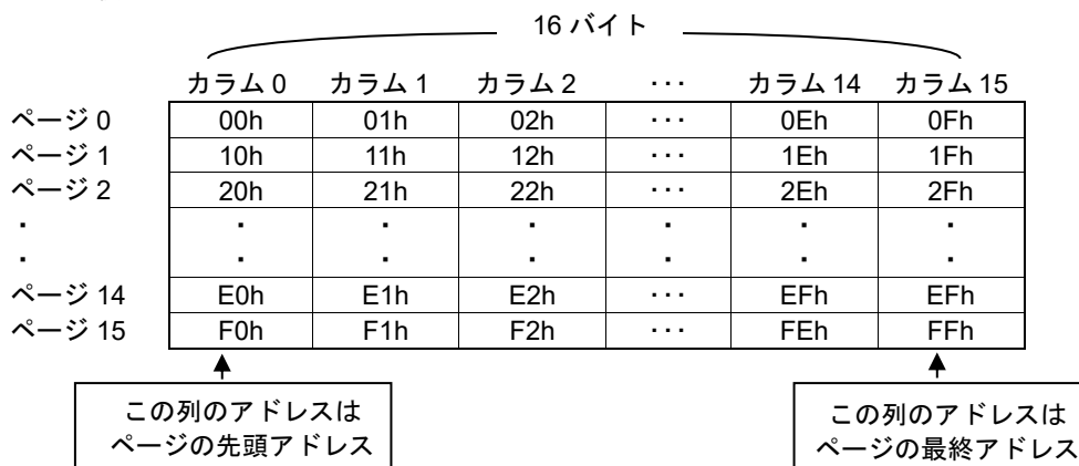
Figure 45. ページライト機能における 16 バイトのページとメモリアレイのアドレスの関係
