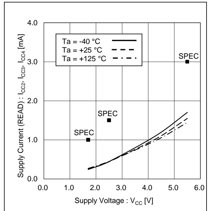
Figure 16. 消費電流 (リード) vs 電源電圧
