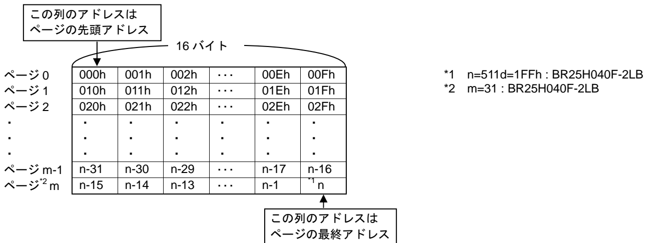
Figure 40. ページライト機能における 16 バイトのページと EEPROM のアドレスの関係
