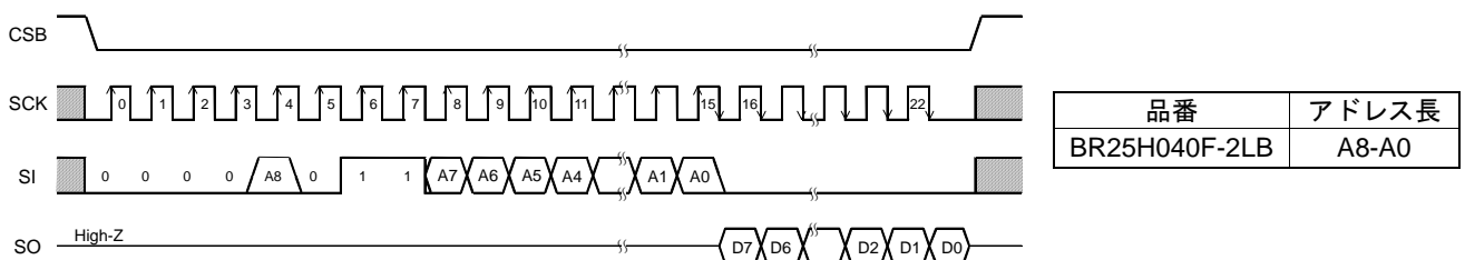
Figure 37. 読み出し命令
