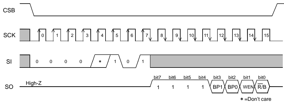
Figure 42. ステータスレジスタ読み出し命令
