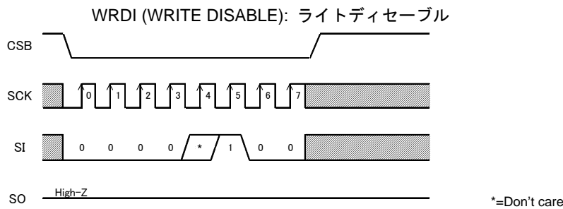
Figure 36. 書き込み禁止
