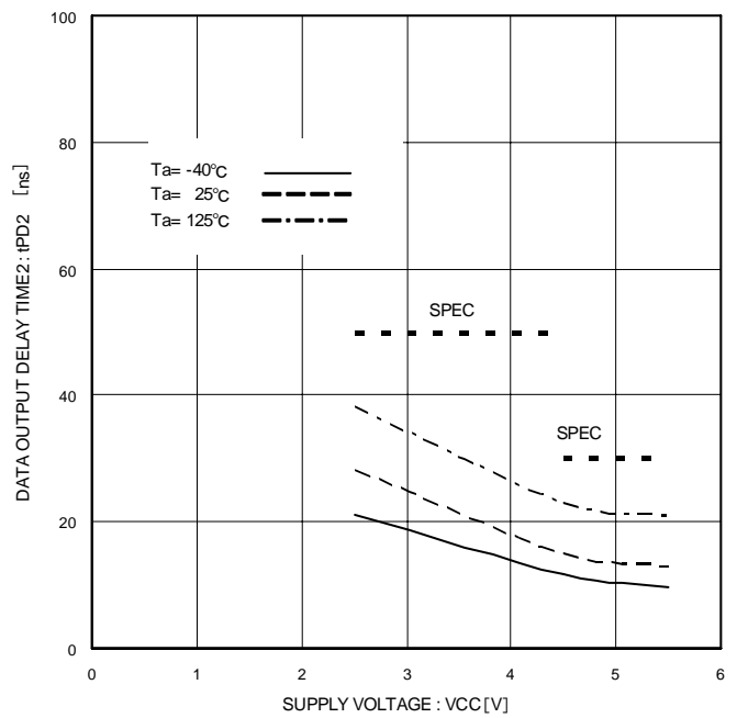
Figure 26. データ出力遅延時間 t_{PD2} ( C_L=30\text{pF} )
