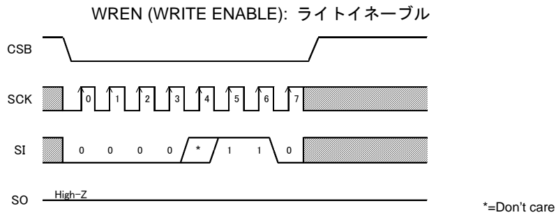
Figure 35. 書き込み可能命令
