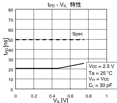
Figure 60. データ出力遅延時間 t_{PD} の V_{IL} 依存性
