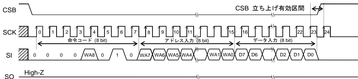
Figure 43. 書き込み命令 (バイトライト)
