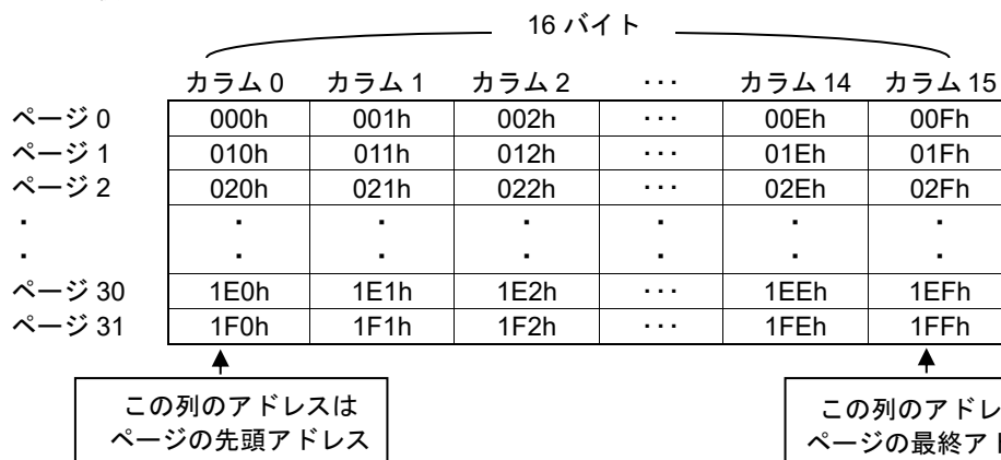
Figure 45. ページライト機能における 16 バイトのページとメモリアレイのアドレスの関係
