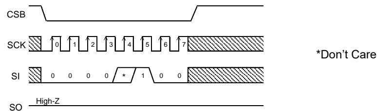
Figure 41. 書き込み禁止命令
