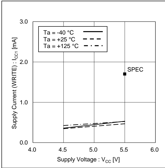
Figure 15. 消費電流 (ライト) vs 電源電圧
