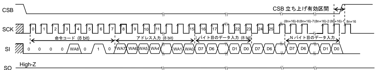
Figure 44. 書き込み命令 (ページライト)
