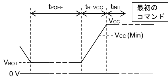
Figure 63. 電源立ち上げ波形図
