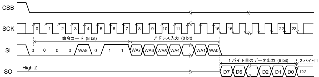
Figure 42. 読み出し命令
