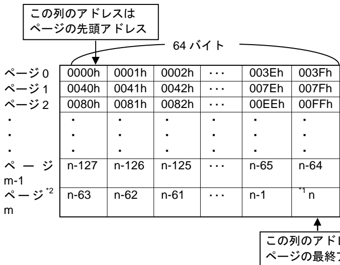
Figure 40. ページライト機能における 64 バイトのページと EEPROM のアドレスの関係
