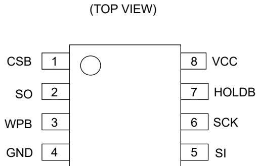
Figure 3. 端子配置図 (SOP8、SOP-J8、TSSOP-B8)
