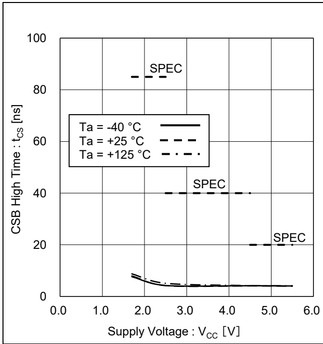
Figure 23. CSB ハイ時間 vs 電源電圧
