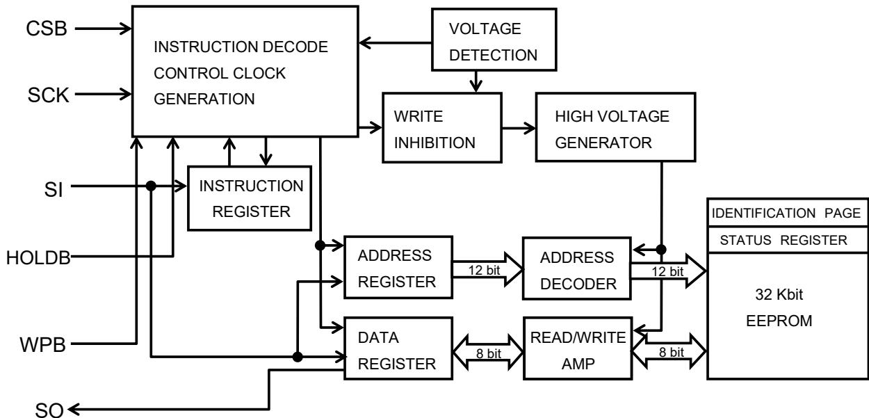
Figure 4. ブロック図
