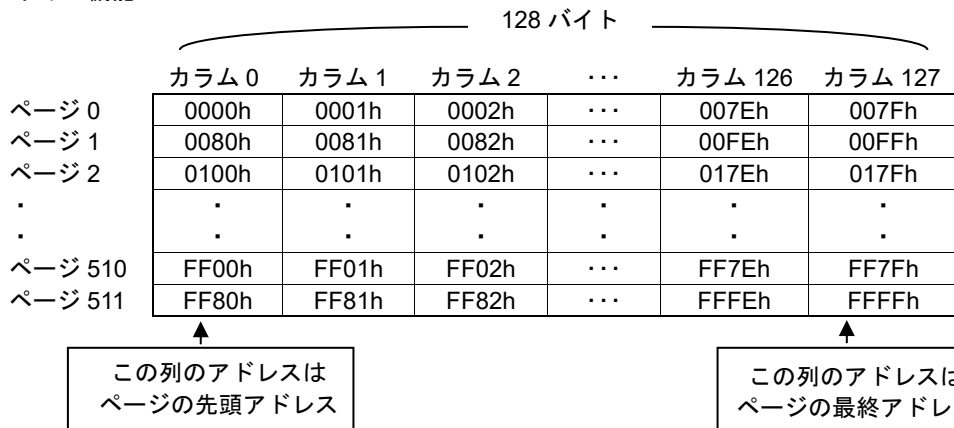
Figure 44. ページライト機能における 128 バイトのページとメモリアレイのアドレスの関係
