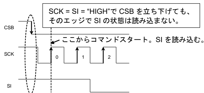
Figure 51. 動作タイミング
