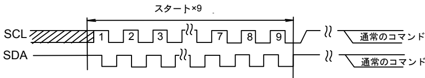
Figure 39-(c). START×9+コマンド入力の場合
