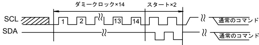
Figure 39-(a). ダミークロック×14+START+START+コマンド入力の場合
