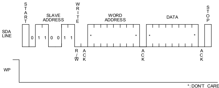
Figure 38. クリアライトプロテクトサイクル
