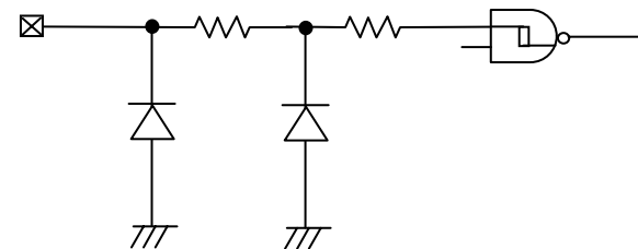
Figure 50. 入力 pin 回路図
