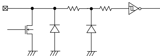
Figure 49. 入力 pin 回路図
