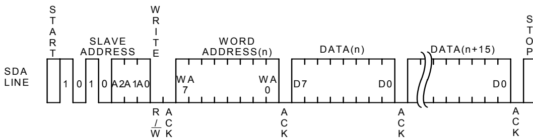
Figure 32. ページライトサイクル
