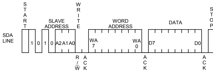
Figure 31. バイトライトサイクル
