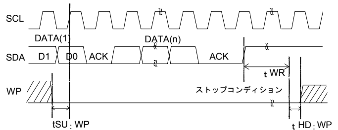
Figure 1(d). ライト実行時 WP タイミング
