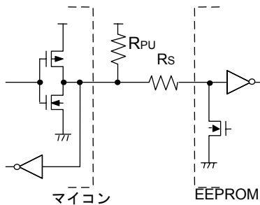
Figure 44. I/O 回路図
