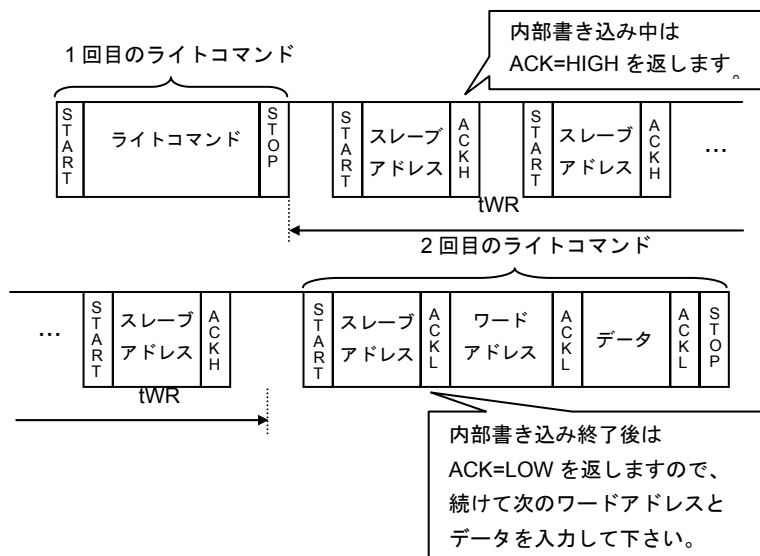
Figure 40. アクノリッジポーリングで連続しめを行う場合
