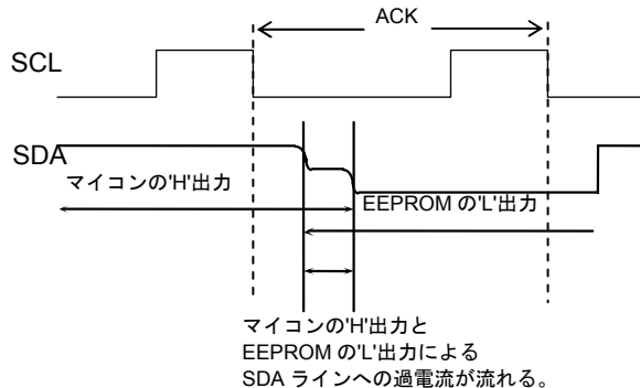
Figure 45. 入出力衝突タイミング
