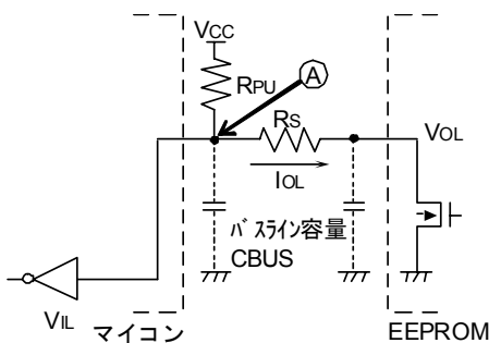
Figure 46. I/O 回路図
