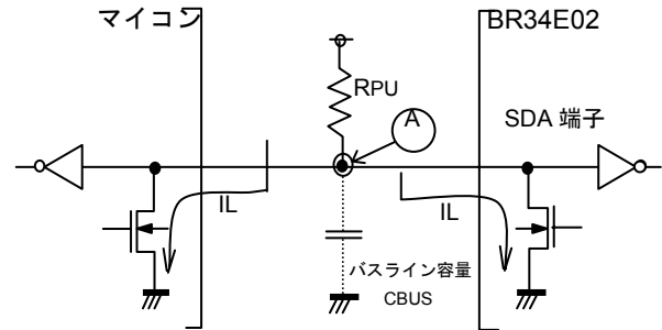
Figure 43. I/O 回路図
