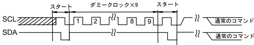
Figure 39-(b). START+ダミークロック×9+START+コマンド入力の場合
