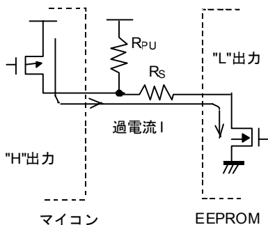
Figure 47. I/O 回路図
