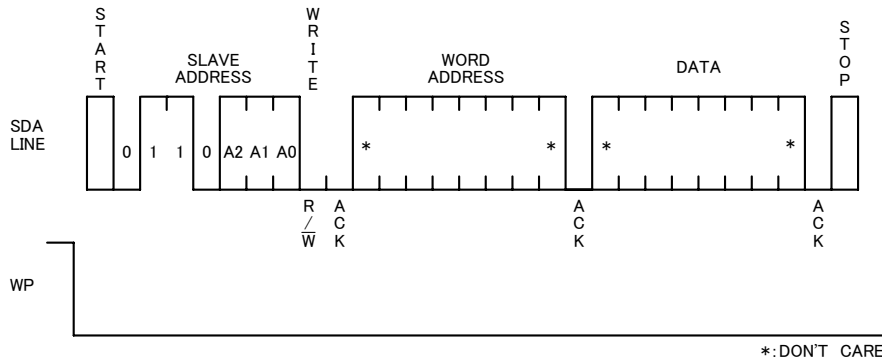
Figure 36. パーマネントセットライトプロテクトサイクル
