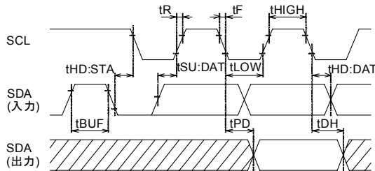
Figure 1(a). 同期データ入出力タイミング
