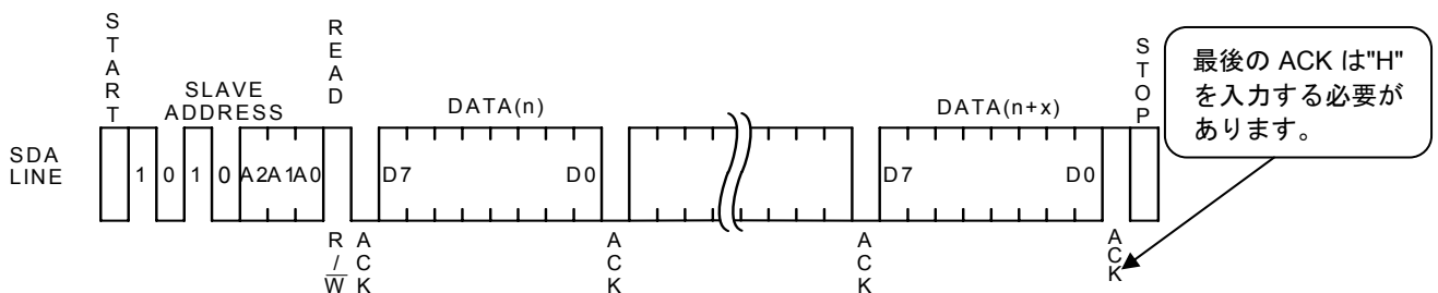
Figure 35. シーケンシャルリードサイクル(カレントリードサイクルの場合)
