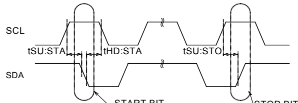
Figure 1(b). スタート・ストップビットタイミング
