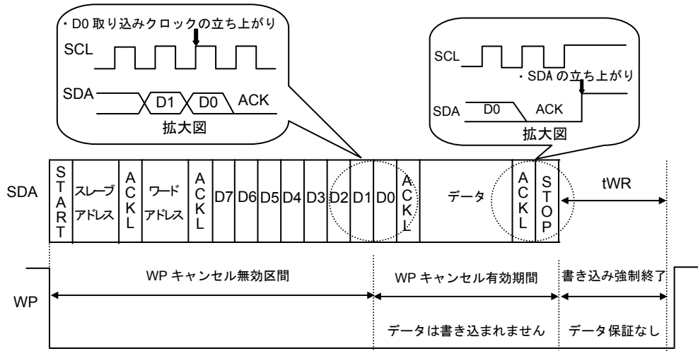
Figure 41. WP 有効タイミング
