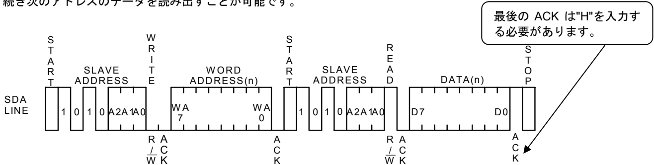
Figure 33. ランダムリードサイクル
