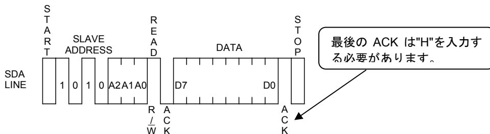
Figure 34. カレントリードサイクル
