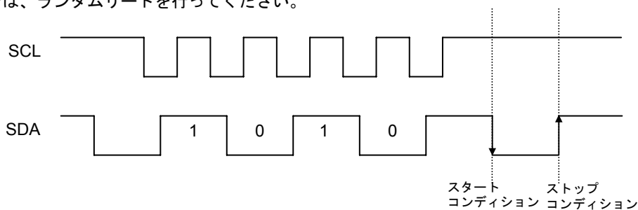
Figure 42. スレーブアドレス入力中にスタート・ストップコンディションでキャンセルした場合
