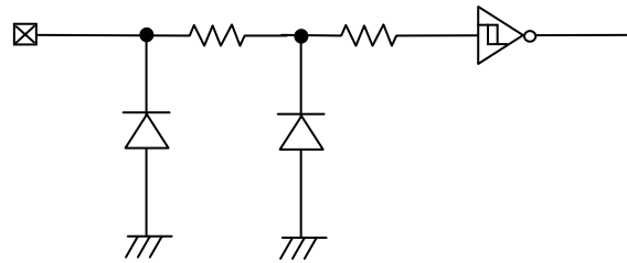
Figure 48. 入力 pin 回路図
