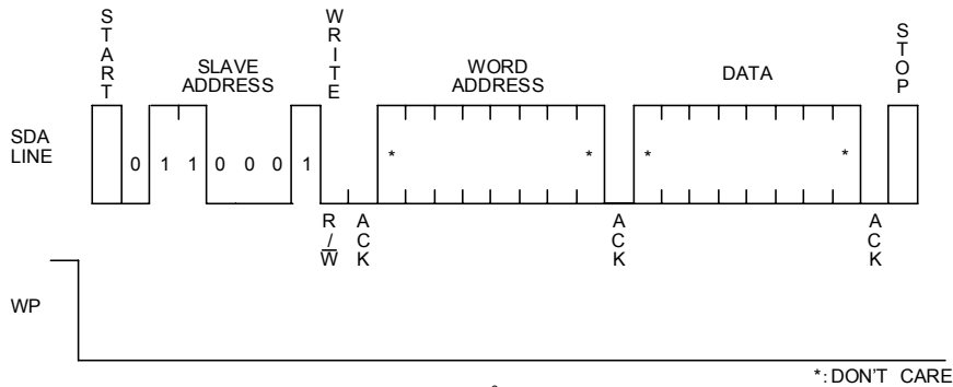
Figure 37. セットライトプロテクトサイクル
