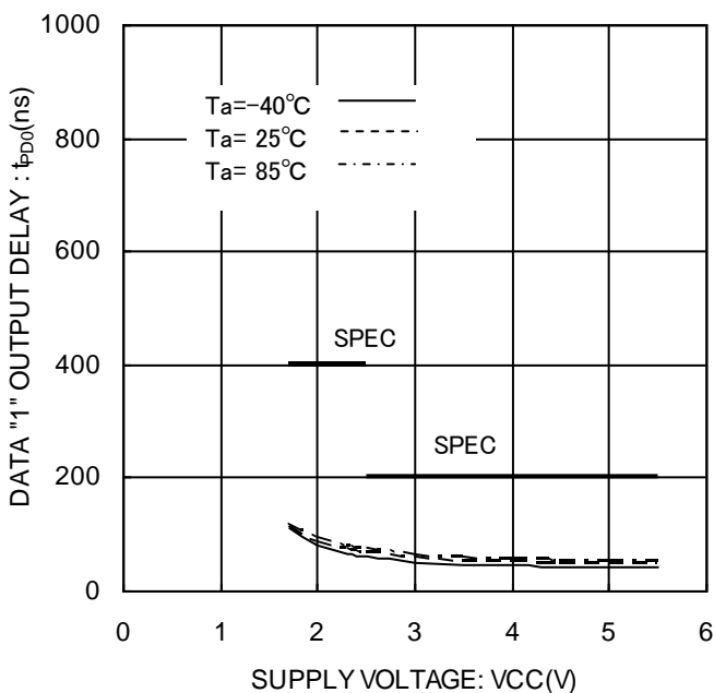
Figure 30. データ"1" 出力遅延時間 t_{PO1}
