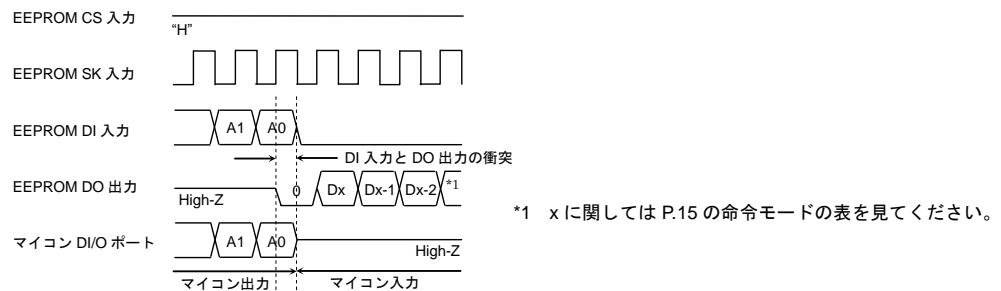
Figure 50. DI, DO 直結時リードデータ出力時の衝突タイミング
