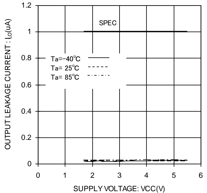
Figure 13. 出力リーク電流 I_{LO}(DO)
