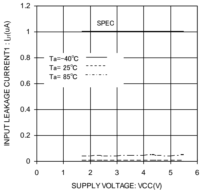
Figure 11. 入力リーク電流 1 I_{LI1}(SK)
