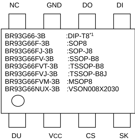
Figure 3. 端子配置図
