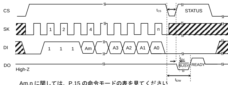
Figure 39. 消去サイクルタイミング
