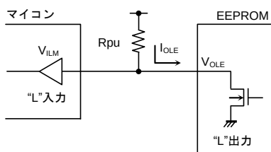
Figure 46. DO プルアップ抵抗
