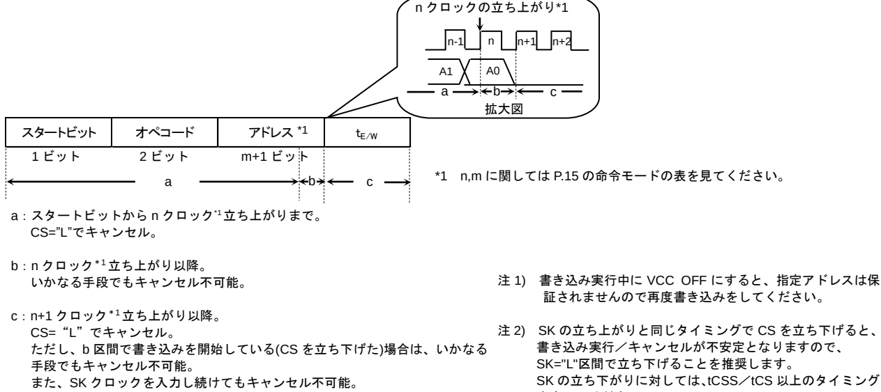
Figure 43. ERASE, ERAL キャンセル有効タイミング
