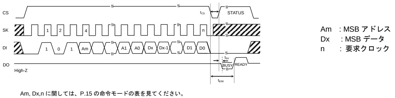
Figure 36. 書き込みサイクル
