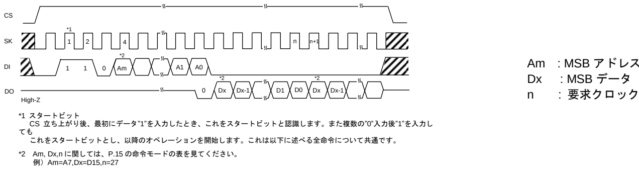
Figure 35. 読み出しサイクル
