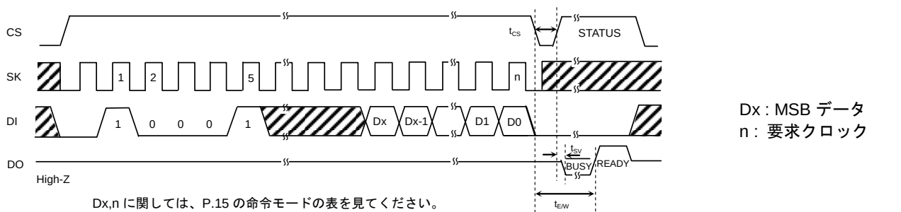
Figure 37. 全アドレス書き込みサイクル
