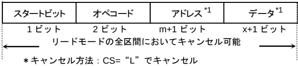
Figure 41. READ キャンセル有効タイミング
