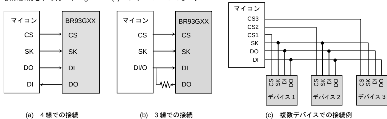
Figure 34. マイコンとの接続方法
