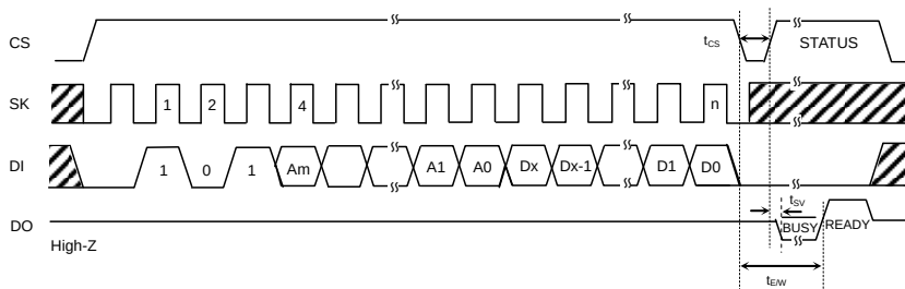
Figure 36. 書き込みサイクル
