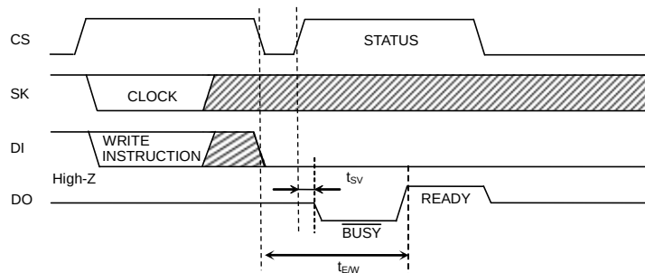
Figure 48. \overline{RDY} STATUS 出力タイミング図
