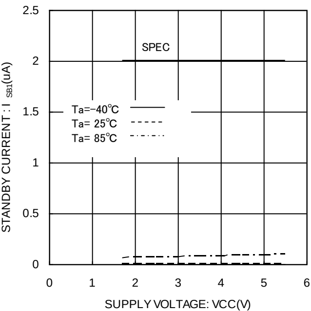
Figure 20. スタンバイ電流 I_{SBI} (CS=0V)
