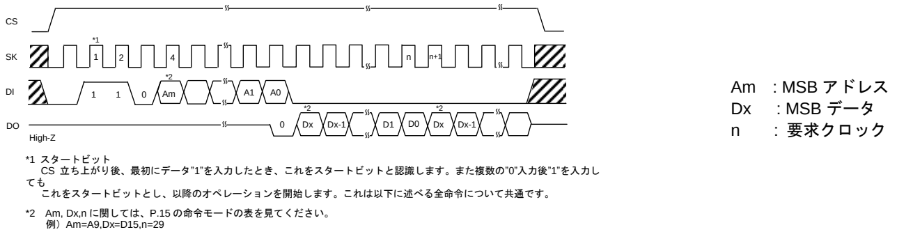
Figure 35. 読み出しサイクル
