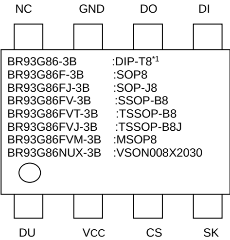
Figure 3. 端子配置図
