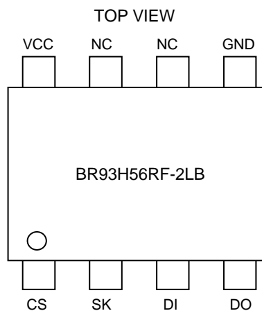
Figure 3. 端子配置図
