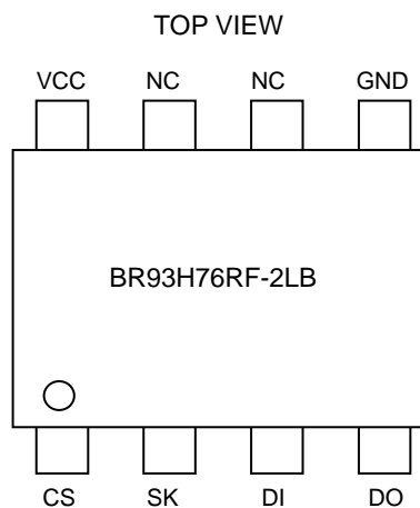
Figure 3. 端子配置図
