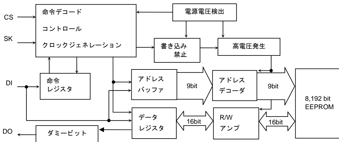
Figure 2. ブロック図
