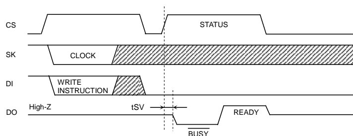
Figure 44. \overline{RDY} ステータス出力タイミング図
