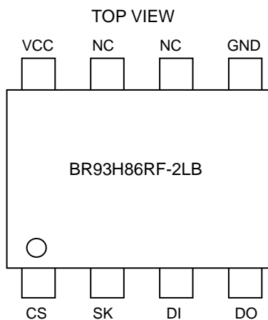
Figure 3. 端子配置図
