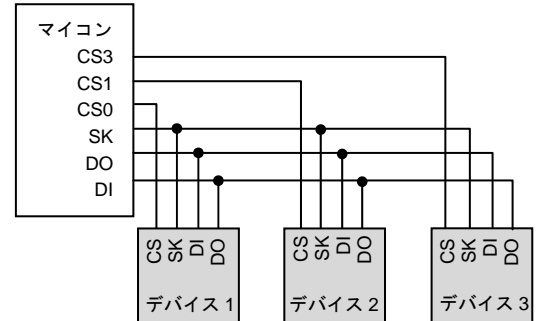
Fig 29-(c). 複数デバイスでの接続例
