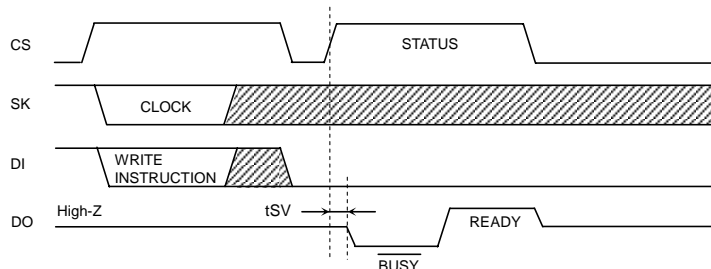
Figure 44. R/B ステータス出力タイミング図
