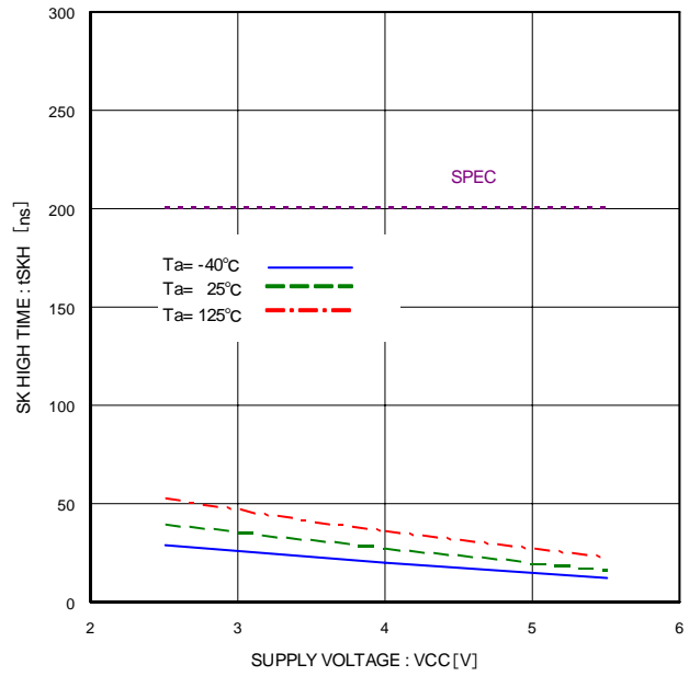
Figure 17. SK ハイ時間 tSKH
