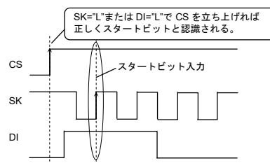
Figure 43. 正常動作タイミング
