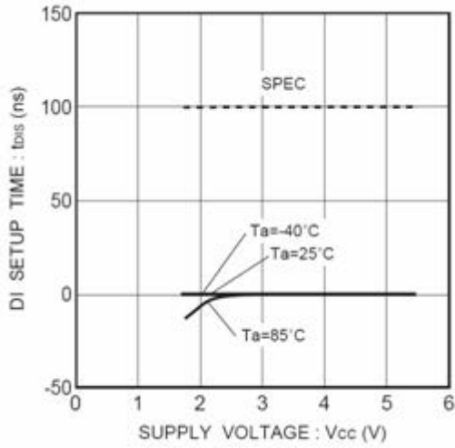
Figure 26. DI セットアップ時間 tDIS
