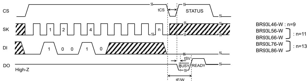
Figure 38. チップ消去サイクルタイミング
