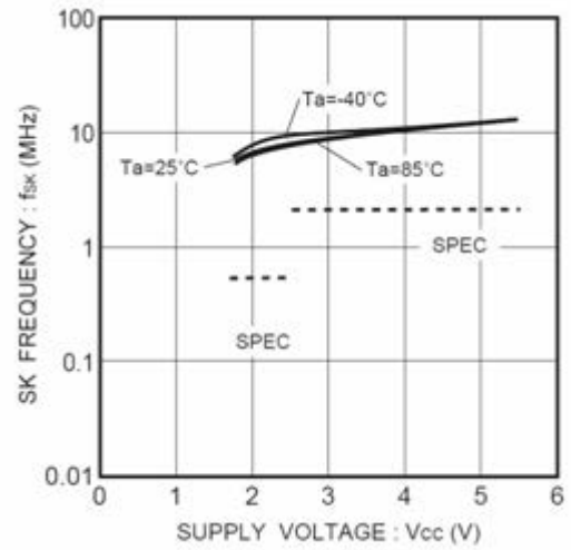
Figure 19. SK 周波数 f_{SK}
