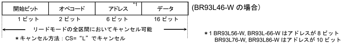
Figure 39. READ キャンセル有効タイミング
