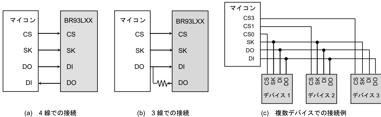
Figure 32. マイコンとの接続方法
