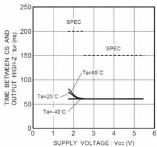
Figure 30. CS より出力 High-Z までの時間 t_{DF}
