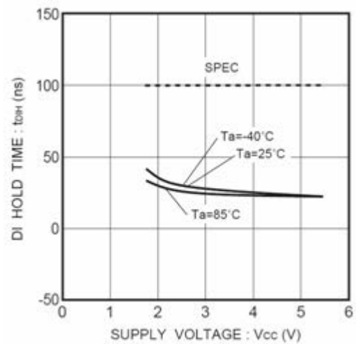
Figure 25. DI ホールド時間 tDIH
