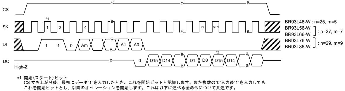
Figure 33. 読み出しサイクル
