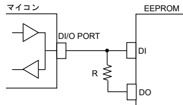
Figure 53. DI, DO 制御ライン共用接続
