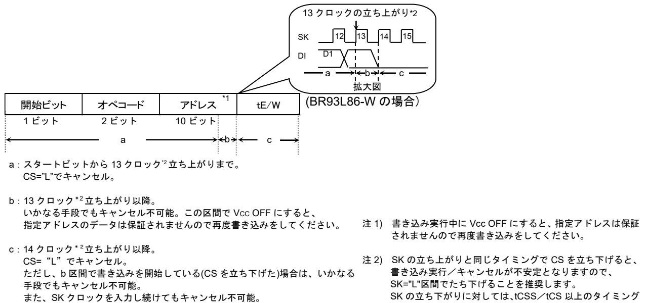
Figure 41. ERASE, ERAL キャンセル有効タイミング
