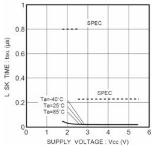
Figure 21. SK "L"時間 t_{SKL}
