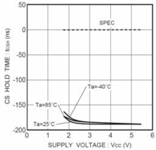
Figure 23. CS ホールド時間 tCSH
