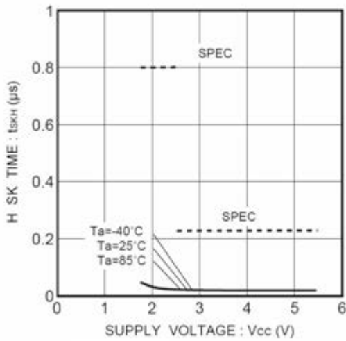
Figure 20. SK "H"時間 t_{SKH}
