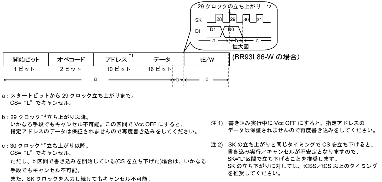
Figure 40. WRITE, WRAL キャンセル有効タイミング
