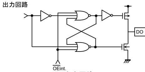
Figure 44. 出力回路(DO)
