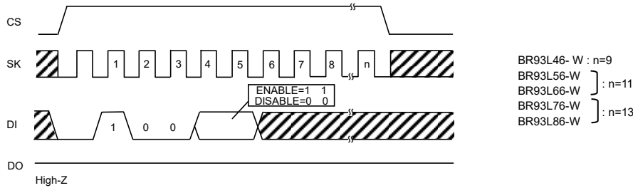
Figure 36. 書き込み可能 / 禁止サイクル
