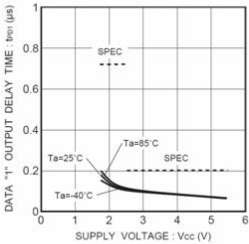
Figure 28. データ "1" 出力遅延時間 tPD1
