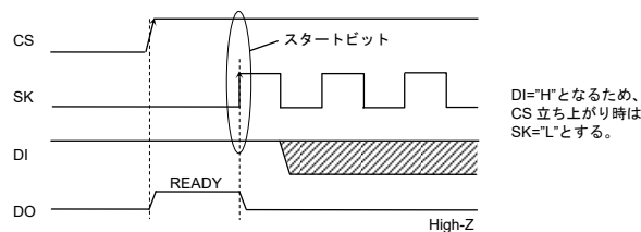
Figure 56. DI, DO 直結時スタートビット入力タイミング
