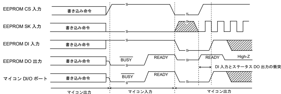
Figure 55. DI, DO 直結時書き込み時の衝突タイミング
