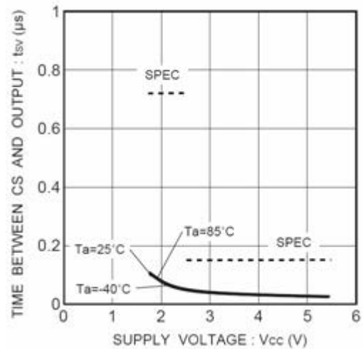
Figure 29. CS より出力確定までの時間 tSV
