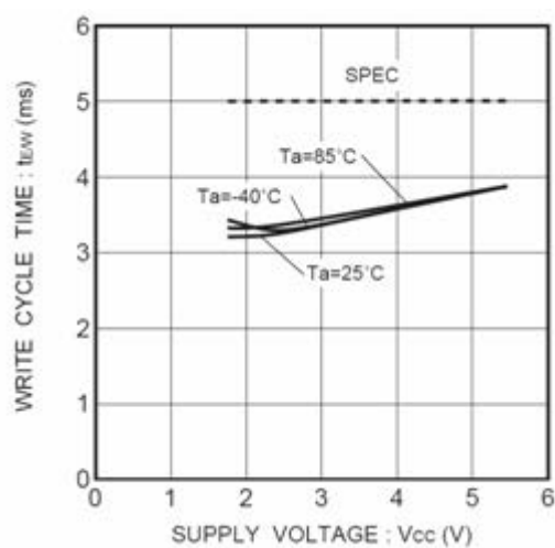
Figure 31. 書き込みサイクル時間 t_{EW}
