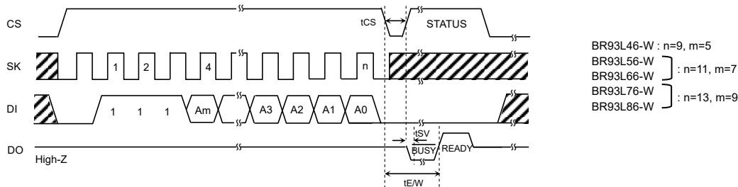
Figure 37. 消去サイクルタイミング
