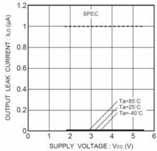
Figure 11. 出力リーク電流 ILO (DO)
