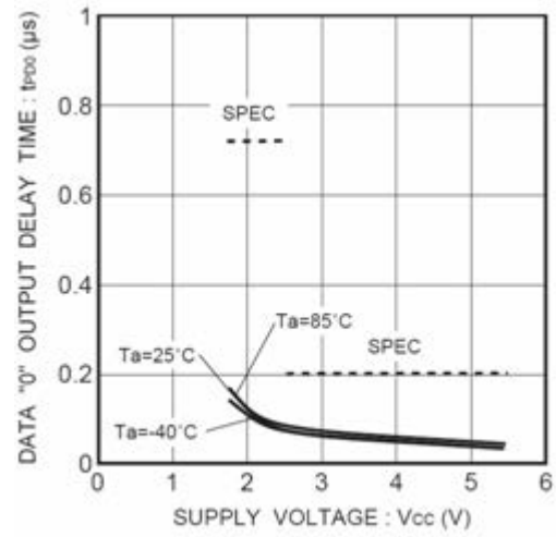
Figure 27. データ "0" 出力遅延時間 tPD0
