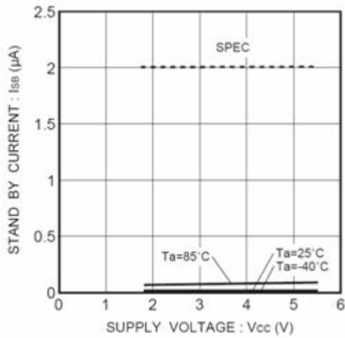
Figure 18. スタンバイ電流 I_{SB}
