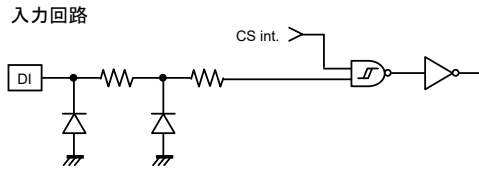
Figure 46. 入力回路(DI)
