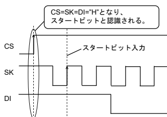
Figure 42. 誤動作タイミング
