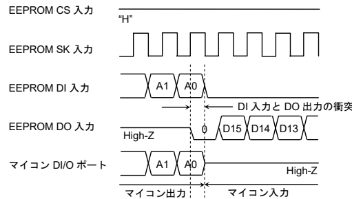
Figure 54. DI, DO 直結時リードデータ出力時の衝突タイミング
