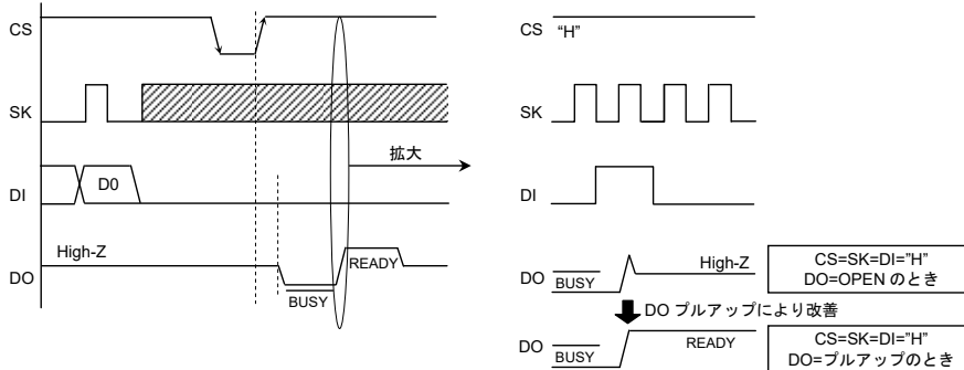
Figure 49. DO=OPEN 時 READY 出力時タイミング
