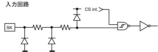
Figure 47. 入力回路(SK)
