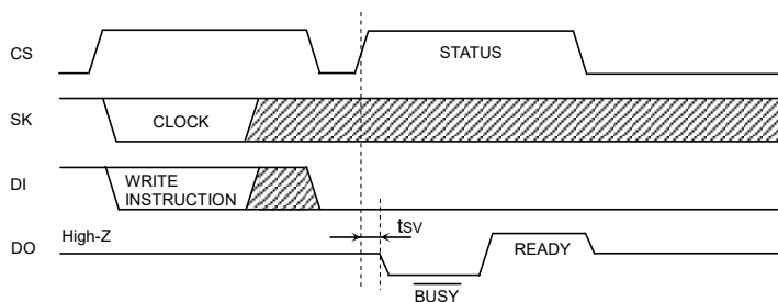
Figure 52. \overline{RDY} ステータス出力タイミング図
