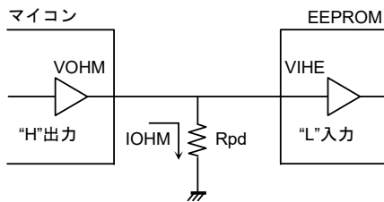
Figure 48. CS プルダウン抵抗
