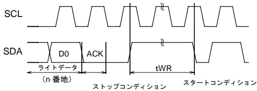
Figure 1-(c) 書き込みサイクルタイミング
