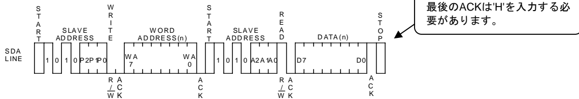
Figure 30. ランダムリードサイクル
