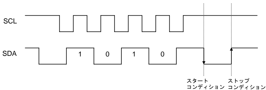
Figure 36. スレーブアドレス入力中にスタート・ストップコンディションでキャンセルした場合
