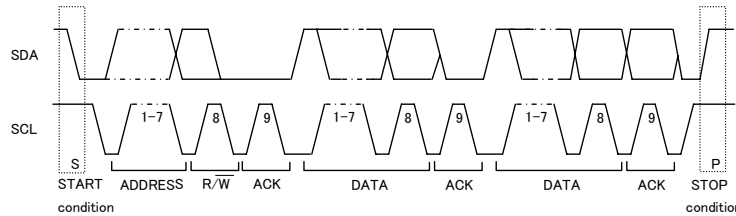
Figure 26. データ転送タイミング
