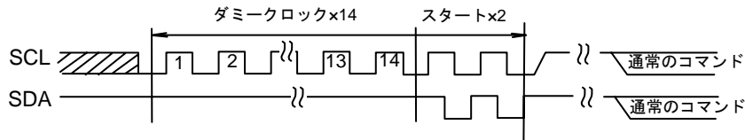
Figure 33-(a) 14 ダミークロック+START+START+コマンド入力の場合
