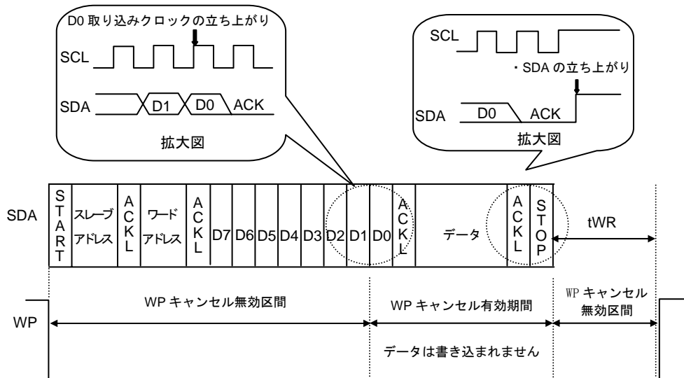
Figure 35. WP 有効タイミング
