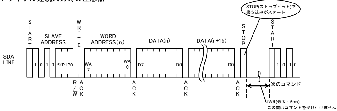
Figure 29. ページライトサイクル
