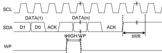
Figure 1-(d) ライト実行時 WP タイミング
