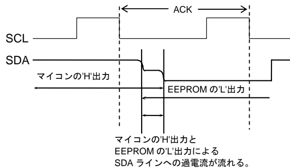
Figure 39. 入出力衝突タイミング
