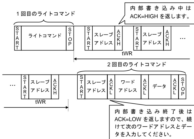
Figure 34. アクノリッジポーリングで連続して書き込みを行う場合
