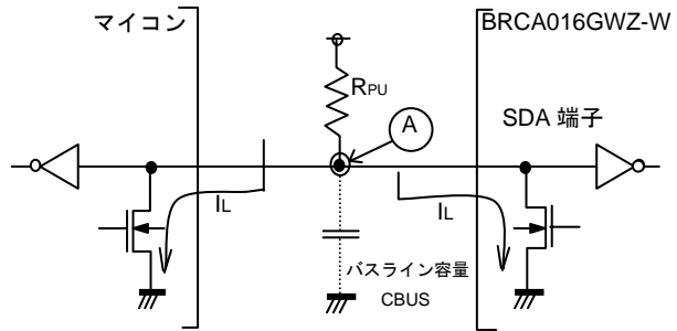
Figure 37. I/O 回路図
