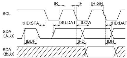
Figure 1-(a) 同期データ入出カタイミング
