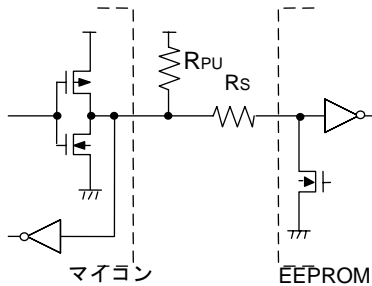
Figure 38. I/O 回路図
