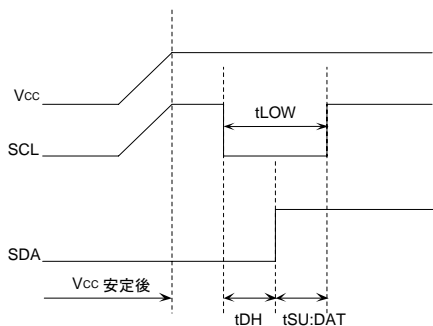
Figure 45. SCL='H' SDA='L'の時
