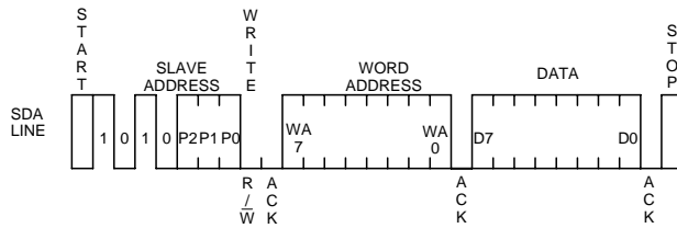
Figure 27. バイトライトサイクル
