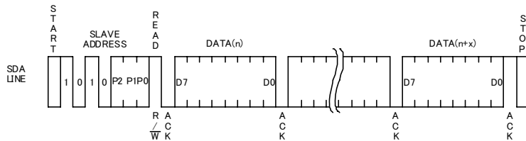
Figure 32. シーケンシャルリードサイクル (カレントリードサイクルの場合)
