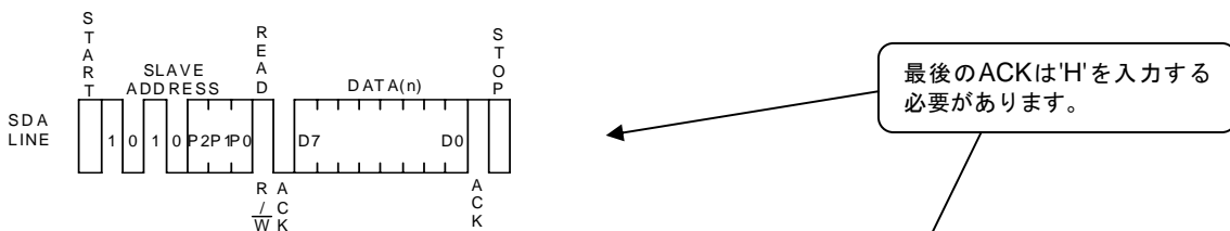
Figure 31. カレントリードサイクル
