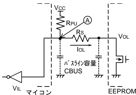
Figure 40. I/O 回路図
