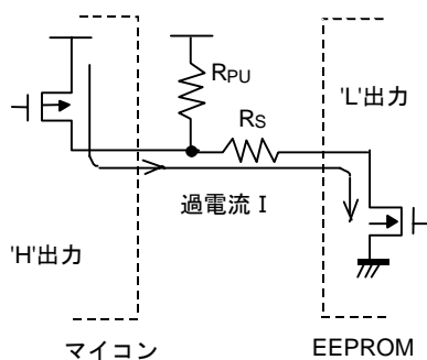
Figure 41. I/O 回路図
