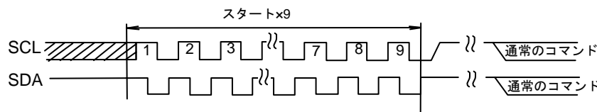
Figure 33-(c) START×9+コマンド入力の場合
