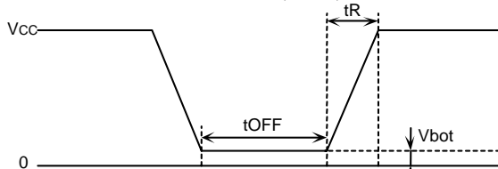
Figure 44. 立ち上がり波形図
