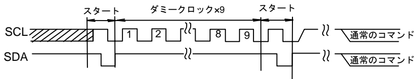
Figure 33-(b) START+9 ダミークロック+START+コマンド入力の場合
