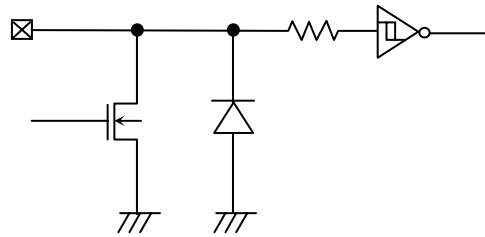
Figure 43. 入出力 pin 回路図
