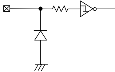
Figure 42. 入力 pin 回路図
