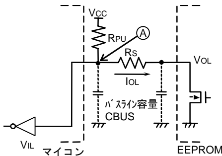
Figure 39. I/O 回路図
