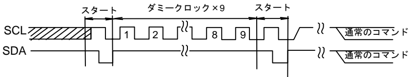
Figure 33-(b). START+ダミークロック × 9 + START + コマンド入力の場合
