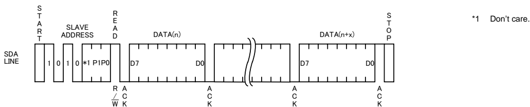
Figure 31. シーケンシャルリードサイクル (カレントリードサイクルの場合)
