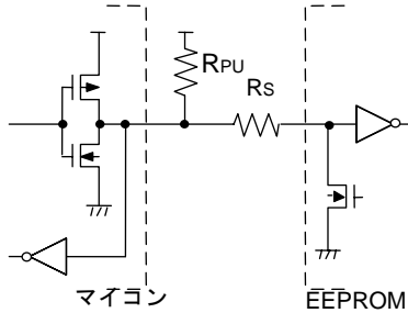
Figure 37. I/O 回路図
