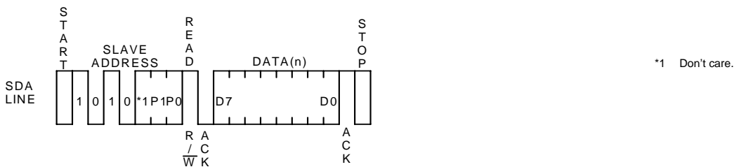
Figure 30. カレントリードサイクル
