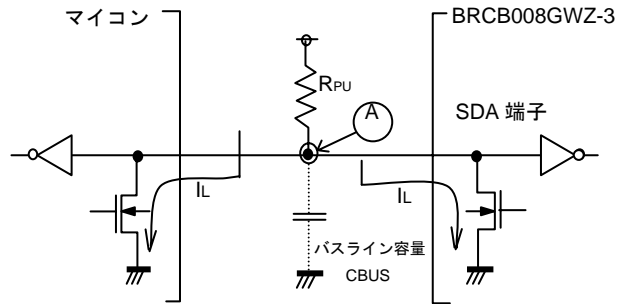
Figure 36. I/O 回路図
