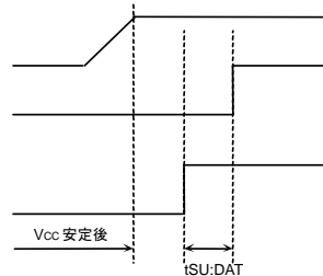
Figure 45. SCL='H' SDA='L'の時
