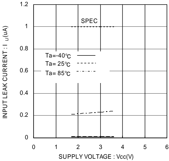
Figure 7. 入力リーク電流 I_{LI} (SCL)
