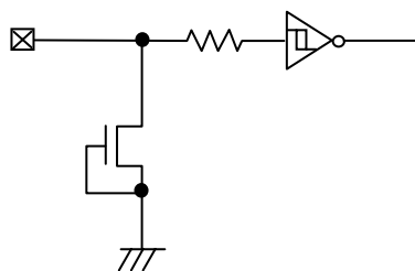
Figure 41. 入力 pin 回路図
