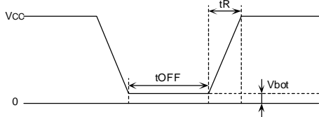
Figure 43. 立ち上がり波形図
