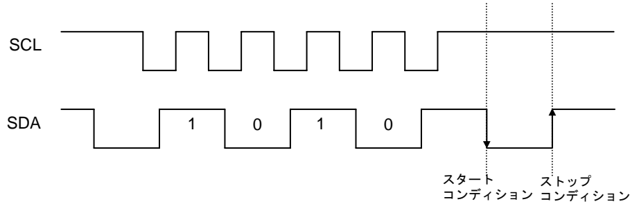
Figure 35. スレーブアドレス入力中にスタート・ストップコンディションでキャンセルした場合
