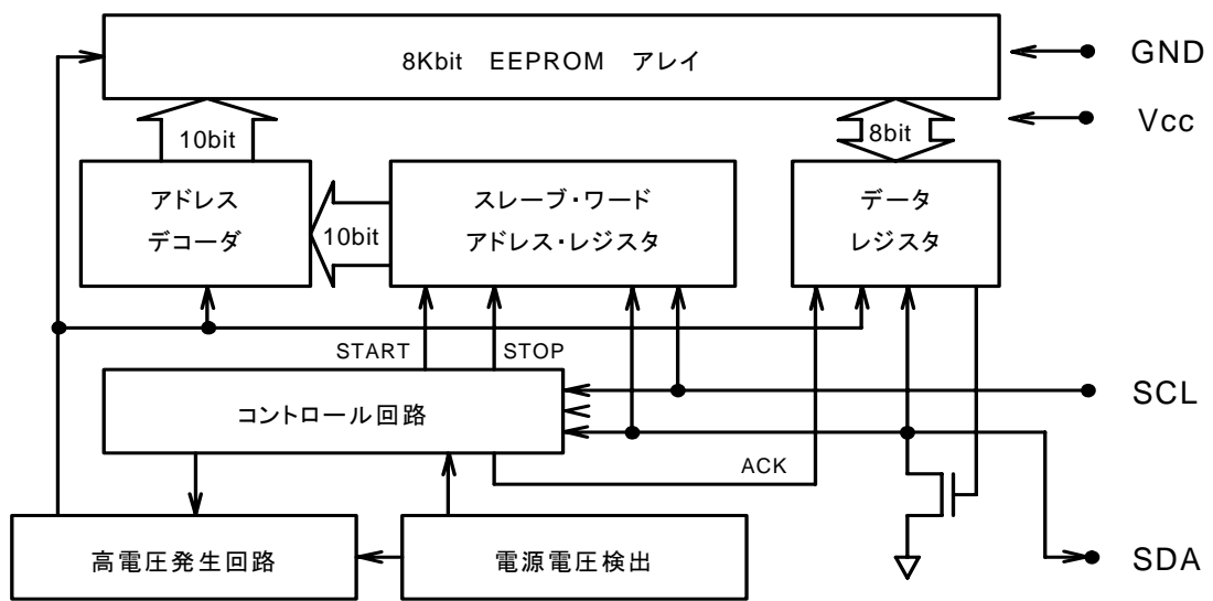
Figure 2. ブロック図
