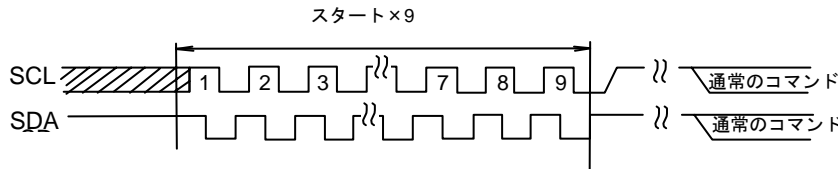
Figure 33-(c). START × 9 + コマンド入力の場合
