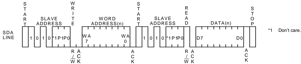
Figure 29. ランダムリードサイクル
