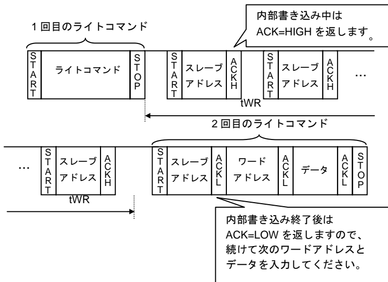
Figure 34. アクリリッジポーリングで連続して書き込みを行う場合
