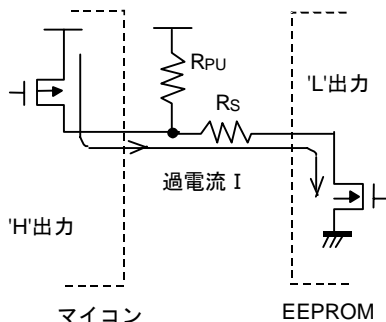
Figure 40. I/O 回路図
