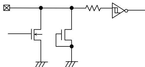
Figure 42. 入出力 pin 回路図
