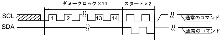
Figure 33-(a). 14 ダミークロック × 14 + START + START + コマンド入力の場合
