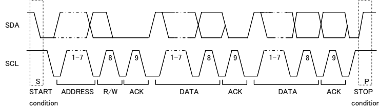
Figure 26. データ転送タイミング
