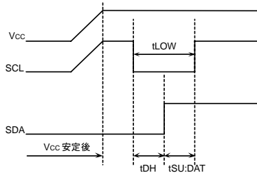
Figure 44. SCL='H' SDA='L'の時
