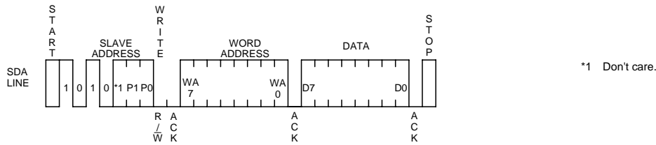
Figure 27. バイトライトサイクル
