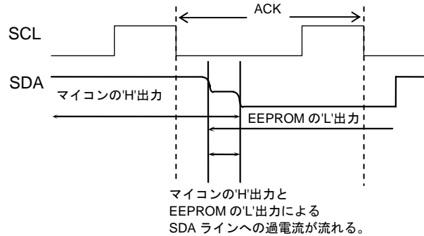
Figure 38. 入出力衝突タイミング
