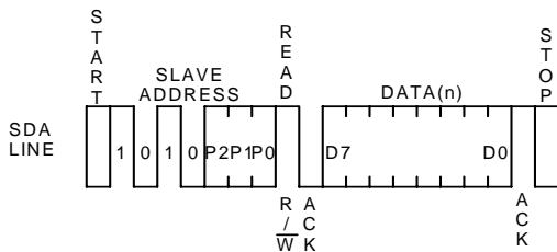
Figure 33. カレントリードサイクル
