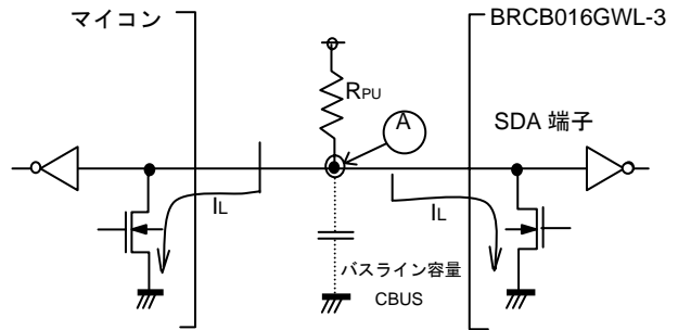
Figure 39. I/O 回路図
