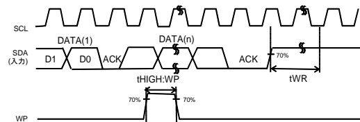
Figure 1-(e). ライトキャンセル時 WP タイミング
