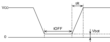
Figure 46. 立ち上がり波形図
