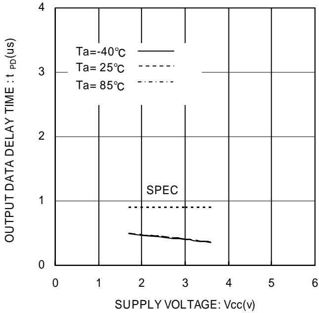
Figure 19. 'L'出力データ遅延時間 t_{PD0}
