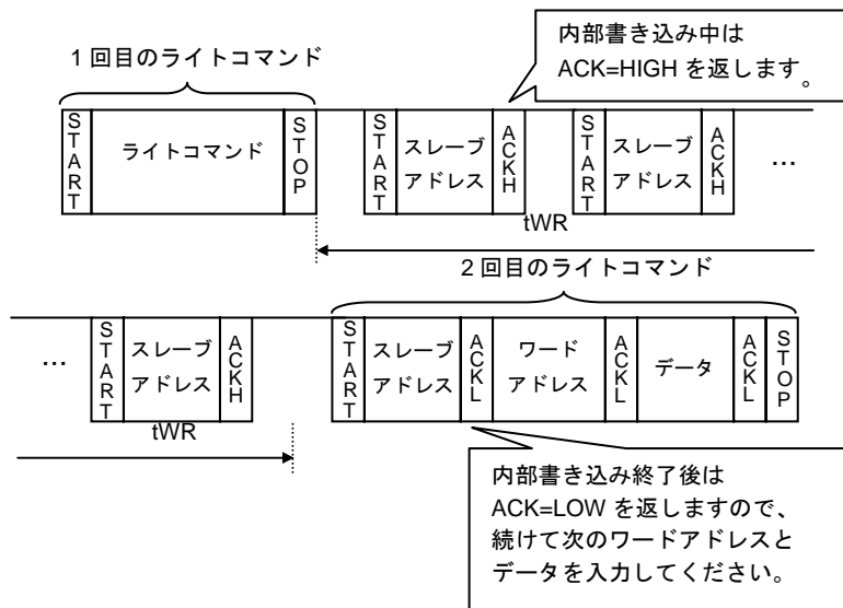
Figure 36. アクノリッジポーリングで連続して書き込みを行う場合
