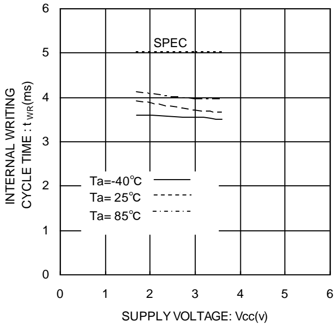
Figure 23. 内部書き込みサイクル時間 t_{WR}
