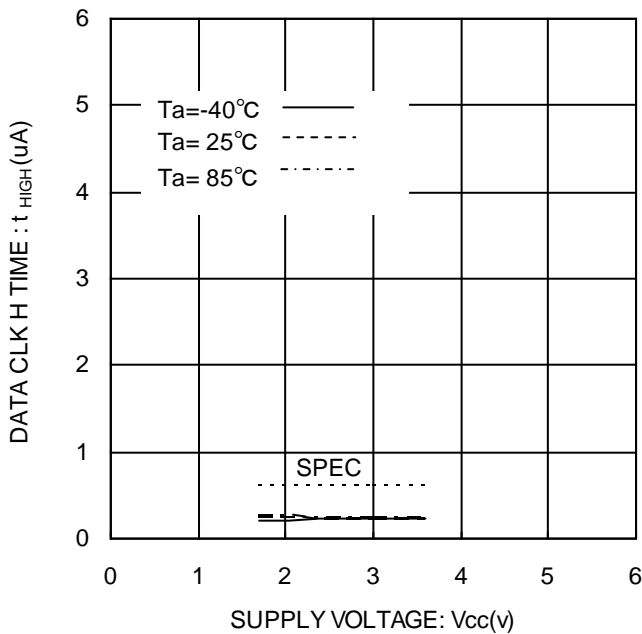
Figure 13. データクロック'H'時間 t_{HIGH}
