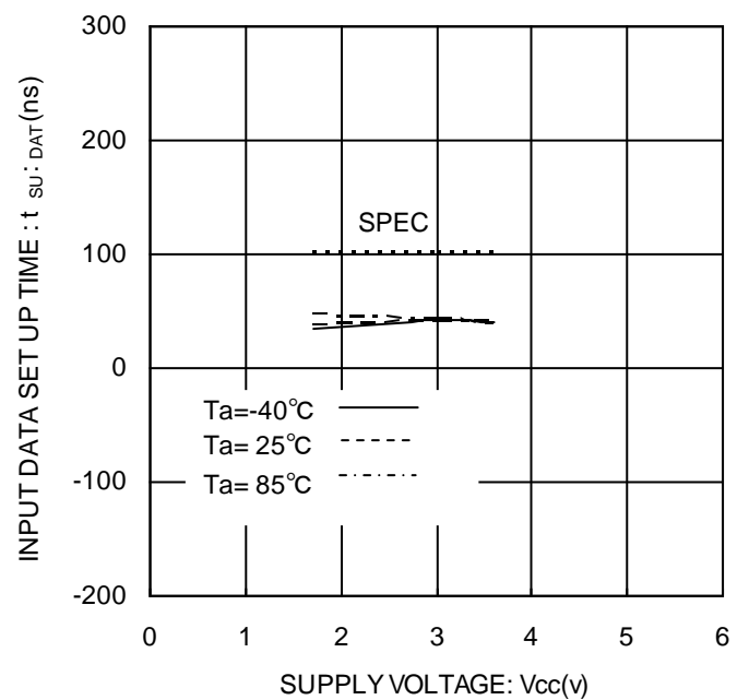
Figure 18. 入力データセットアップ時間 t_{SU:DAT}
