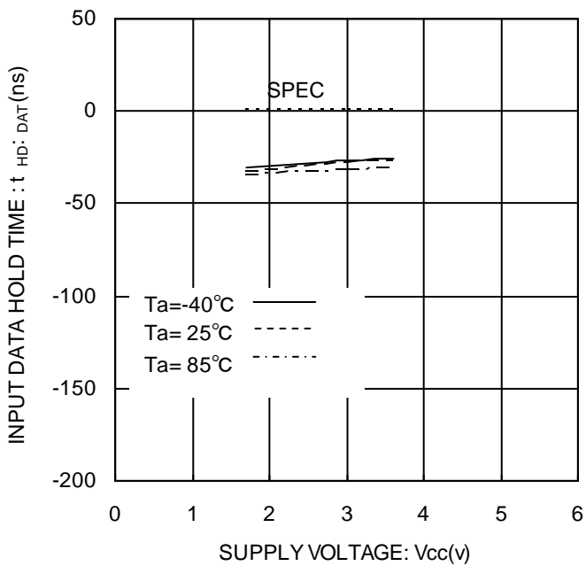
Figure 17. 入力データホールド時間 t_{HD:DAT}
