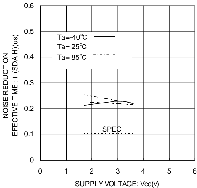
Figure 25. ノイズ除去有効時間 t_l (SDA H)
