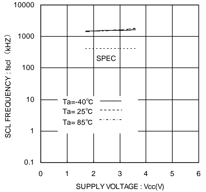
Figure 12. SCL 周波数 f_{SCL}
