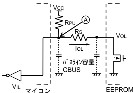
Figure 42. I/O 回路図
