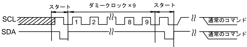
Figure 35-(b). START+ダミークロック × 9 + START + コマンド入力の場合
