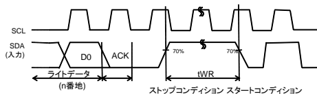
Figure 1-(c). 書き込みサイクルタイミング
