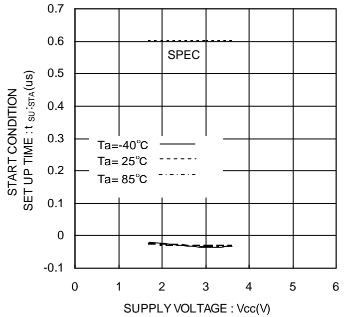
Figure 16. スタートコンディションセットアップ時間 t_{SU:STA}
