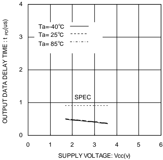
Figure 19. 'L'出力データ遅延時間 t_{PD0}
