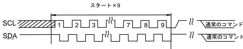
Figure 35-(c). START × 9 + コマンド入力の場合
