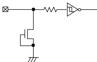
Fig 44. 入力 pin 回路図
