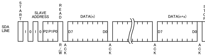
Figure 34. シーケンシャルリードサイクル (カレントリードサイクルの場合)
