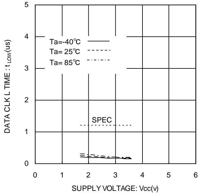
Figure 14. データクロック'L'時間 t_{LOW}
