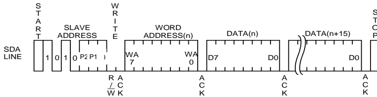
Figure 31. ページライトサイクル
