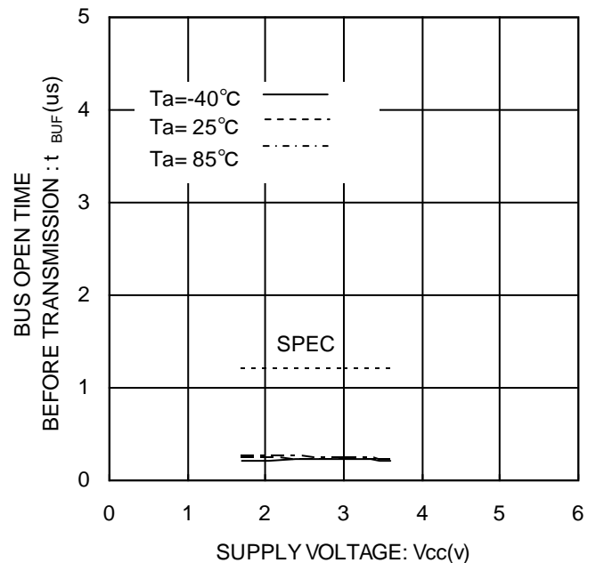
Figure 22. 転送開始前バス開放時間 t_{BUF}
