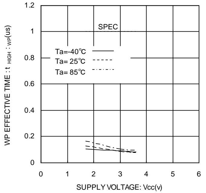
Figure 28. WP 有効時間 t_{HIGH} : WP
