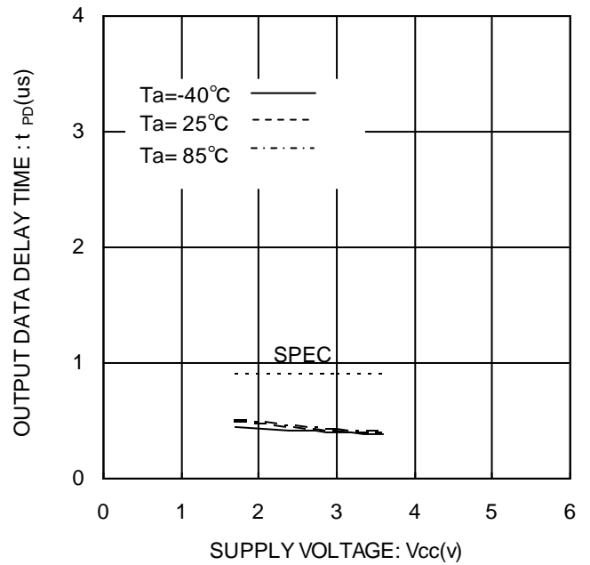
Figure 20. 'H'出力データ遅延時間 t_{PD1}
