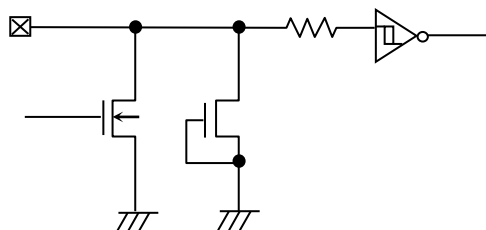
Fig 45. 入出力 pin 回路図
