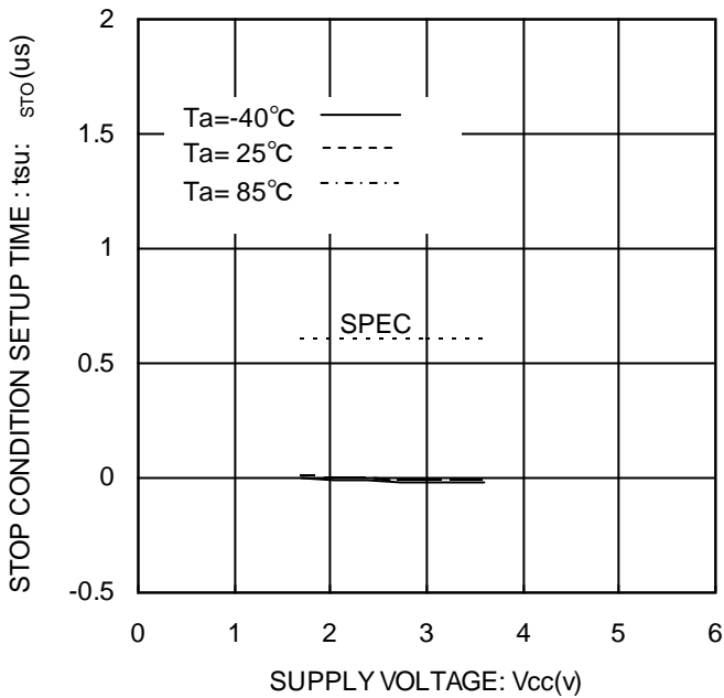
Figure 21. ストップコンディションセットアップ時間 t_{SU:STO}
