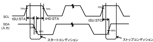
Figure 1-(b). スタート・ストップタイミング
