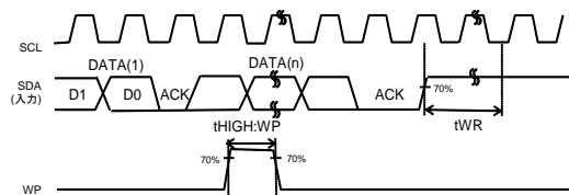
Figure 1-(d). ライト実行時 WP タイミング
