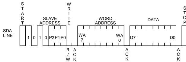
Figure 30. バイトライトサイクル
