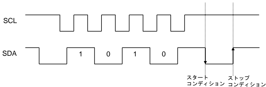
Figure 38. スレーブアドレス入力中にスタート・ストップコンディションでキャンセルした場合
