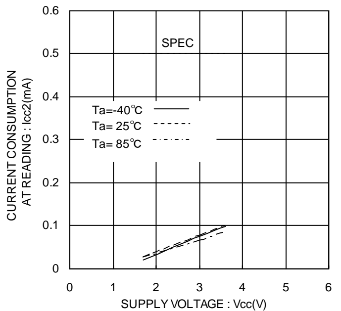
Figure 10. リード動作時消費電流 I_{cc2} ( f_{scl}=400kHz )
