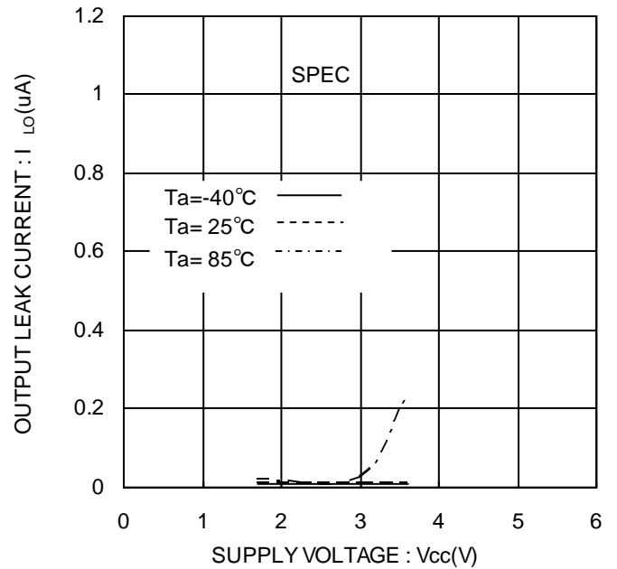
Figure 8. 出力リーク電流 I_{Lo} (SDA)
