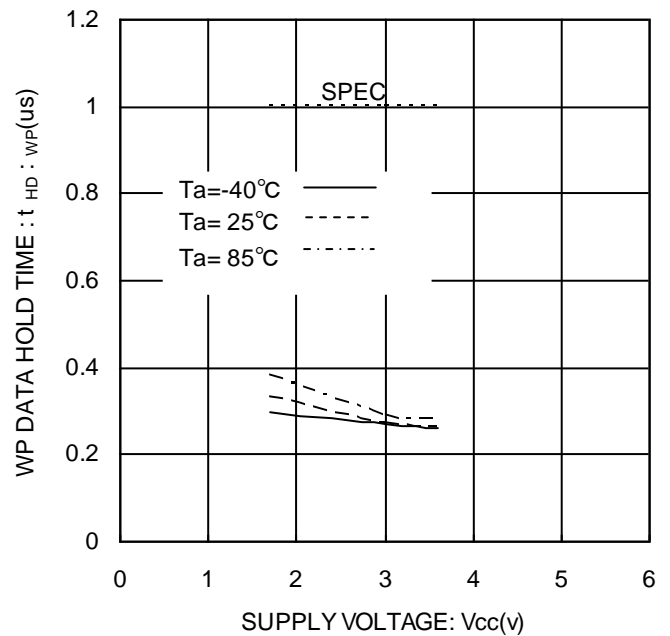
Figure 26. WP ホールド時間 t_{DH:WP}
