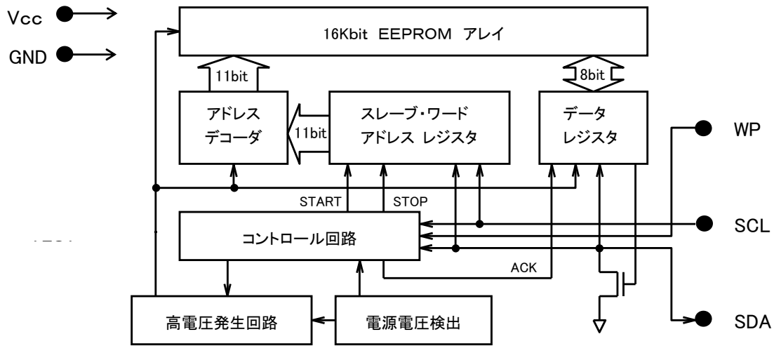
Figure 2. ブロック図
