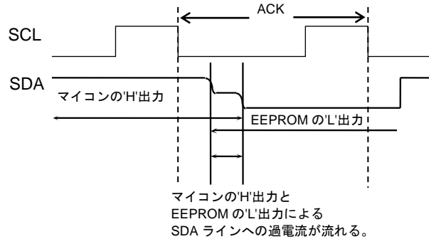
Figure 41. 入出力衝突タイミング
