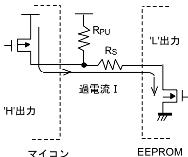
Figure 43. I/O 回路図
