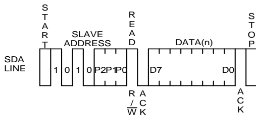
Figure 33. カレントリードサイクル
