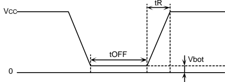
Figure 46. 立ち上がり波形図
