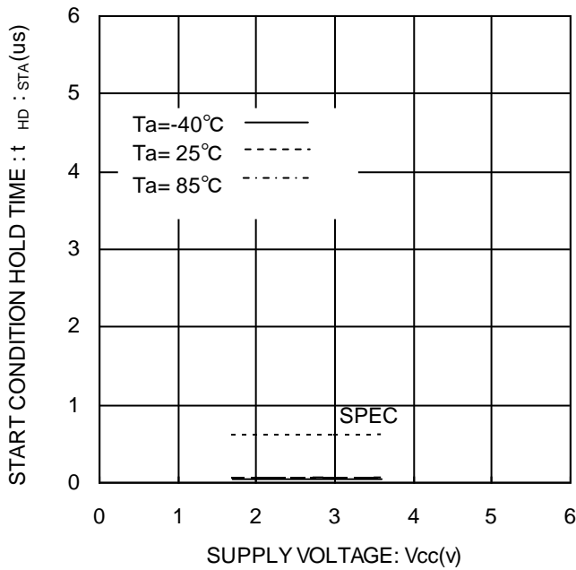
Figure 15. スタートコンディションホールド時間 t_{HD:STA}
