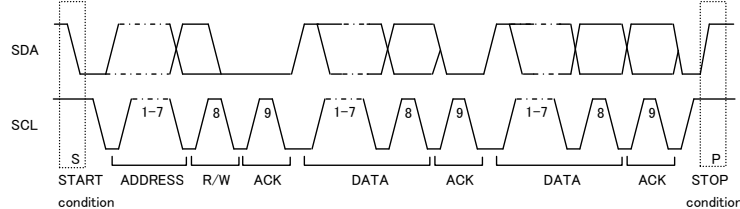
Figure 29. データ転送タイミング
