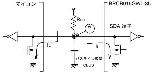
Figure 39. I/O 回路図
