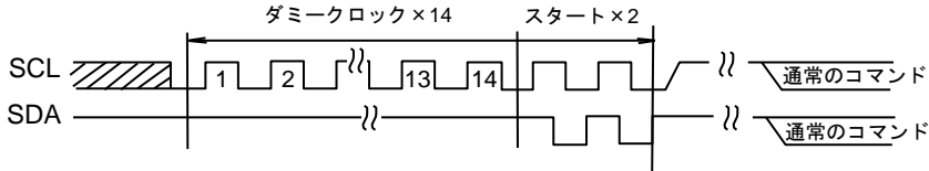
Figure 35-(a). 14 ダミークロック × 14 + START + START + コマンド入力の場合
