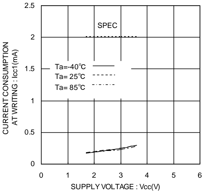
Figure 9. ライト動作時消費電流 I_{cc1} ( f_{scl}=400kHz )
