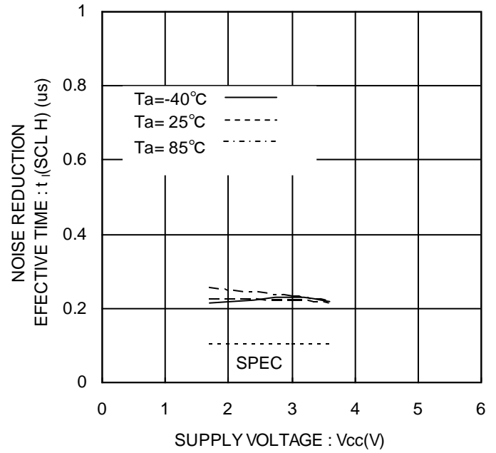
Figure 24. ノイズ除去有効時間 t_l (SCL H)
