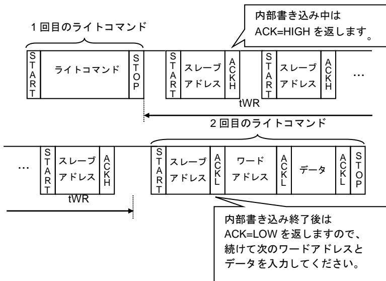
Figure 36. アクノリッジポーリングで連続して書き込みを行う場合
