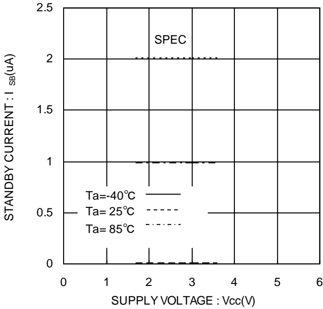
Figure 11. スタンバイ電流 I_{SB}
