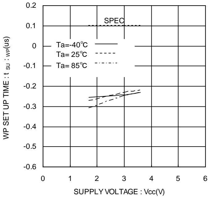
Figure 27. WP セットアップ時間 t_{SU} : WP
