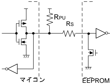
Figure 40. I/O 回路図
