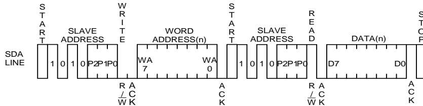
Figure 32. ランダムリードサイクル
