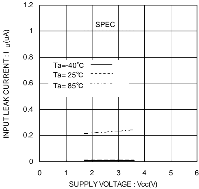
Figure 7. 入力リーク電流 I_i (SCL)
