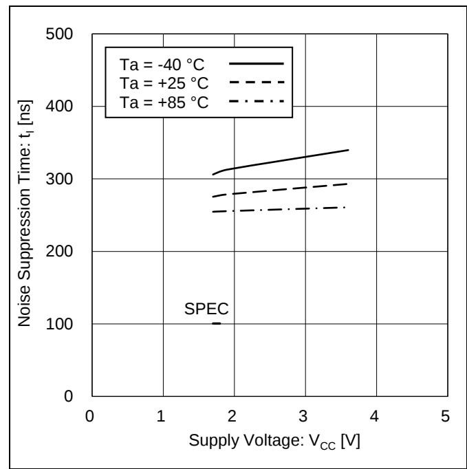
Figure 32. ノイズ除去有効時間 vs 電源電圧 (SCL 'LOW')
