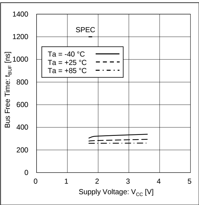
Figure 29. バス開放時間 vs 電源電圧
