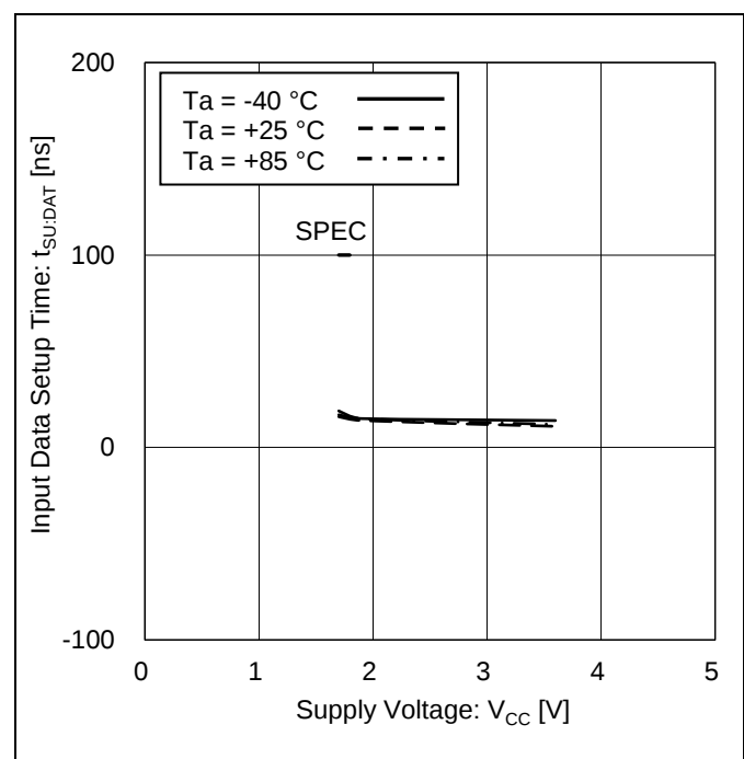
Figure 22. 入力データセットアップ時間 vs 電源電圧 (SDA 'LOW' to 'HIGH')
