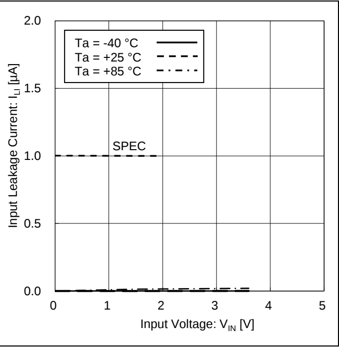
Figure 9. 入力リーク電流 vs 入力電圧
