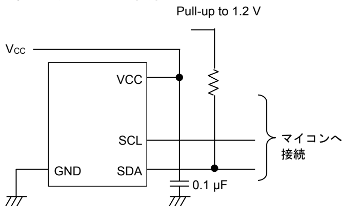
Figure 1. 基本アプリケーション回路図
