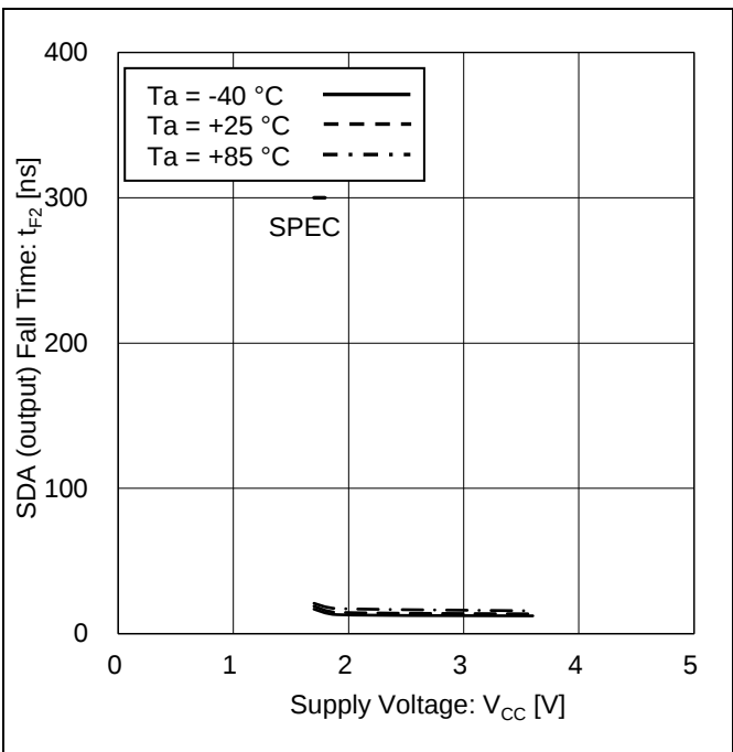
Figure 17. SDA の出力立ち下がり時間 vs 電源電圧
