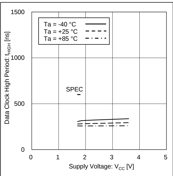
Figure 15. データクロック 'HIGH' 時間 vs 電源電圧
