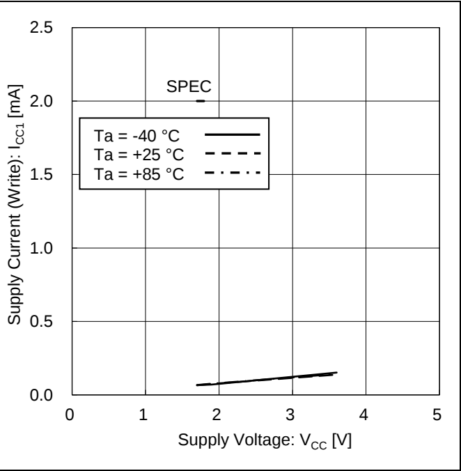
Figure 11. 消費電流 (ライト) vs 電源電圧 ( f_{SCL} = 400\text{ kHz} )
