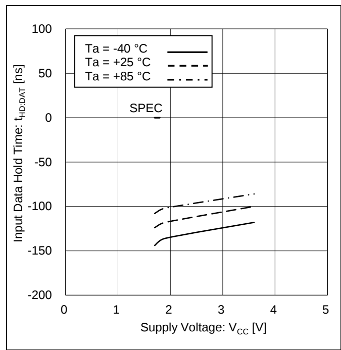
Figure 21. 入力データホールド時間 vs 電源電圧 (SDA 'HIGH' to 'LOW')
