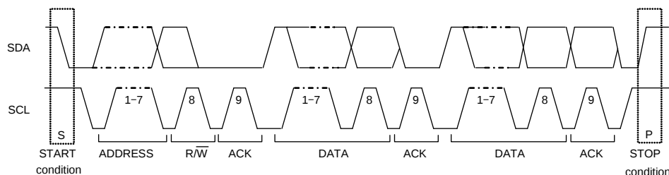
Figure 35. データ転送タイミング
