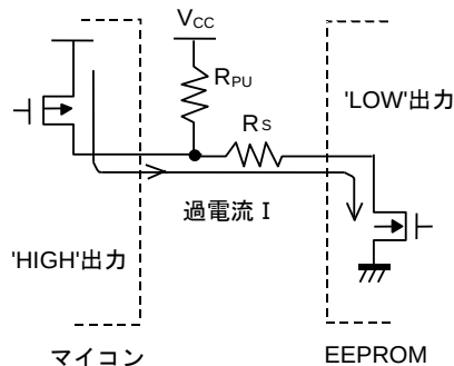
Figure 48. I/O 回路図
