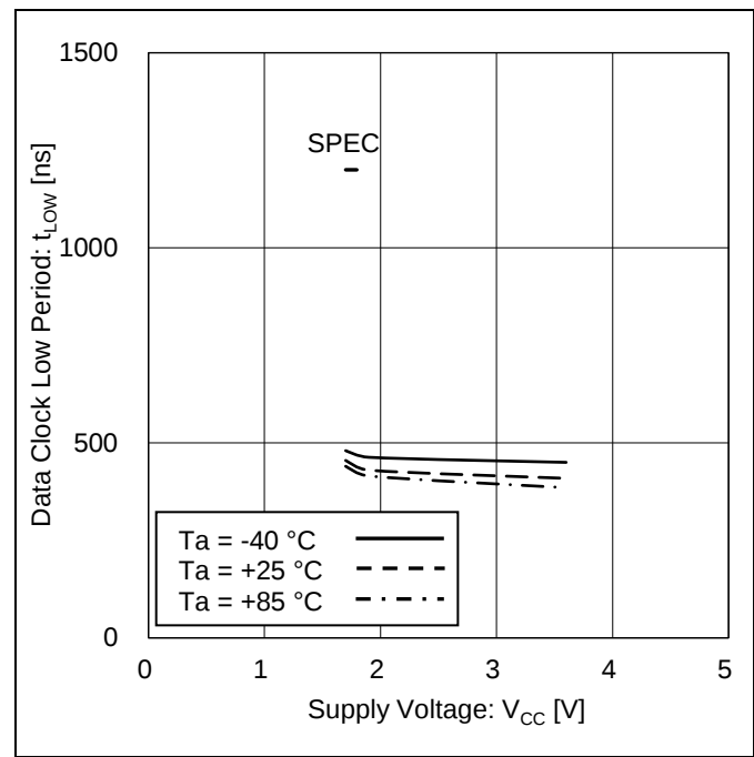
Figure 16. データクロック'LOW'時間 vs 電源電圧
