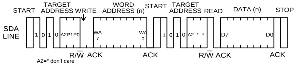
Figure 38. ランダムリード
