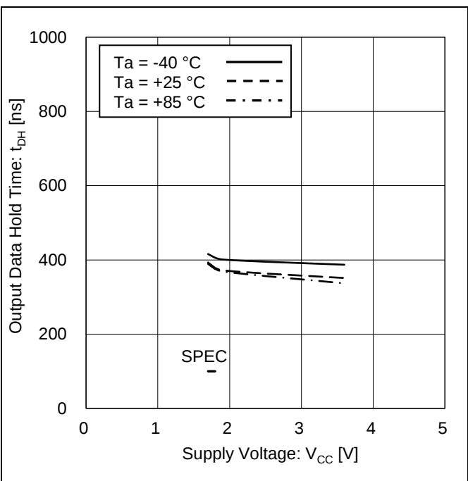
Figure 27. 出力データホールド時間 vs 電源電圧 (SDA 'HIGH' to 'LOW')
