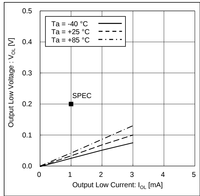
Figure 8. 'LOW'出力電圧 vs 'LOW'出力電流 ( V_{CC} = 1.7\text{ V} )
