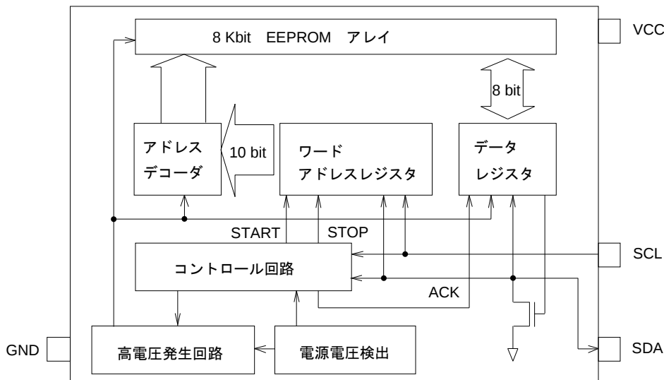
Figure 4. ブロック図
