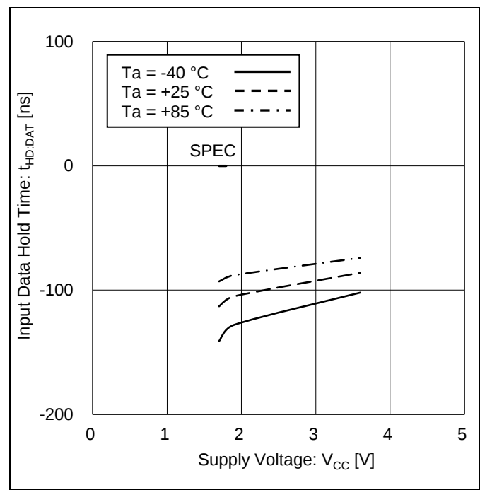
Figure 20. 入力データホールド時間 vs 電源電圧 (SDA 'LOW' to 'HIGH')
