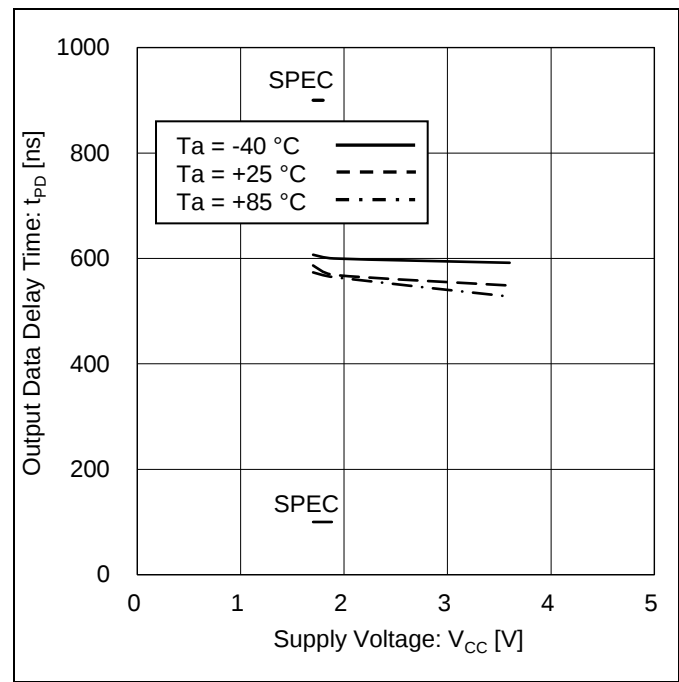
Figure 24. 出力データ遅延時間 vs 電源電圧 (SDA 'LOW' to 'HIGH')
