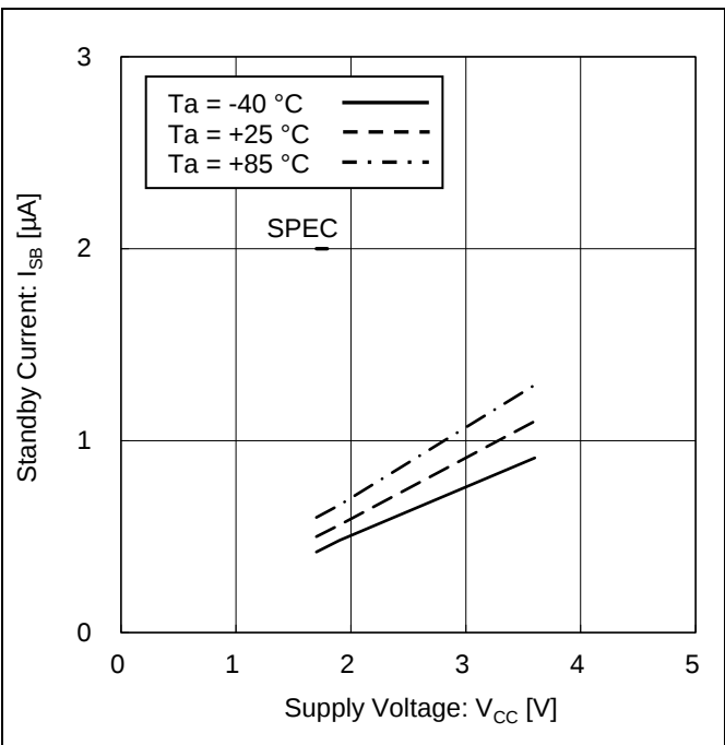
Figure 13. スタンバイ電流 vs 電源電圧
