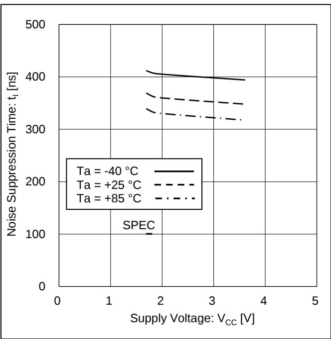
Figure 33. ノイズ除去有効時間 vs 電源電圧 (SDA 'HIGH')
