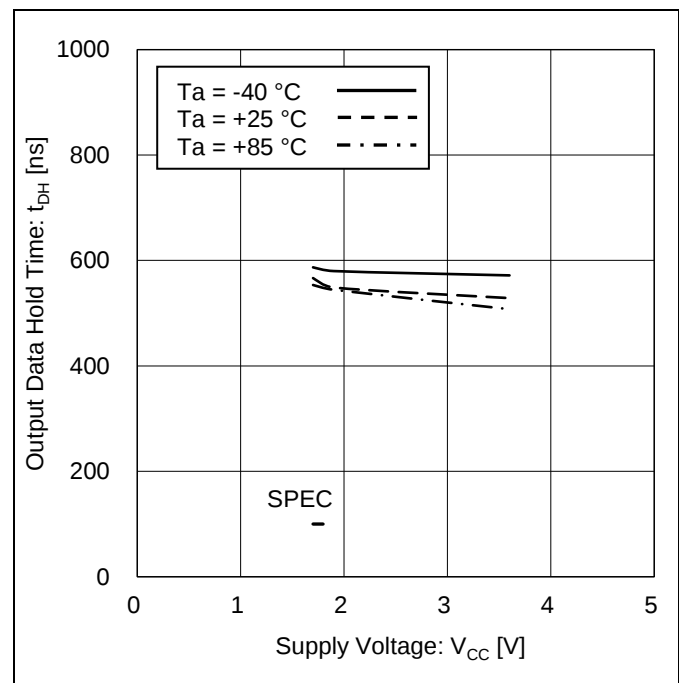
Figure 26. 出力データホールド時間 vs 電源電圧 (SDA 'LOW' to 'HIGH')
