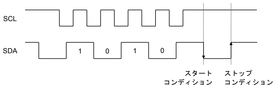
Figure 43. ターゲットアドレス入力中にスタート・ストップコンディションでキャンセルした場合
