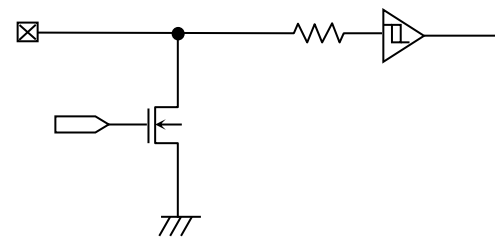
Figure 51. 入出力端子回路図 (SDA)
