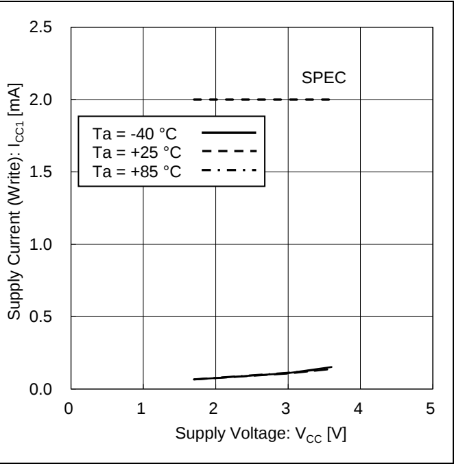
Figure 12. 消費電流 (ライト) vs 電源電圧 ( f_{SCL} = 400 \text{ kHz} )
