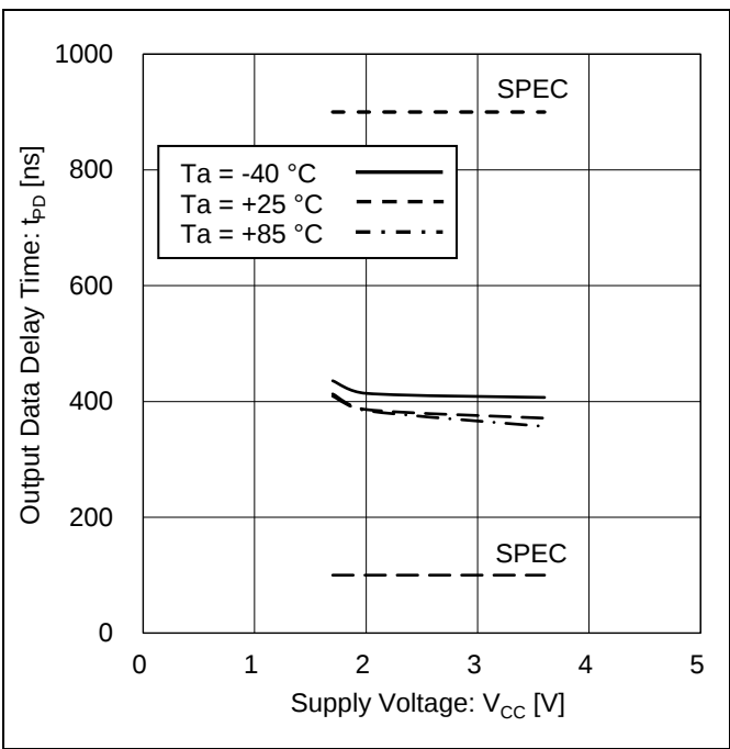
Figure 26. 出力データ遅延時間 vs 電源電圧 (SDA 'HIGH' to 'LOW')
