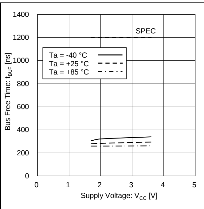
Figure 30. バス開放時間 vs 電源電圧
