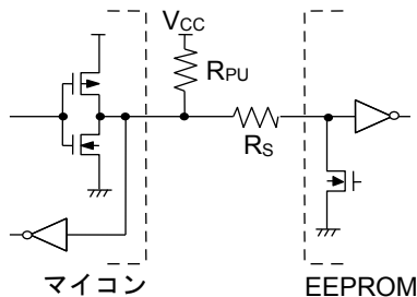
Figure 46. I/O 回路図
