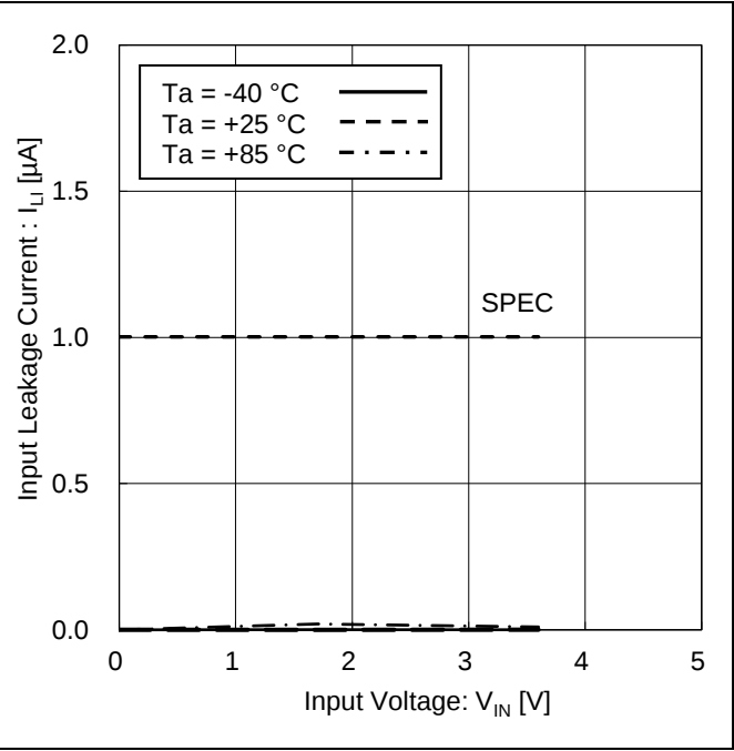
Figure 10. 入力リーク電流 vs 入力電圧
