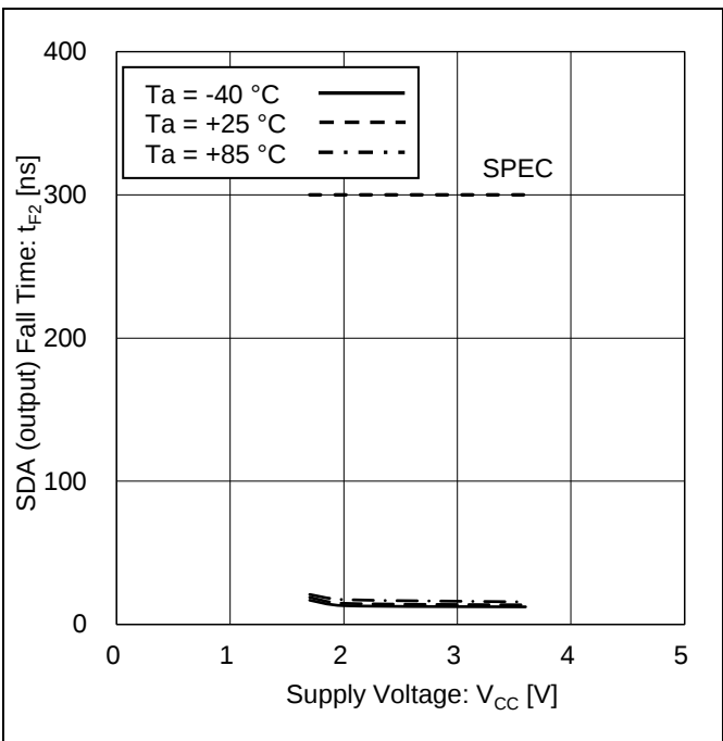
Figure 18. SDA の出力立ち下がり時間 vs 電源電圧
