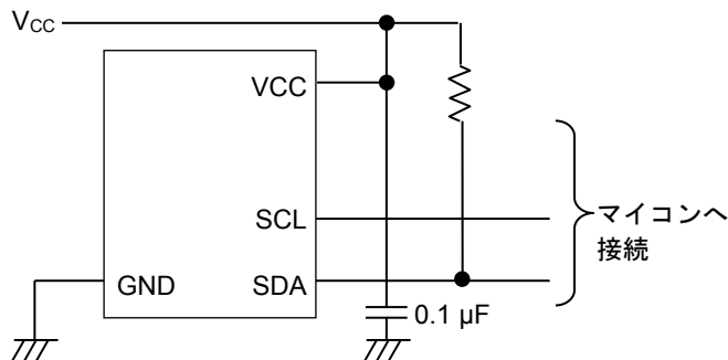
Figure 1. 基本アプリケーション回路図
