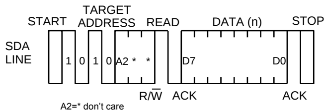
Figure 40. カレントリード
