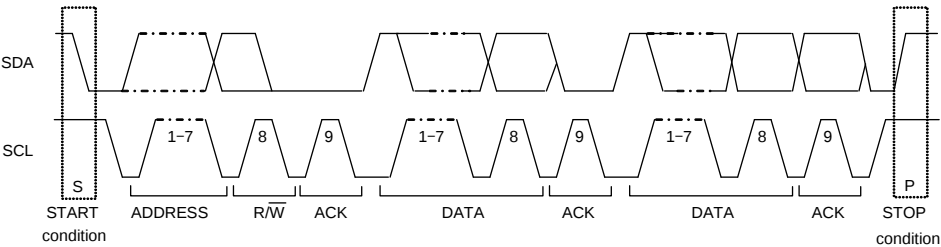
Figure 36. データ転送タイミング
