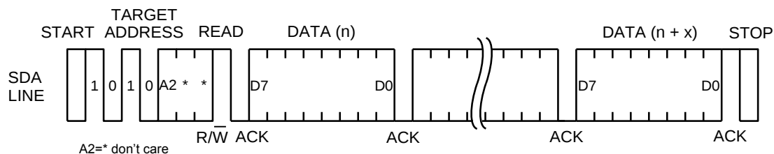
Figure 41. シーケンシャルリード (カレントリードの場合)
