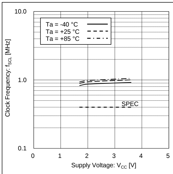
Figure 15. SCL 周波数 vs 電源電圧
