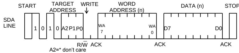
Figure 37. バイトライト
