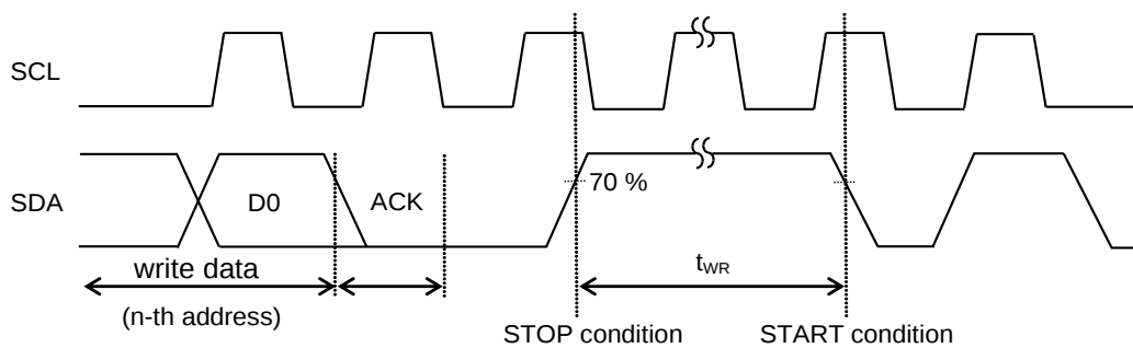
Figure 5-(c). 書き込みタイミング
