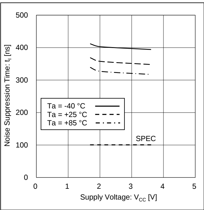
Figure 34. ノイズ除去有効時間 vs 電源電圧 (SDA 'HIGH')
