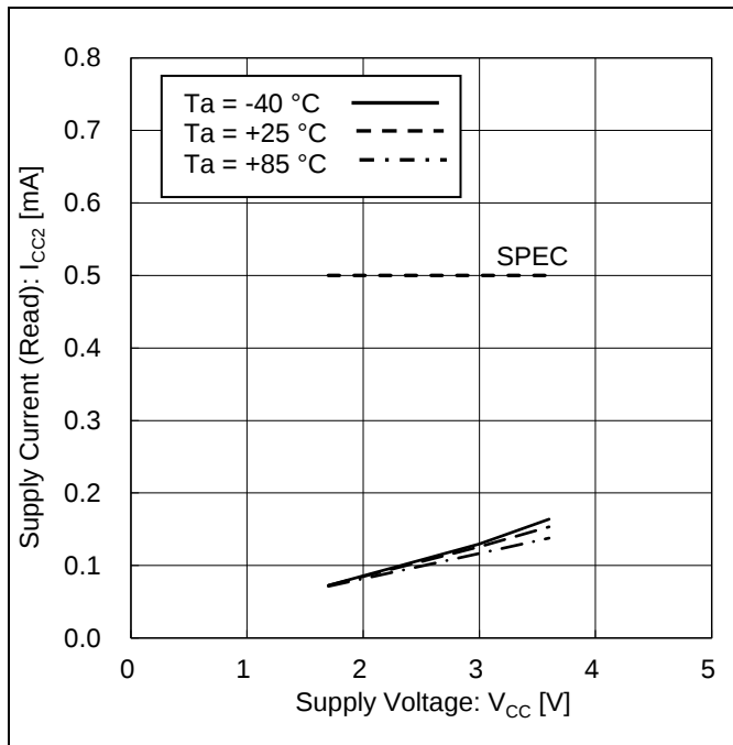
Figure 13. 消費電流 (リード) vs 電源電圧 ( f_{SCL} = 400 \text{ kHz} )
