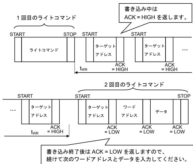
Figure 43. アクノリッジポーリングで連続して書き込みを行う場合
