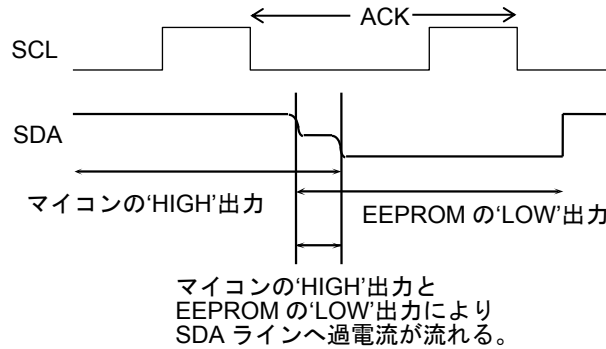
Figure 47. 入出力衝突タイミング
