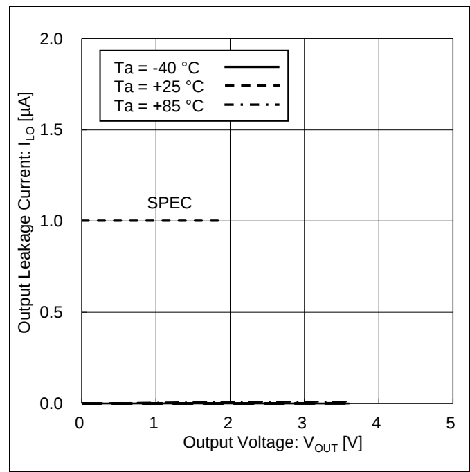
Figure 10. 出力リーク電流 vs 出力電圧
