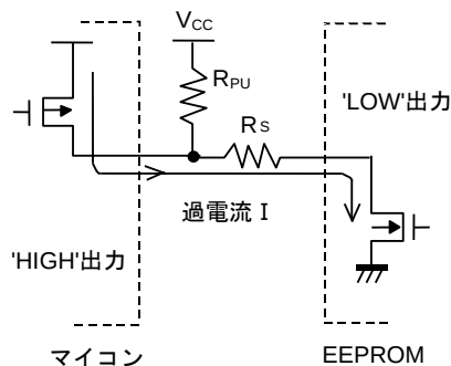
Figure 49. I/O 回路図
