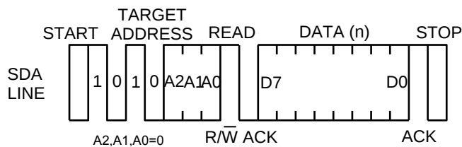
Figure 38. ランダムリード
