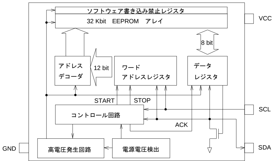
Figure 4. ブロック図
