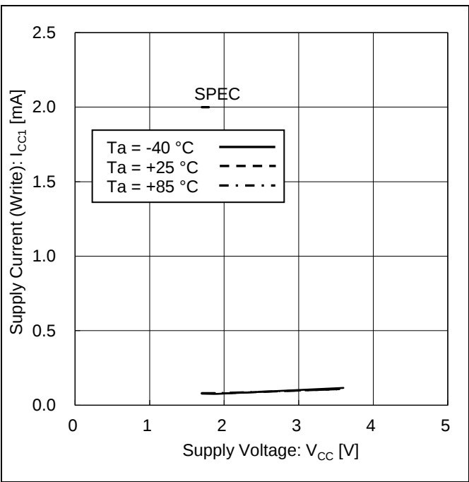
Figure 11. 消費電流 (ライト) vs 電源電圧 ( f_{SCL} = 400\text{ kHz} )
