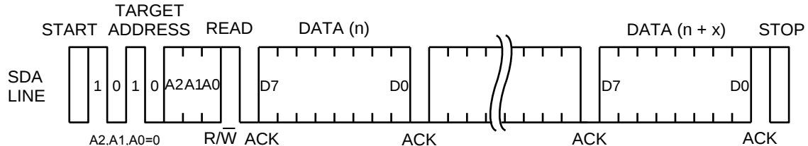
Figure 40. シーケンシャルリード (カレントリードの場合)
