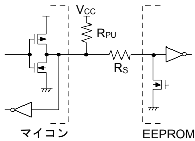
Figure 46. I/O 回路図
