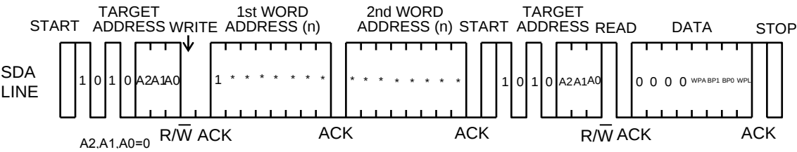
Figure 41-(b). ソフトウェアによる書き込み禁止レジスタのリードコマンド
