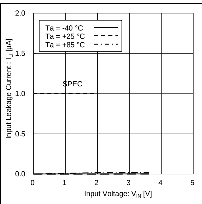
Figure 9. 入力リーク電流 vs 入力電圧
