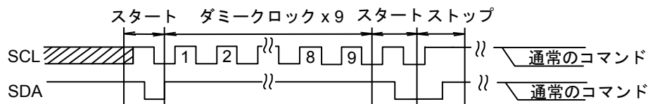
Figure 42. ソフトウェアリセット入力タイミング
