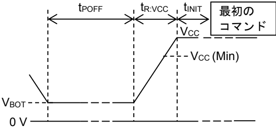
Figure 50. 電源立ち上げ波形図
