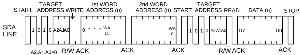
Figure 38. ランダムリード
