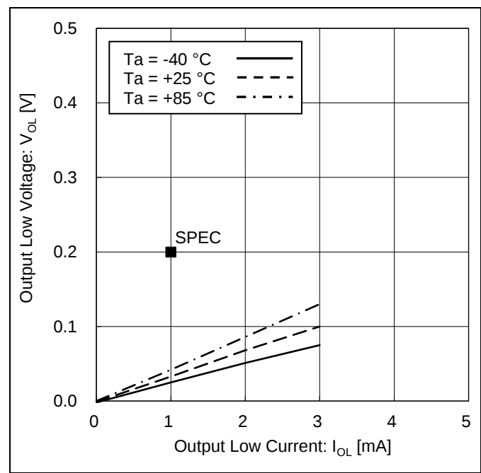
Figure 8. 'LOW'出力電圧 vs 'LOW'出力電流 (V CC = 1.7 V)
