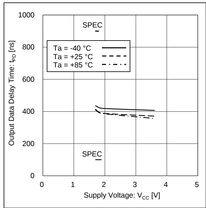
Figure 25. 出力データ遅延時間 vs 電源電圧 (SDA 'HIGH' to 'LOW')
