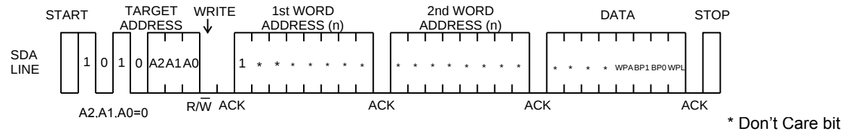
Figure 41-(a). ソフトウェアによる書き込み禁止レジスタのライトコマンド
