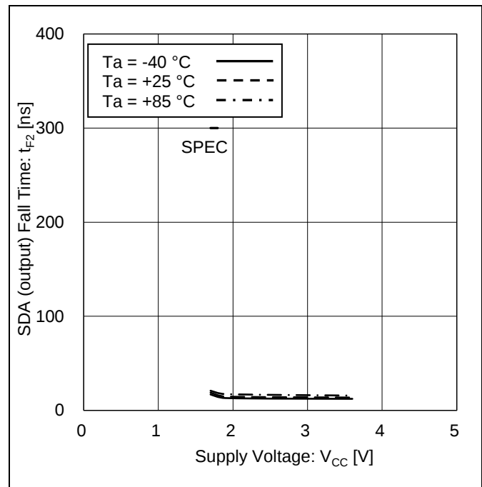
Figure 17. SDA の出力立ち下がり時間 vs 電源電圧
