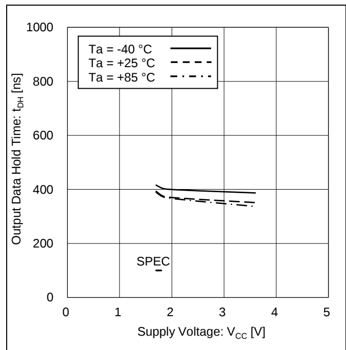
Figure 27. 出力データホールド時間 vs 電源電圧 (SDA 'HIGH' to 'LOW')
