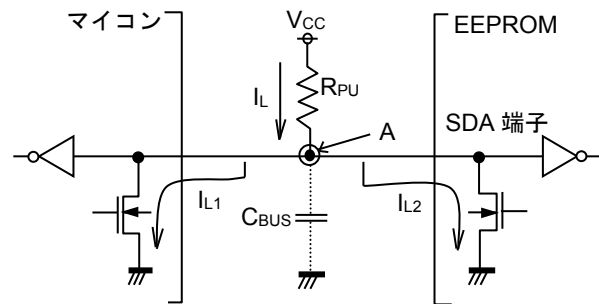
Figure 45. I/O 回路図
