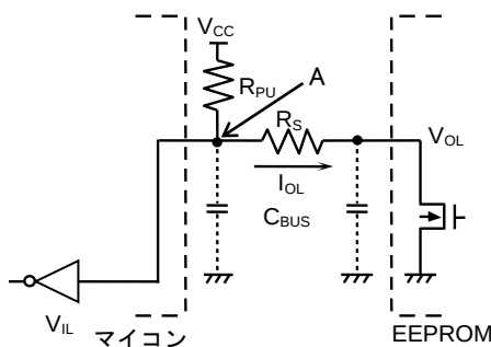
Figure 48. I/O 回路図
