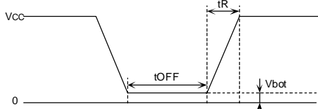
Figure 51. 立ち上がり波形図
