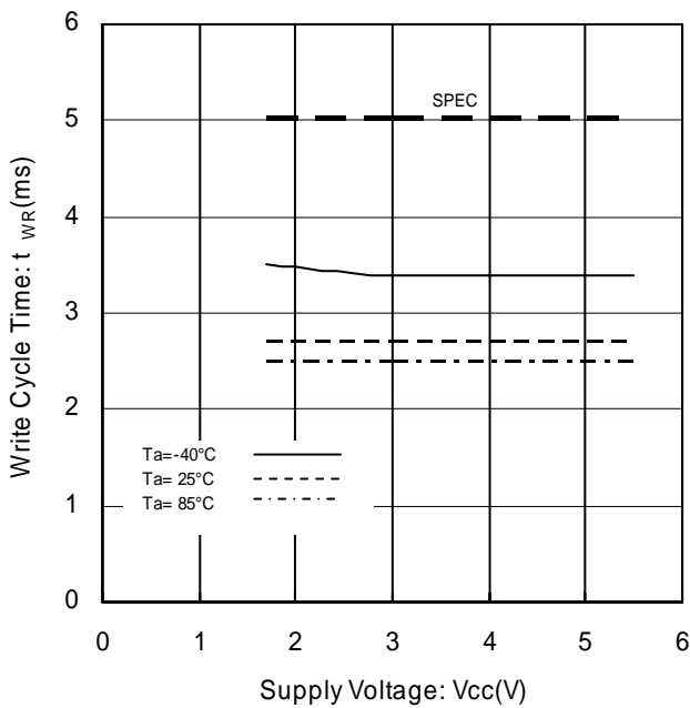
Figure 26. 内部書き込みサイクル時間 vs 電源電圧
