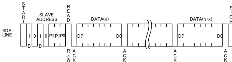
Figure 37. シーケンシャルリードサイクル (カレントリードサイクルの場合)
