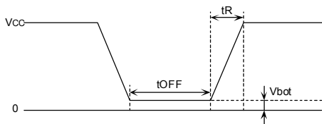
Figure 48. 立ち上がり波形図
