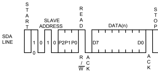
Figure 36. カレントリードサイクル
