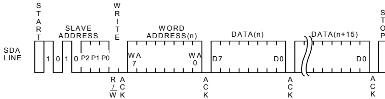
Figure 34. ページライトサイクル
