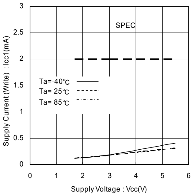
Figure 10. ライト動作時消費電流 vs 電源電圧 (f<sub>SCL</sub>=1MHz)
