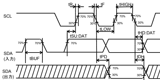
Figure 1-(a). 同期データ入出力タイミング
