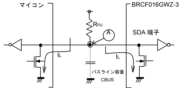
Figure 41. I/O 回路図
