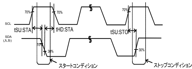
Figure 1-(b). スタート・ストップタイミング
