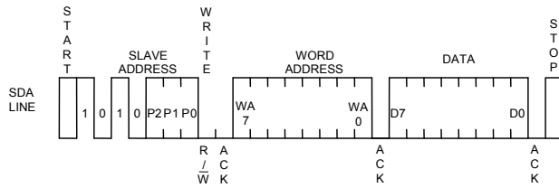
Figure 33. バイトライトサイクル
