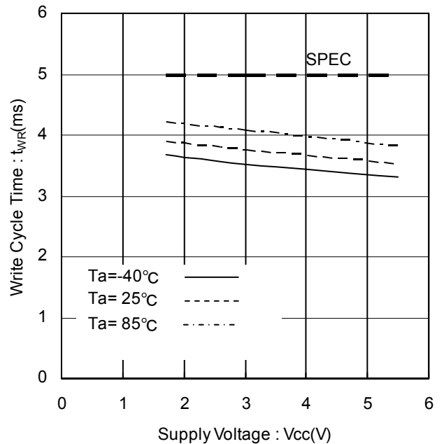
Figure 27. 内部書き込みサイクル時間 vs 電源電圧
