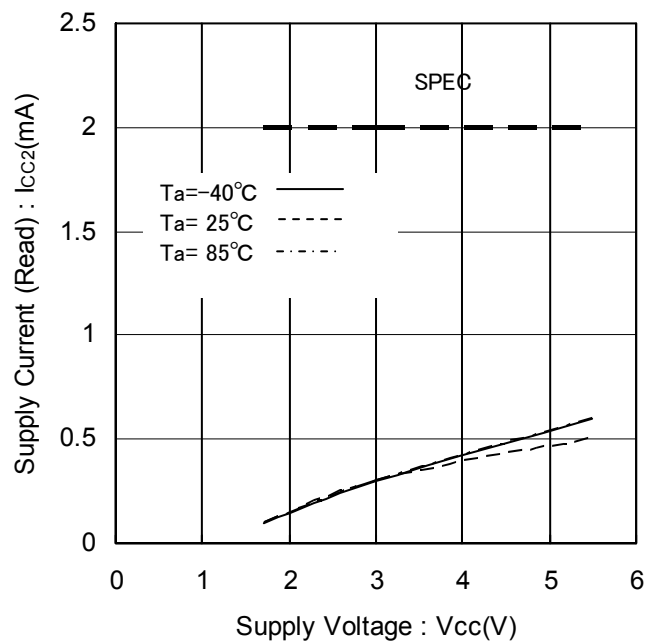
Figure 11. リード動作時消費電流 vs 電源電圧 (f<sub>SCL</sub>=1MHz)
