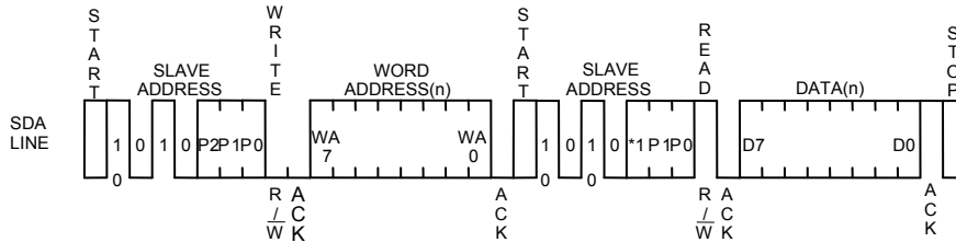
Figure 35. ランダムリードサイクル
