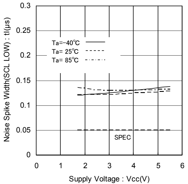
Figure 29. ノイズ除去有効時間 vs 電源電圧 (SCL L)
