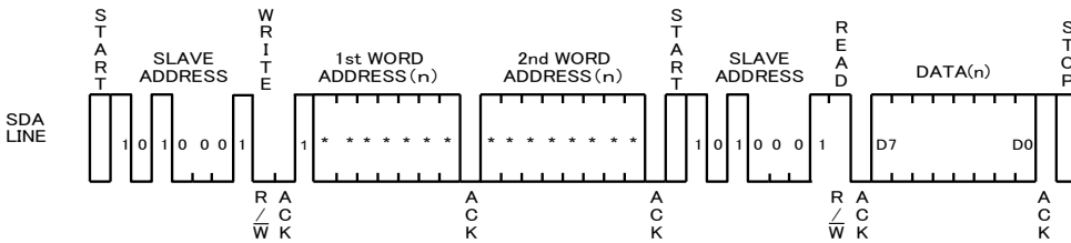
Figure 37. リード ライトプロテクトレジスタ サイクル
