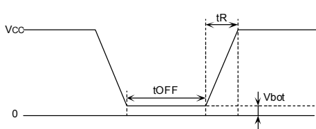
Figure 48. 立ち上がり波形図
