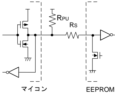
Figure 45. I/O 回路図
