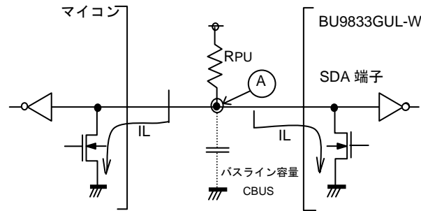
Figure 44. I/O 回路図
