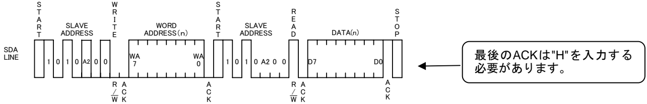
Figure 36. ランダムリードサイクル
