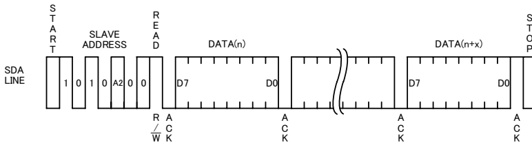
Figure 38. シーケンシャルリードサイクル
