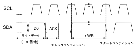
Figure 1(c) ライトサイクルタイミング
