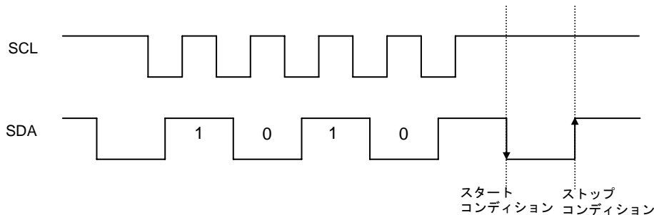
Figure 43. スレープアドレス入力中にスタート・ストップコンディションでキャンセルした場合
