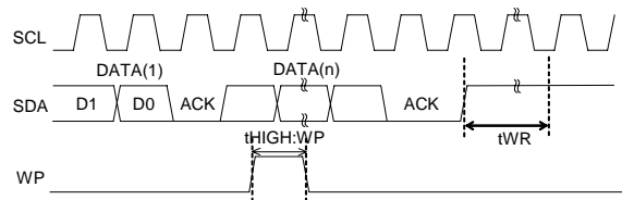
Figure 1(e) ライトキャンセル時 WP タイミング
