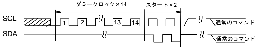
Figure 40 -(a) ダミークロック+START+START+コマンド入力の場合
