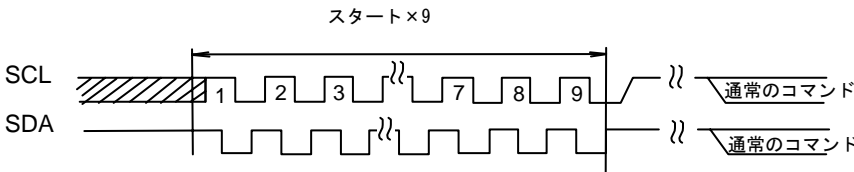
Figure 40-(c) START x 9+コマンド入力の場合
