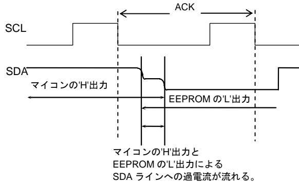
Figure 46. 入出力衝突タイミング
