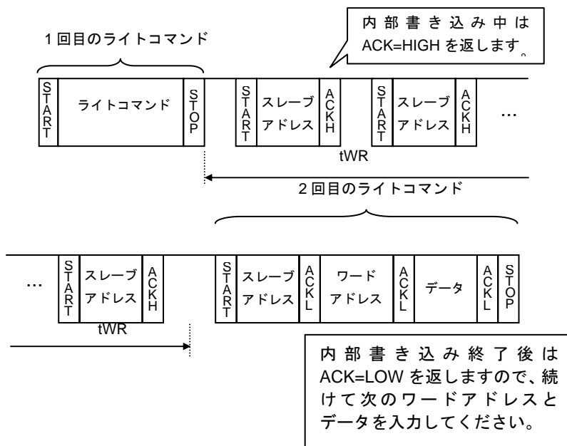
Figure 41. アクノリッジポーリングで連続して書き込みを行う場合
