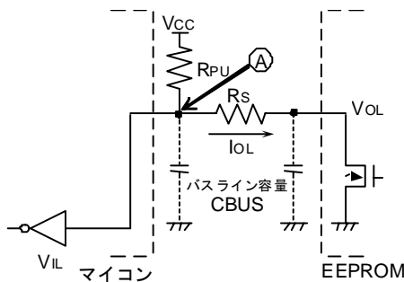
Figure 47. I/O 回路図
