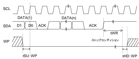
Figure 1-(d) ライト実行時 WP タイミング
