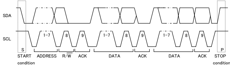
Figure 30. データ転送タイミング
