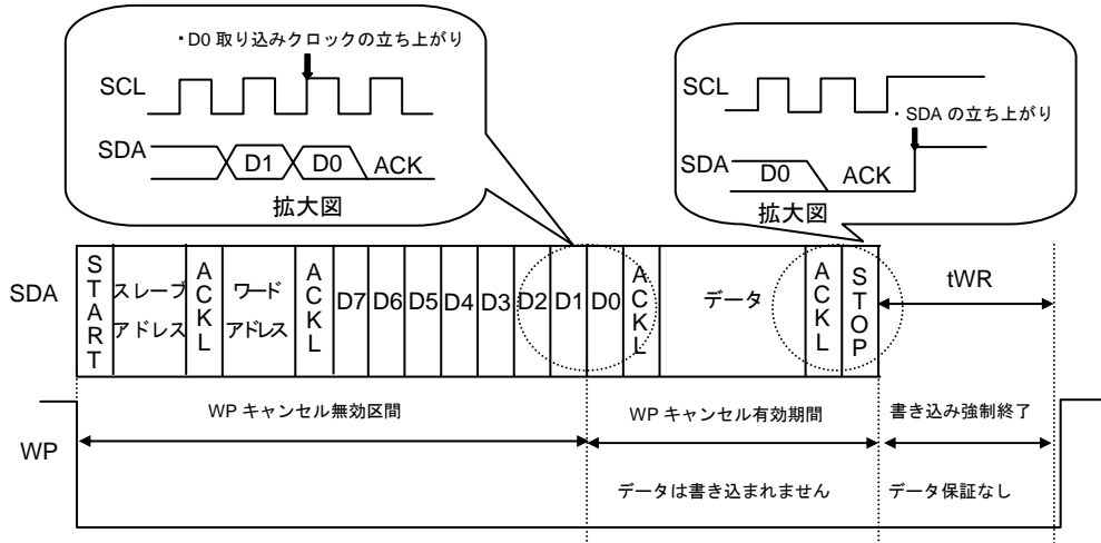
Figure 42. WP 有効タイミング
