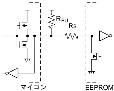
Figure 45. I/O 回路図
