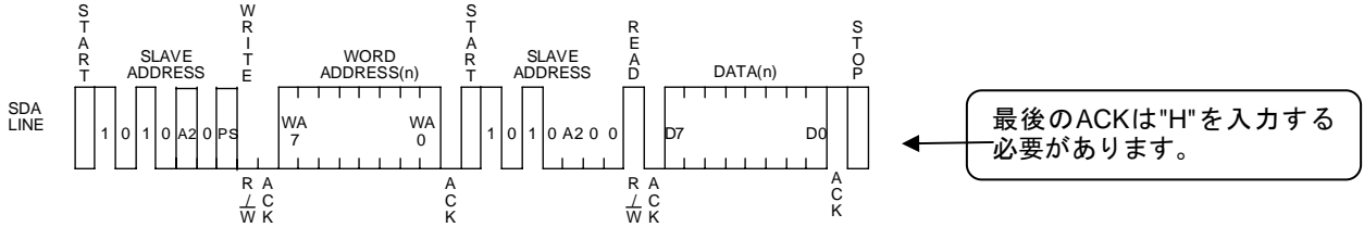
Figure 36. ランダムリードサイクル
