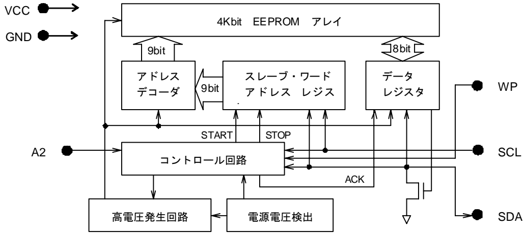
Fig.2 ブロック図
