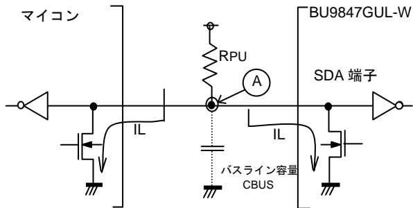
Figure 44. I/O 回路図
