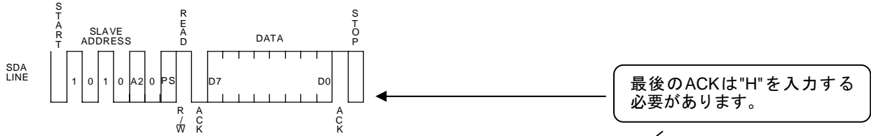
Figure 37. カレントリードサイクル
