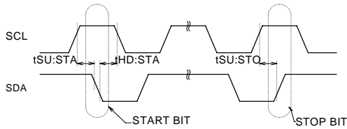
Figure 1-(b) スタート・ストップ
