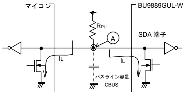
Figure 41. I/O 回路図
