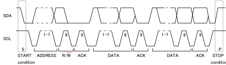
Figure 30. データ転送タイミング
