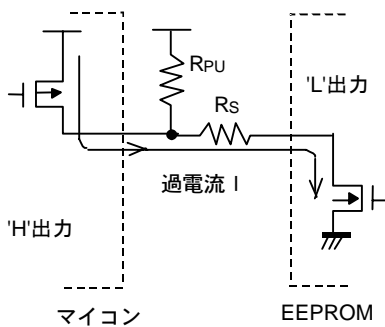
Figure 45. I/O 回路図
