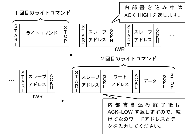
Figure 38. アクリッジポーリングで連続して書き込みを行う場合
