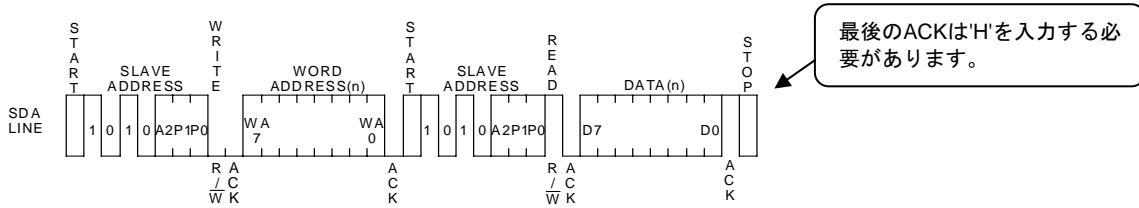
Figure 34. ランダムリードサイクル
