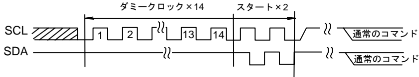
Figure 37-(a) 14 ダミークロック+START+START+コマンド入力の場合
