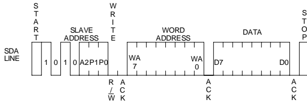
Figure 31. バイトライトサイクル
