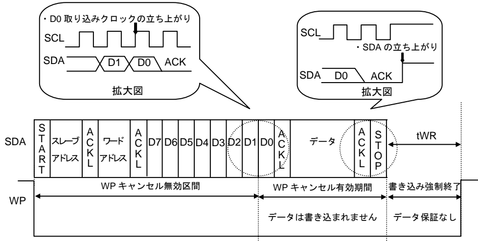
Figure 39. WP 有効タイミング
