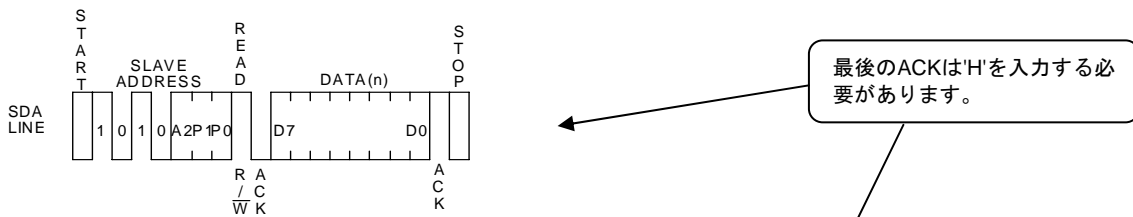
Figure 35. カレントリードサイクル
