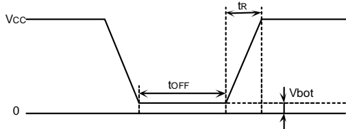
Figure 48. 立ち上がり波形図
