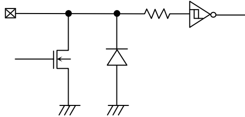
Figure 47. 入出力 pin 回路図
