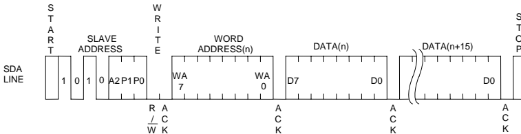
Figure 32. ページライトサイクル
