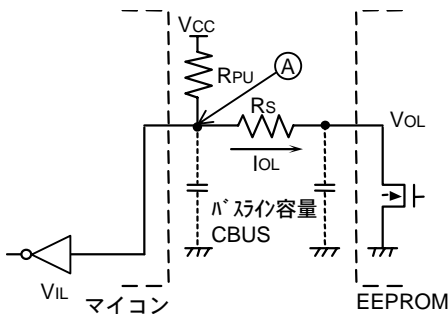
Figure 44. I/O 回路図
