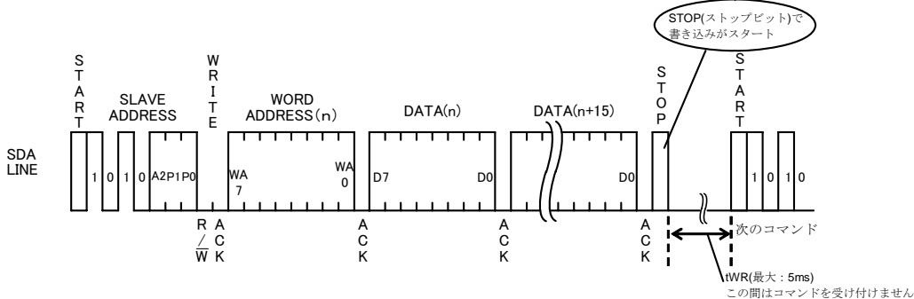
Figure 33. ページライトサイクル
