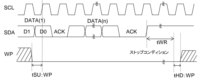
Figure 1-(d) ライト実行時 WP タイミング
