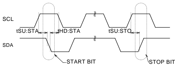
Figure 1-(a) 同期データ入出力タイミング
