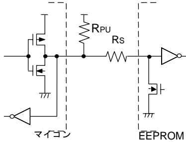
Figure 42. I/O 回路図
