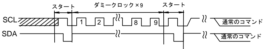
Figure 37-(b) START+9 ダミークロック+START+コマンド入力の場合
