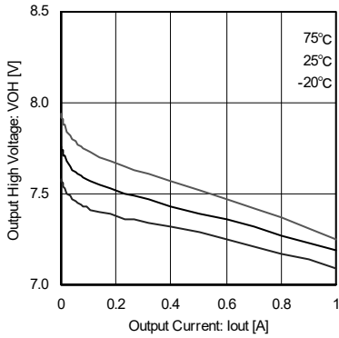
Fig.3 出力H電圧-出力電流 (BA6247FP-Y)
