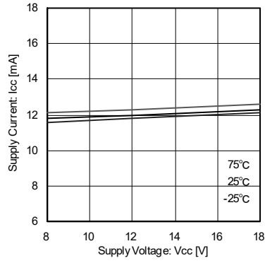
Fig.2 回路電流 (BA6238A)
