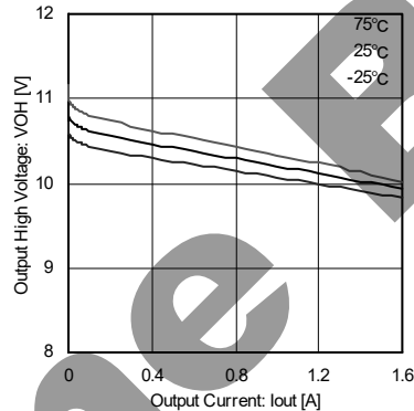
Fig.4 出力H電圧-出力電流 (BA6238A)
