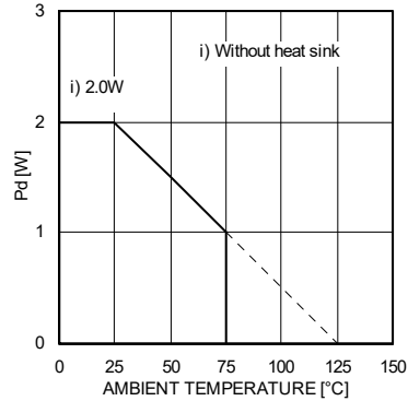
Fig.8 熱軽減曲線 (BA6238A, HSIP10)
