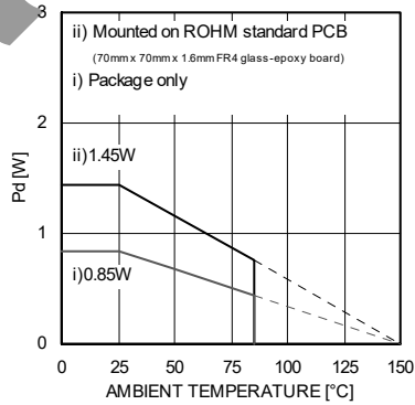
Fig.7 熱軽減曲線 (BA6247FP-Y, HSOP25)
