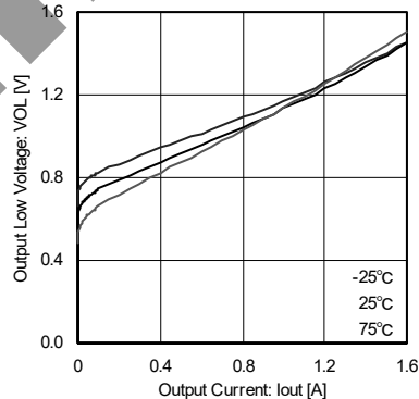
Fig.6 出力L電圧-出力電流 (BA6238A)
