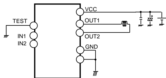
Figure 1. アプリケーション回路図
