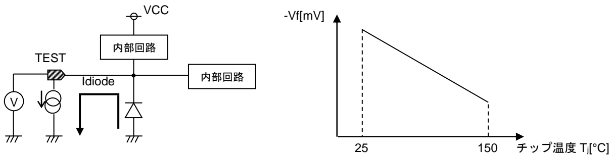
Figure 5. チップ温度測定の模式図
