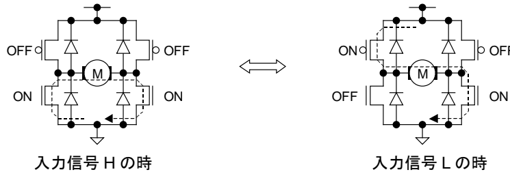
Figure 33. PWM 制御モード(出力)
