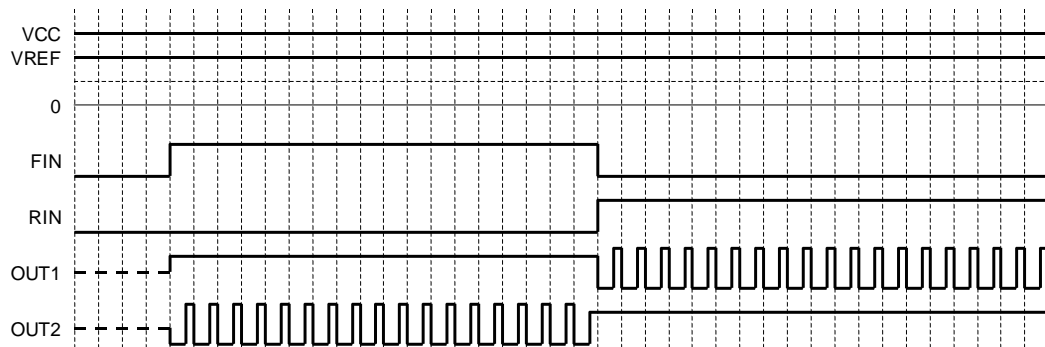
Figure 35. VREF 制御モード(タイミングチャート)
