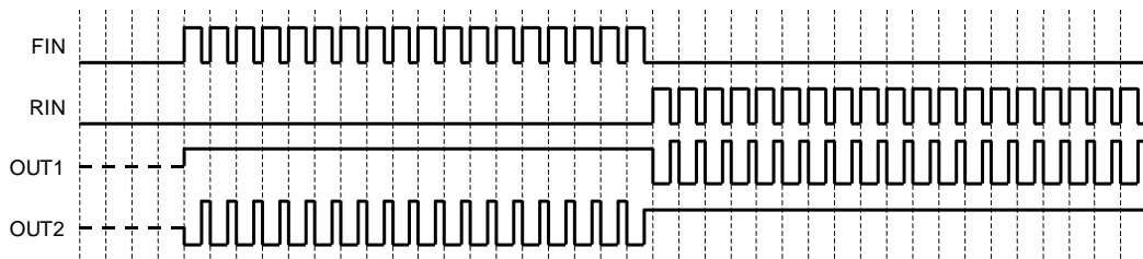
Figure 32. PWM 制御モード(タイミングチャート)
