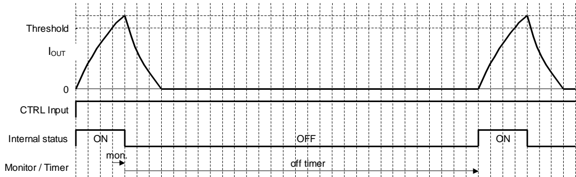
Figure 36. 過電流保護動作の例(タイミングチャート)
