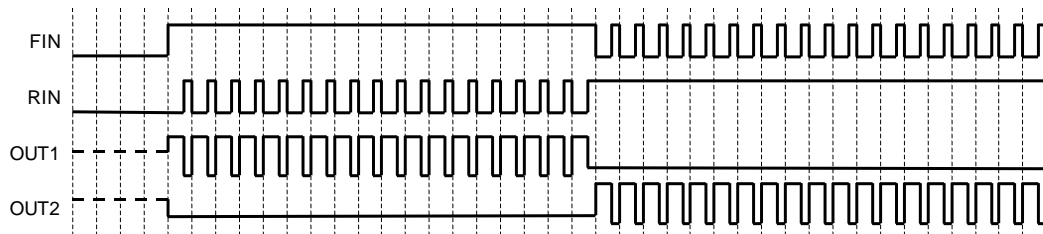
Figure 33. PWM 制御モード(出力)
