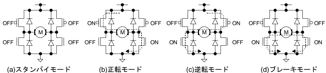
Figure 30. 基本動作モード(出力)
