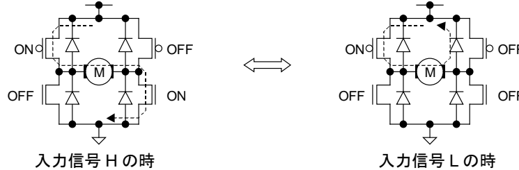
Figure 31. PWM 制御モード(出力)
