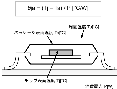
Fig.14 熱抵抗
