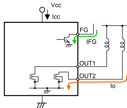
Fig.54 IC の消費電力の計算
