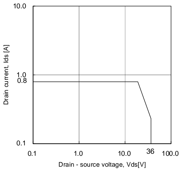
Fig.11 出力 Tr ASO ( T_{on}=100\text{msec} )
