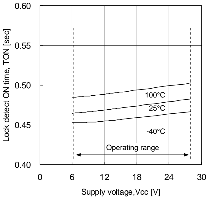
Fig.7 ロック検出 ON 時間
