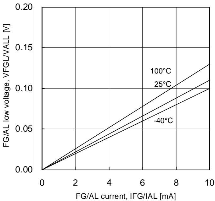
Fig.9 FG/AL 出力 L 電圧(温特)
