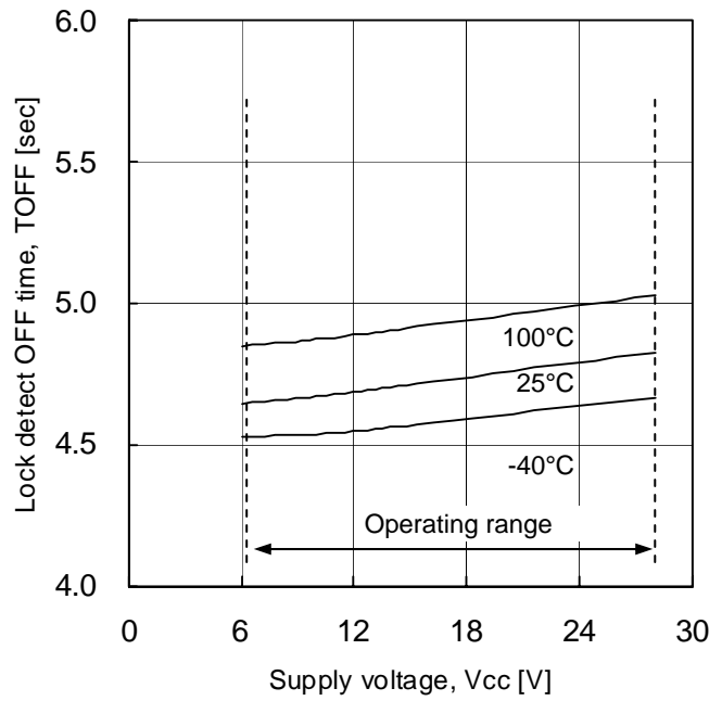
Fig.8 ロック検出 OFF 時間
