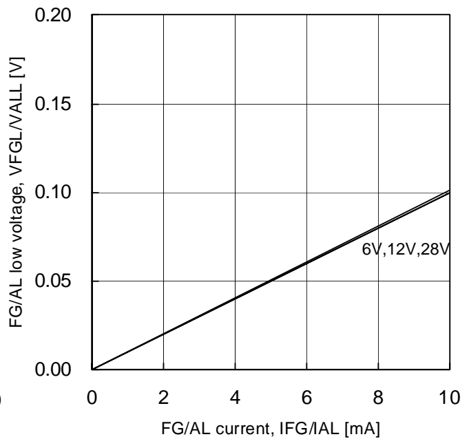
Fig. 10 FG/AL 出力 L 電圧(電特)
