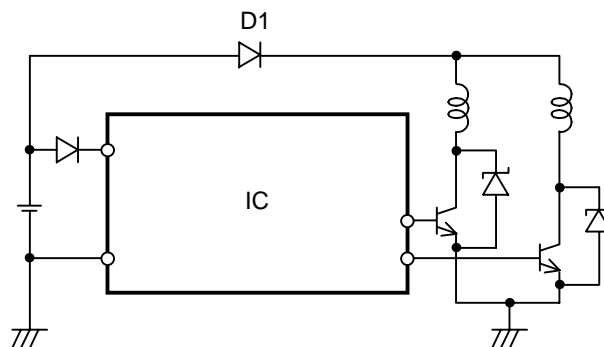
Fig.17 電源ラインの分離
