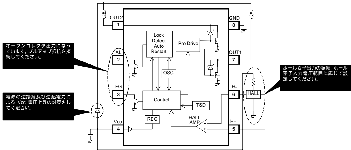
Fig.12 応用回路例
