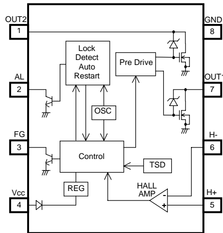
Fig. 2 ブロック図
