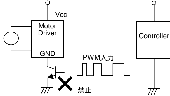
Fig.19 GND ライン PWM スイッチング禁止
