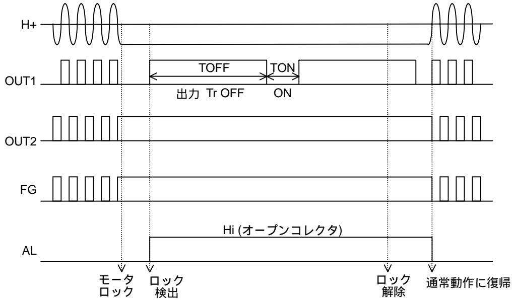
Fig.13 ロック保護(内蔵カウンタ方式)タイミングチャート
