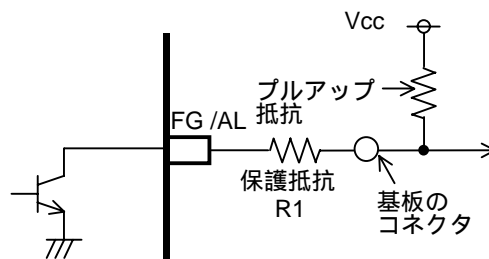
Fig.18 FG,AL 端子の保護
