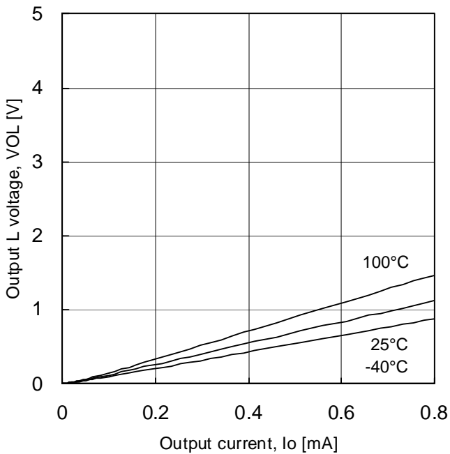
Fig.5 出力L電圧
