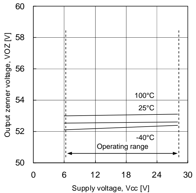
Fig.6 出力ツェナー電圧
