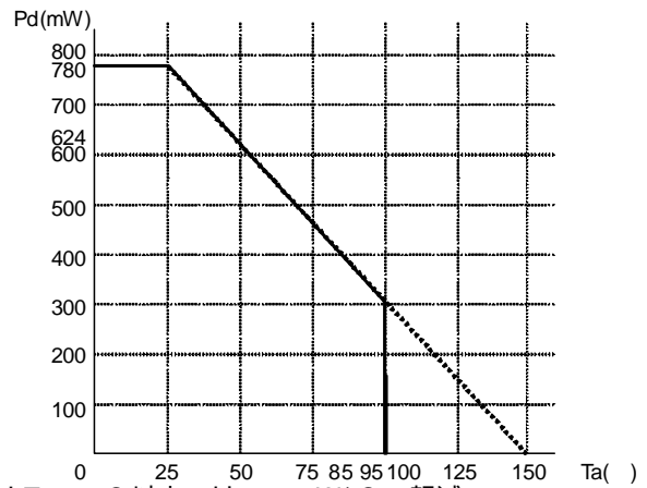
Fig.15 熱軽減曲線
