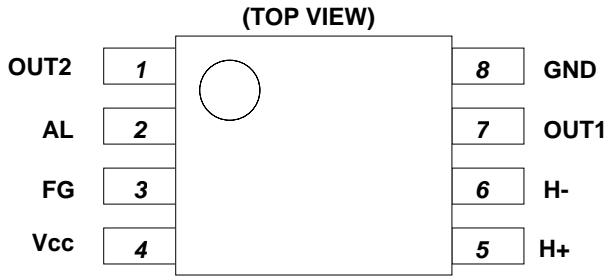
Fig.1 端子配置図
