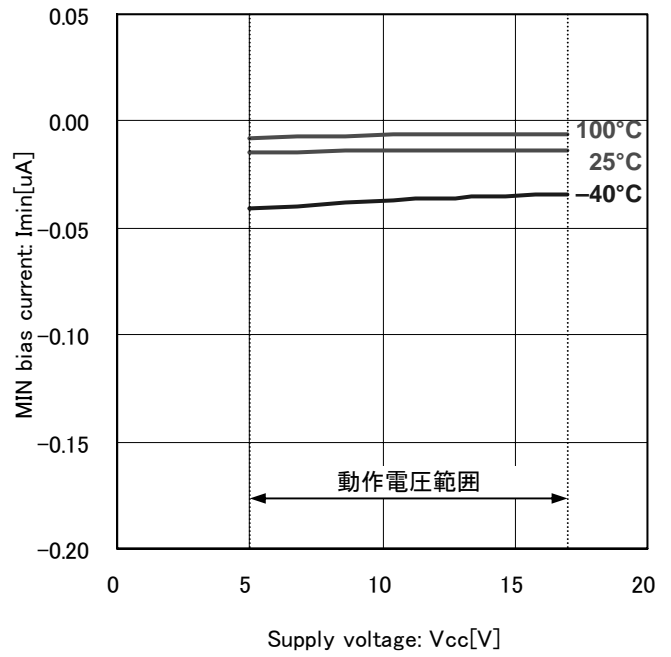
Fig.24 MIN バイアス電流
