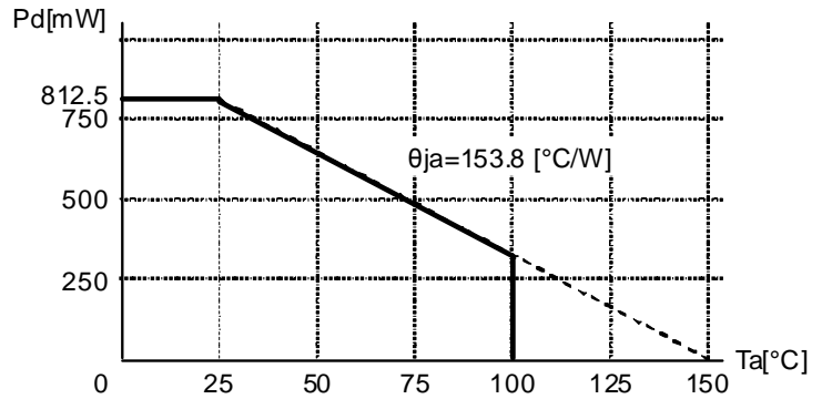
Fig.28 熱軽減曲線
