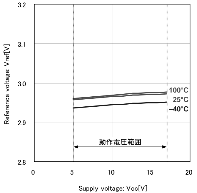
Fig.20 基準電圧
