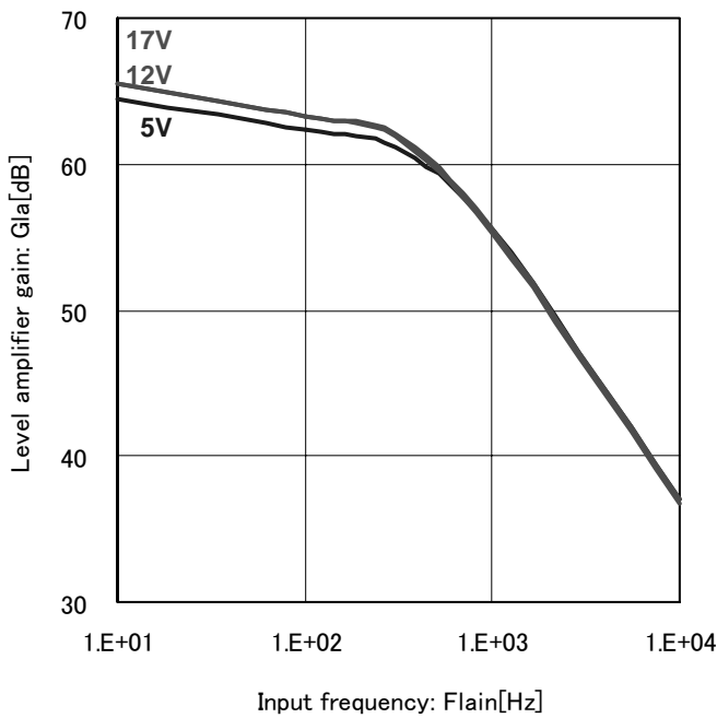
Fig.17 レベルアンプゲイン (Ta=25°C)
