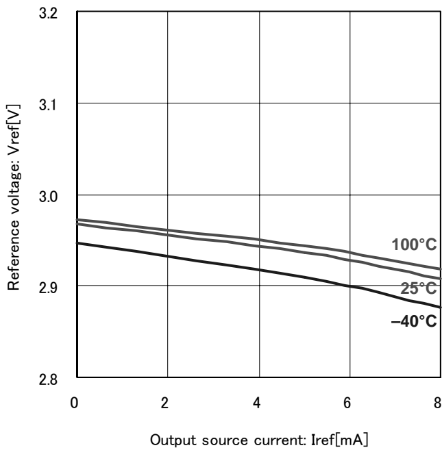
Fig.21 基準電圧電流能力 (Vcc=12V)
