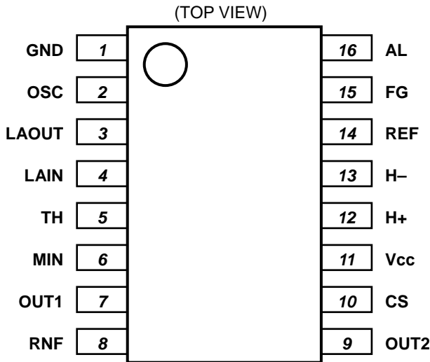
Fig.1 端子配置図
