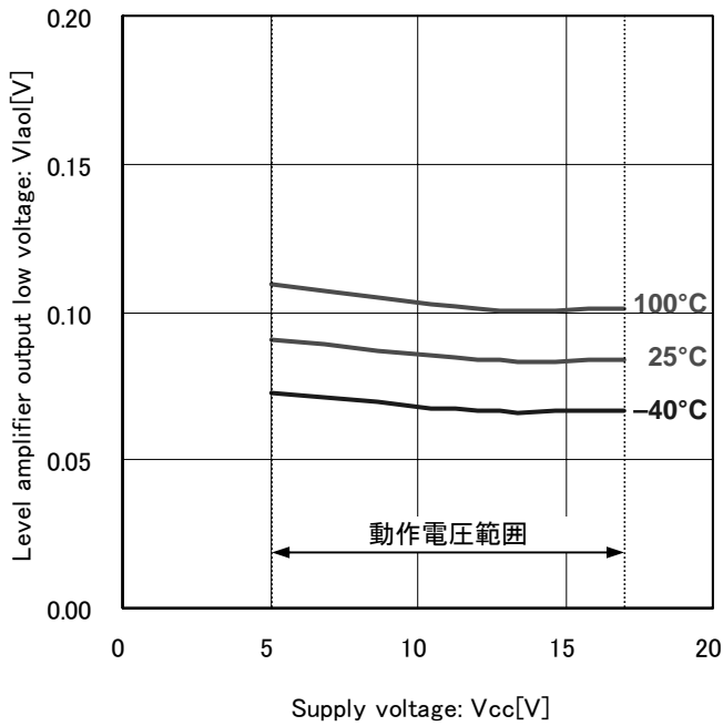
Fig.19 レベルアンプ出力 Low 電圧
