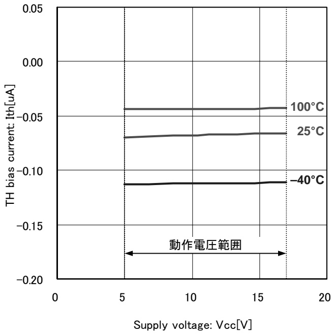
Fig.23 TH バイアス電流
