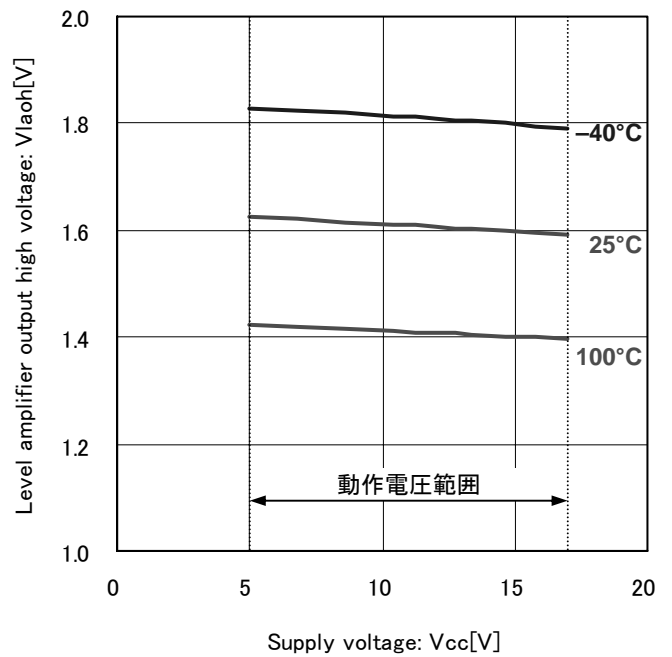
Fig.18 レベルアンプ出力 High 電圧
