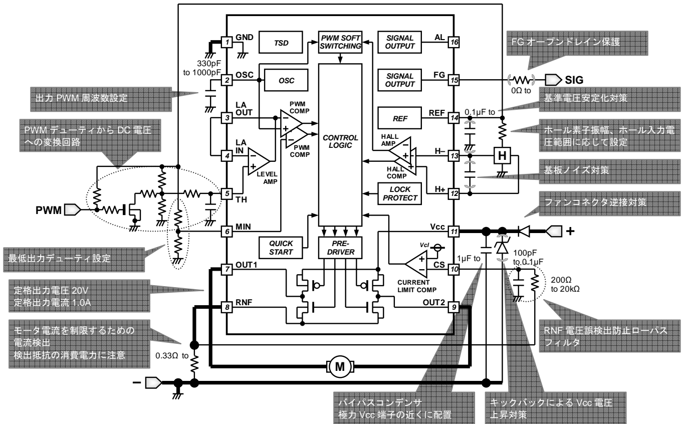
Fig.25 四線式(FG 出力)PWM 可変速モータ 応用回路例
