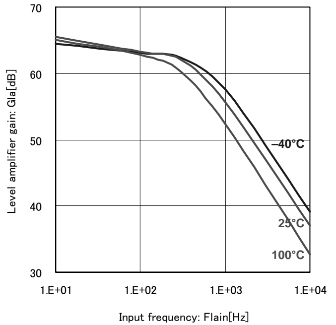
Fig.16 レベルアンプゲイン (Vcc=12V)
