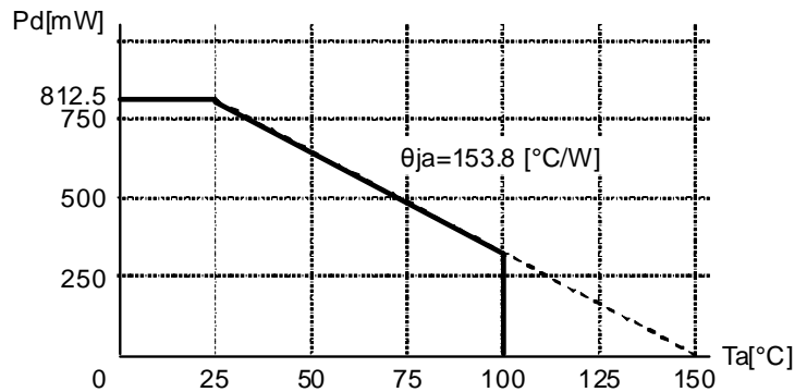
Fig.23 熱軽減曲線
