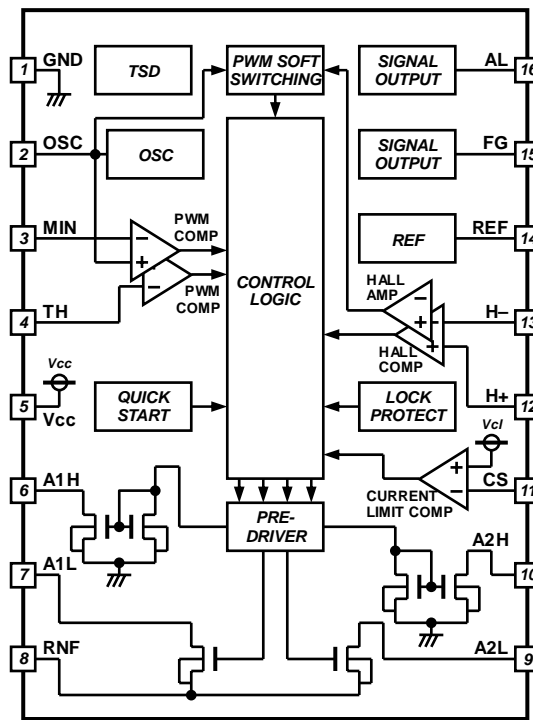
Fig.2 ブロック図
