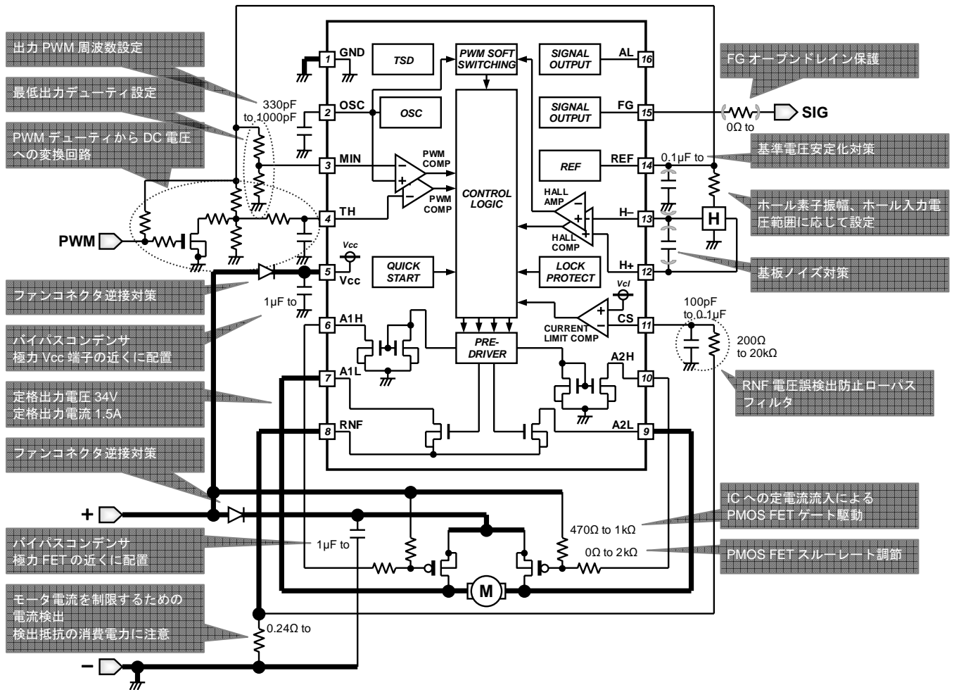
Fig.21 四線式(FG 出力)PWM 可変速モータ 応用回路例
