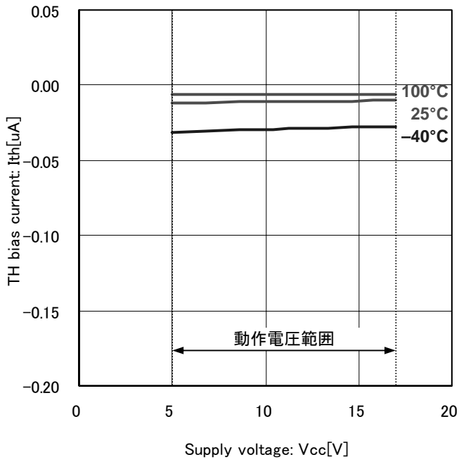
Fig.19 TH バイアス電流
