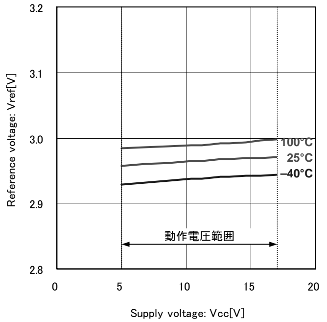
Fig.16 基準電圧
