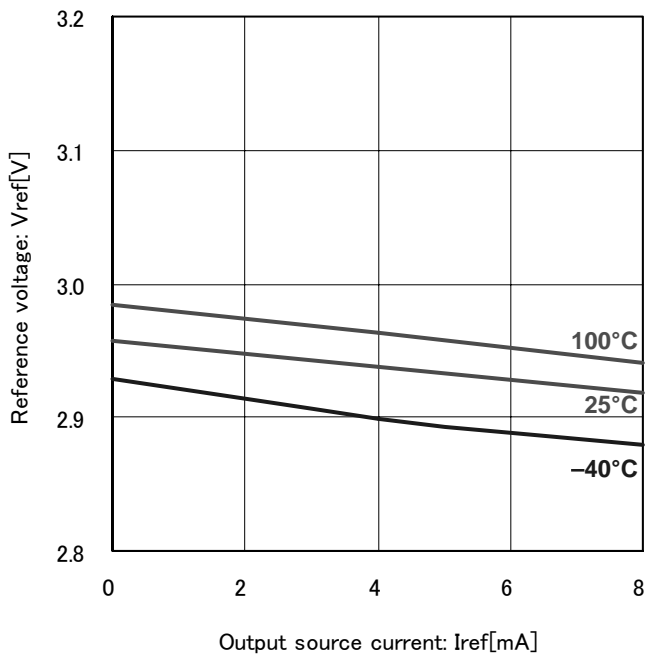
Fig.17 基準電圧電流能力 (Vcc=12V)
