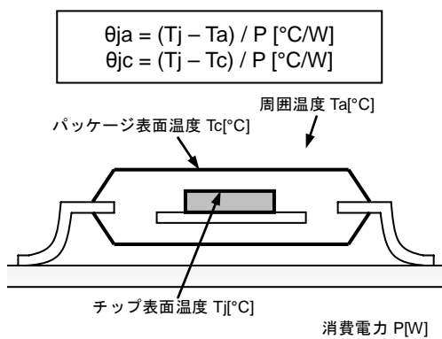
Fig.22 熱抵抗
