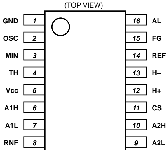
Fig.1 端子配置図
