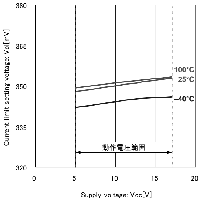
Fig.18 カレントリミット設定電圧
