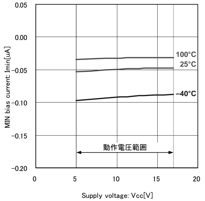
Fig.20 MIN バイアス電流
