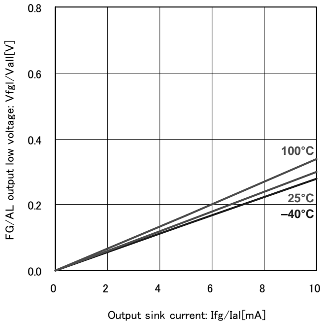
Fig.11 FG/AL 出力 Low 電圧 (Vcc=12V)
