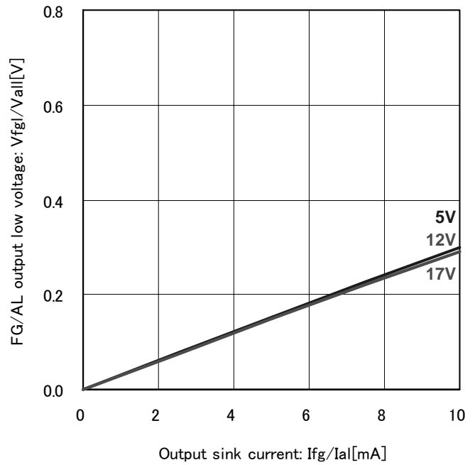
Fig.12 FG/AL 出力 Low 電圧 (Ta=25°C)
