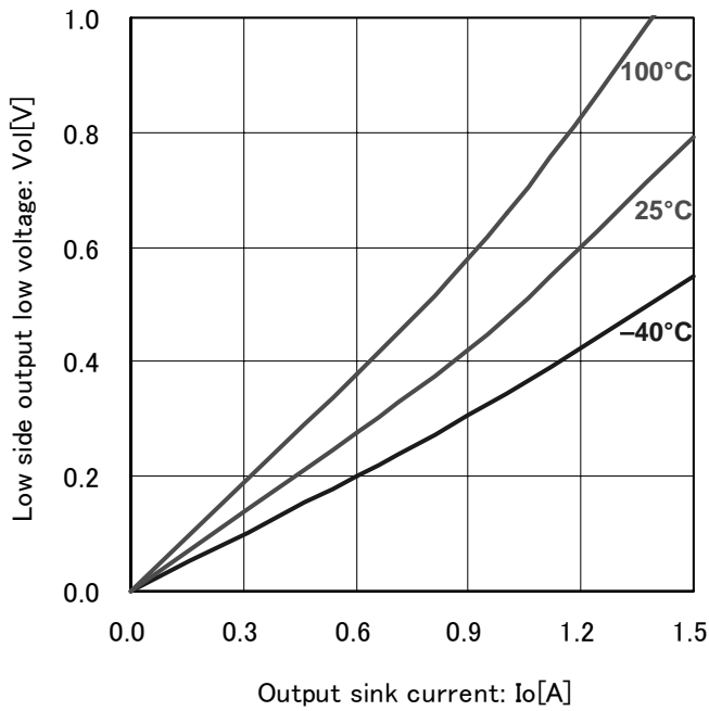
Fig.7 下側出力 Low 電圧 (V cc =12V)
