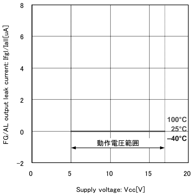
Fig.13 FG/AL 出力リーク電流
