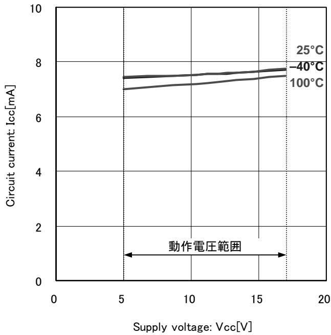
Fig.3 回路電流
