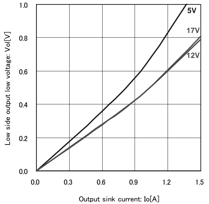
Fig.8 下側出力 Low 電圧 (T a =25°C)
