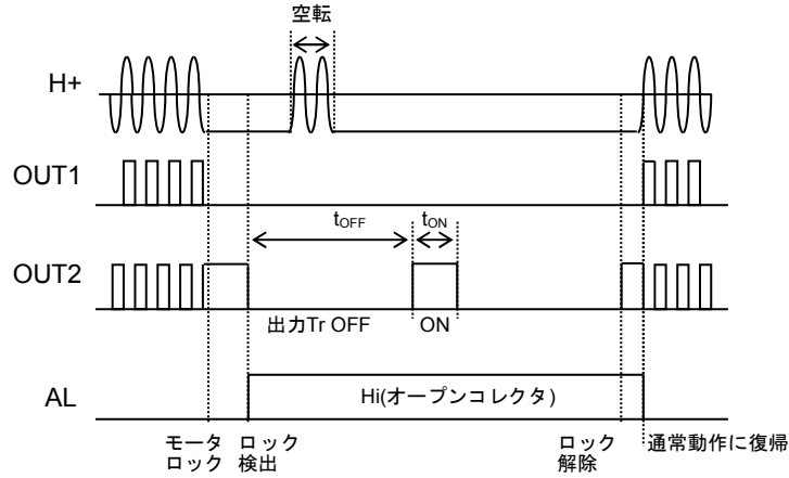
Figure 13. ロック保護タイミングチャート
