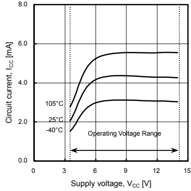
Figure 2. 回路電流 2
