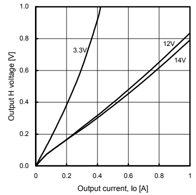
Figure 6. 出力 H 電圧 (電圧特性)
