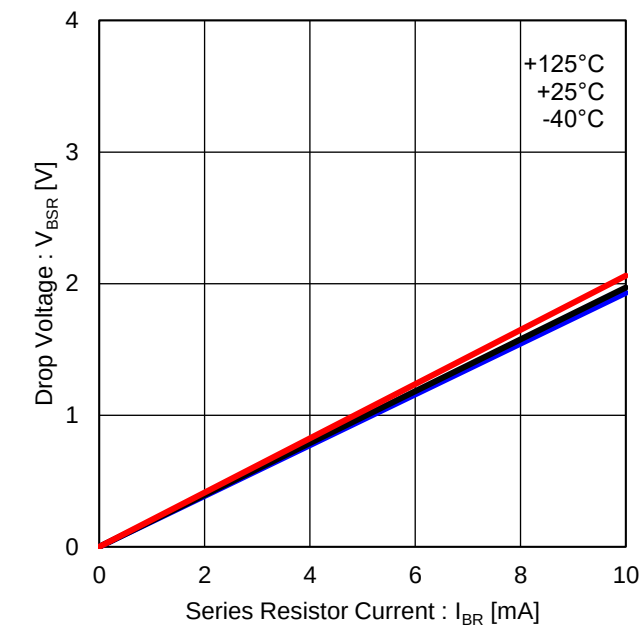
Figure 21. ブートダイオード直列抵抗特性
