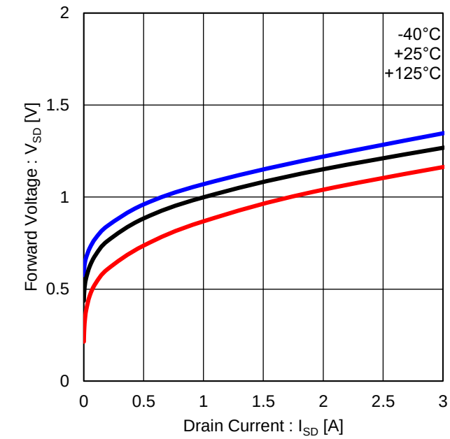
Figure 19. 出力ボディダイオード特性
