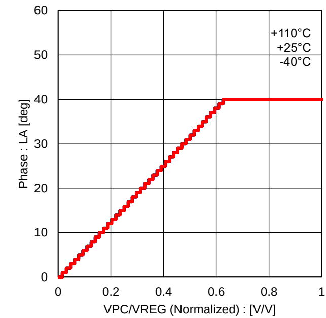
Figure 34. PC 電圧一位相角特性
