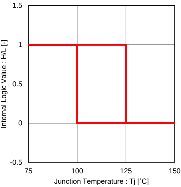
Figure 43. 過熱検出特性
