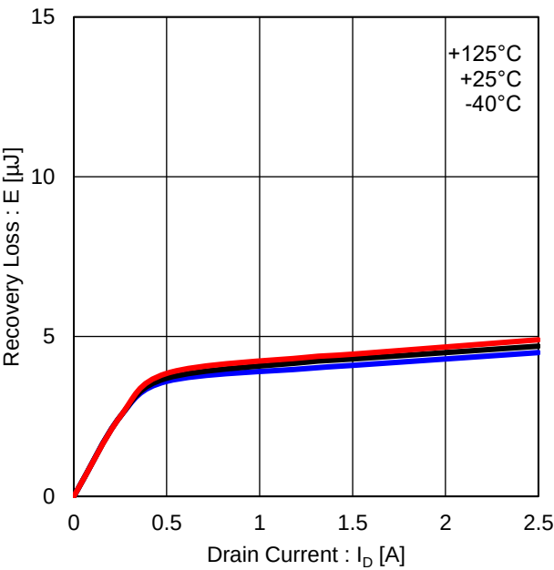
Figure 23. 上側リカバリー・ロス (VDC=300V)
