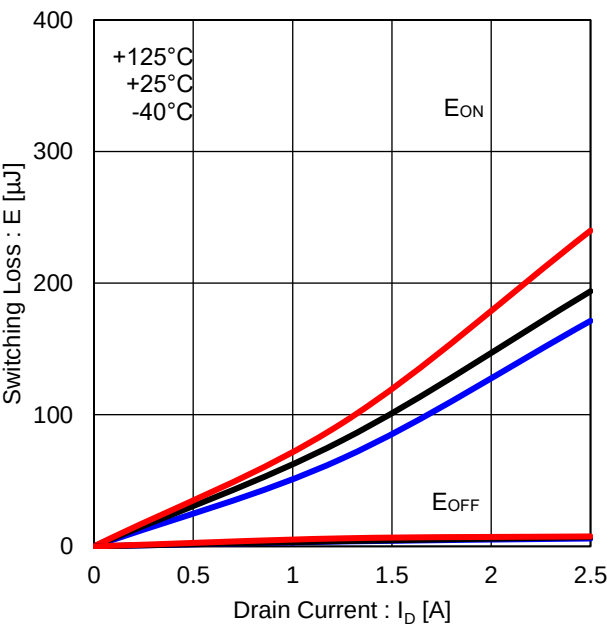
Figure 24. 下側スイッチング・ロス (VDC=300V)
