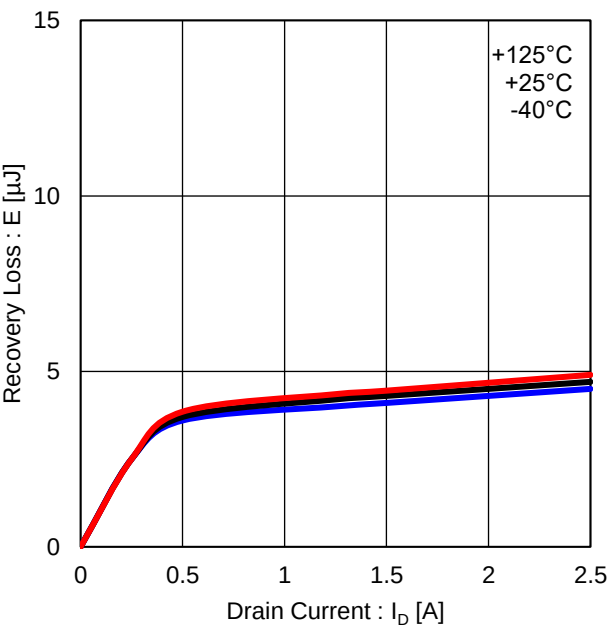
Figure 25. 下側リカバリー・ロス (VDC=300V)
