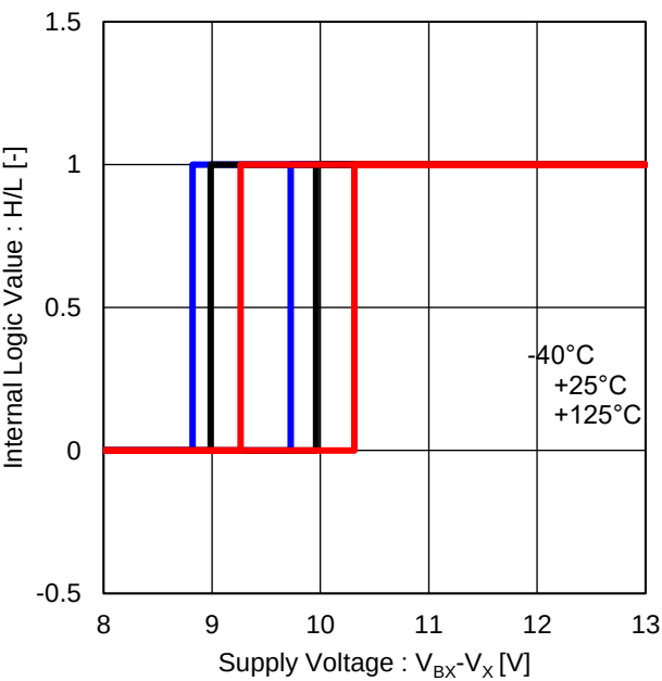
Figure 44. 上側 UVLO 特性
