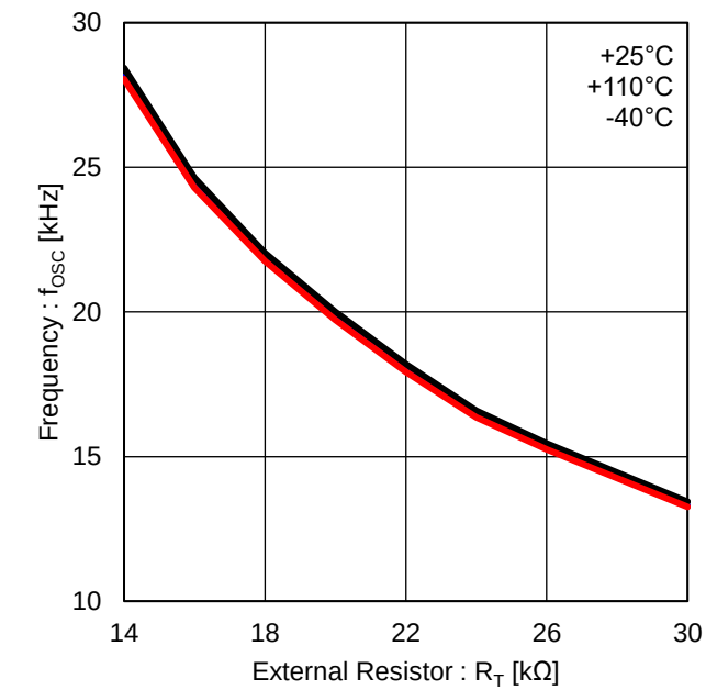
Figure 35. 発振周波数－RT 特性
