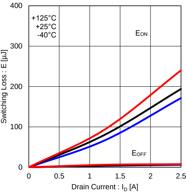
Figure 22. 上側スイッチング・ロス (VDC=300V)
